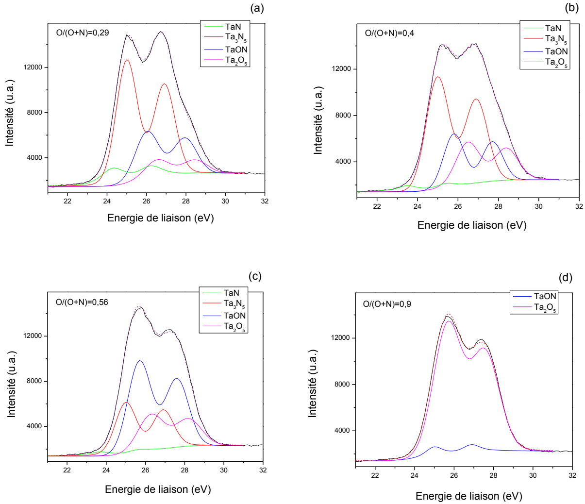
Figure 72. Spectre XPS du niveau Ta4f de couches minces de \text{TaO}_x\text{N}_y de compositions variables.
