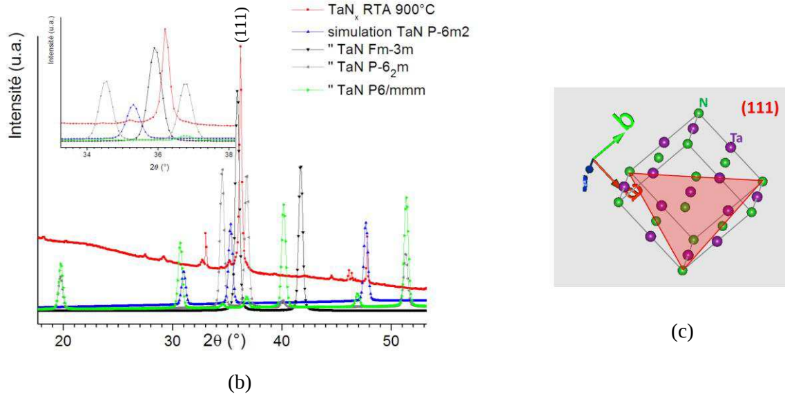
Figure 82. Diagramme DRX de la phase \text{TaN}_x RTA 900°C comparé (a) : au diagramme X de la phase \text{TaN}_x avant recuit et à celui du substrat Si ; (b) : aux diagrammes simulés des phases TaN rapportés dans la littérature. (c) visualisation des plans (111) de la structure TaN cubique à faces centrées (Fm-3m).
