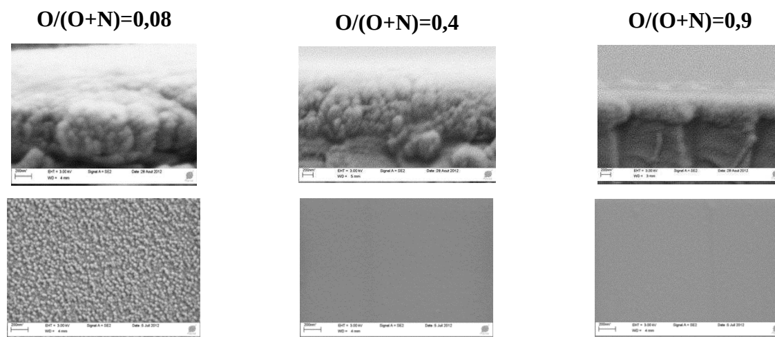
Figure 58. Images MEB de la surface des couches minces \text{TaO}_x\text{N}_y déposées pour différents rapports \text{O}/(\text{O}+\text{N}) .
