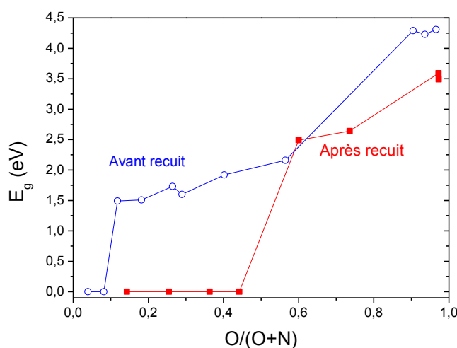
Figure 110. Gap optique obtenu à partir des mesures ellipsométriques des couches minces de \text{TaO}_x\text{N}_y avant et après recuit dans un four RTA à 900^\circ\text{C}
