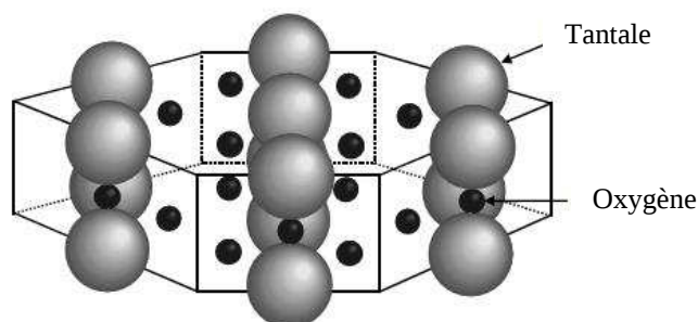
Figure 15. Structure de l'oxyde de tantale en phase hexagonale [26].
