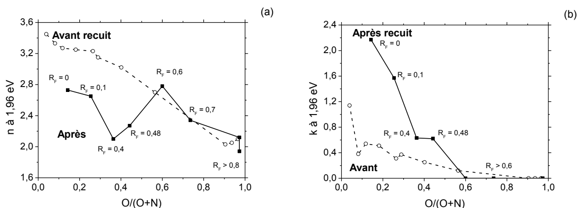
Figure 109. (a) Indice de réfraction et (b) coefficient d'extinction des couches minces TaO_xN_y à 1,96 eV avant et après recuit.
