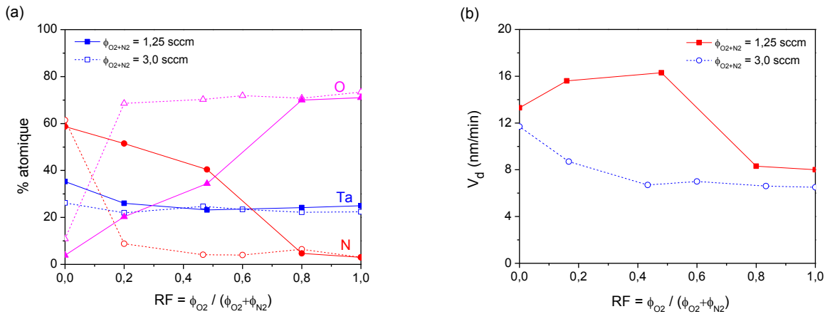
Figure 54. (a) composition élémentaire et (b) vitesse de dépôt des films déposés à R_F croissant à pour \Phi_{O_2+N_2} = 1,25 (plain) et 3,0 sccm (ouvert).
