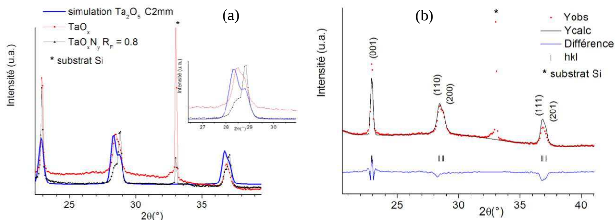
Figure 91. (a) comparaison du diagramme observé pour \text{TaO}_x avec le diagramme de la phase \text{TaO}_x\text{N}_y R_F = 1 et celui simulé de la phase \text{Ta}_2\text{O}_5 (C2mm) (b) résultats de l'affinement du diagramme X par la méthode de Rietveld en considérant la phase \text{Ta}_2\text{O}_5 (C2mm) (Yobs : données expérimentales ; Ycalc : diagramme calculé ; Différence : Yobs-Ycalc ; hkl : indices de Miller des plans atomiques qui diffractent).
