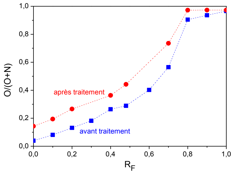
Figure 80. Rapport de composition des couches minces de TaO_xN_y en oxygène et azote en fonction de R_F pour les couches avant et après traitement thermique à 900°C sous azote.
