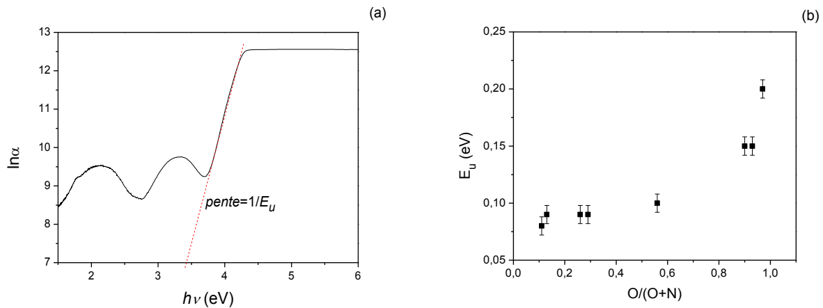
Figure 98 (a) Détermination de l'énergie d'Urbach et (b) valeurs de l'énergie d'Urbach pour les couches minces de \text{TaO}_x\text{N}_y de compositions différentes.
