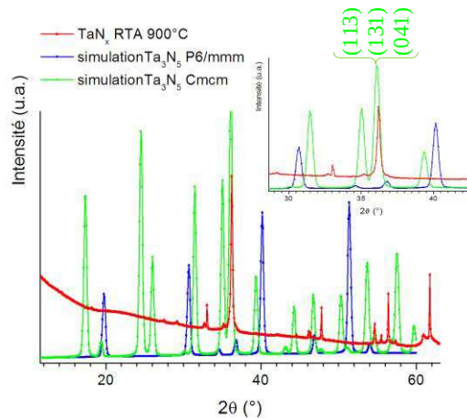
Figure 83. Diagramme X de la phase \text{TaN}_x RTA 900°C comparée aux diagrammes simulés des phases \text{Ta}_3\text{N}_5 rapportés dans la littérature.
