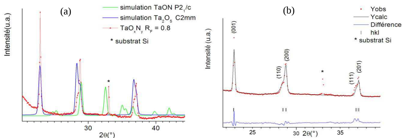
Figure 89. (a) comparaison du diagramme observé pour \text{TaO}_x\text{N}_y R_F = 0,8 avec les diagrammes simulés des phases \text{Ta}_2\text{O}_5 ( C2mm ) et \text{TaON} ( P2_1/c ) (b) résultats de l'affinement du diagramme X par la méthode de Rietveld en considérant la phase \text{Ta}_2\text{O}_5 ( C2mm ) (Yobs : données expérimentales ; Ycalc : diagramme calculé ; Différence : Yobs-Ycalc ; hkl : indices de Miller des plans atomiques qui diffractent).
