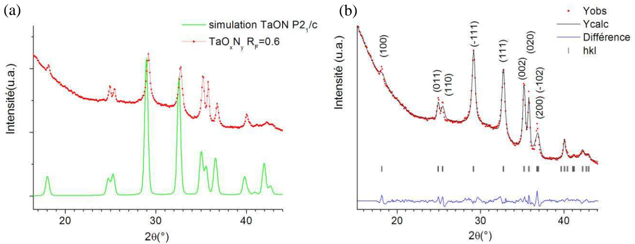
Figure 86. (a) comparaison du diagramme observé pour TaO x N y R F = 0,6 avec le diagramme simulé de la phase TaON (P21/c) (b) résultats de l’affinement du diagramme X par la méthode de Rietveld en considérant la phase TaON (P21/c) (Yobs : données expérimentales ; Ycalc : diagramme calculé ; Différence : Yobs-Ycalc ; hkl : indices de Miller des plans atomiques qui diffractent).
