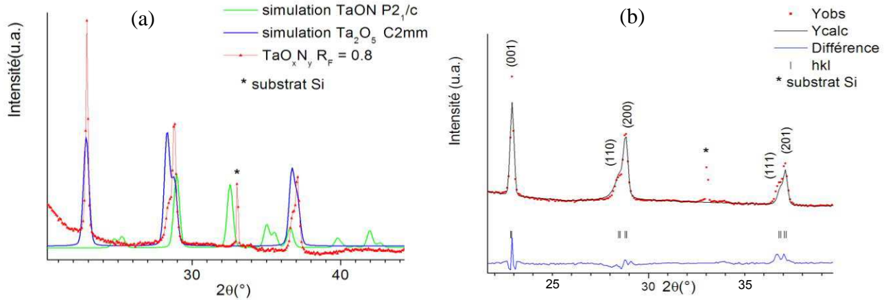
Figure 89. (a) comparaison du diagramme observé pour TaO_xN_y R_F = 0,8 avec les diagrammes simulés des phases Ta_2O_5 (C2mm) et TaON ( P2_1/c ) (b) résultats de l’affinement du diagramme X par la méthode de Rietveld en considérant la phase Ta_2O_5 (C2mm) (Yobs : données expérimentales ; Ycalc : diagramme calculé ; Différence : Yobs-Ycalc ; hkl : indices de Miller des plans atomiques qui diffractent).
