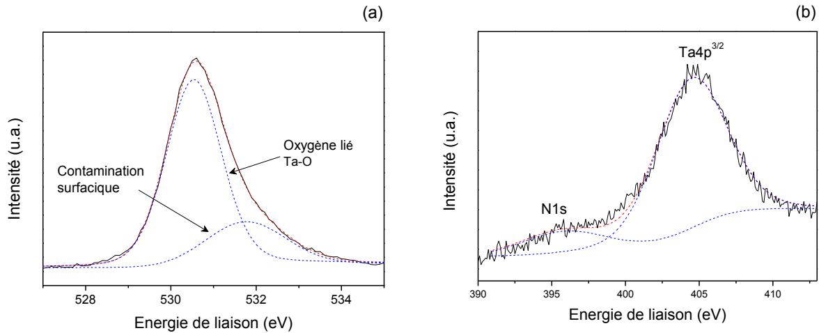
Figure 75. (a) Spectre XPS du niveau \text{O}1s et (b) celui du niveau \text{N}1s et \text{Ta}4p^{3/2} d'une couche mince de \text{TaO}_x ( R_F=1 ).
