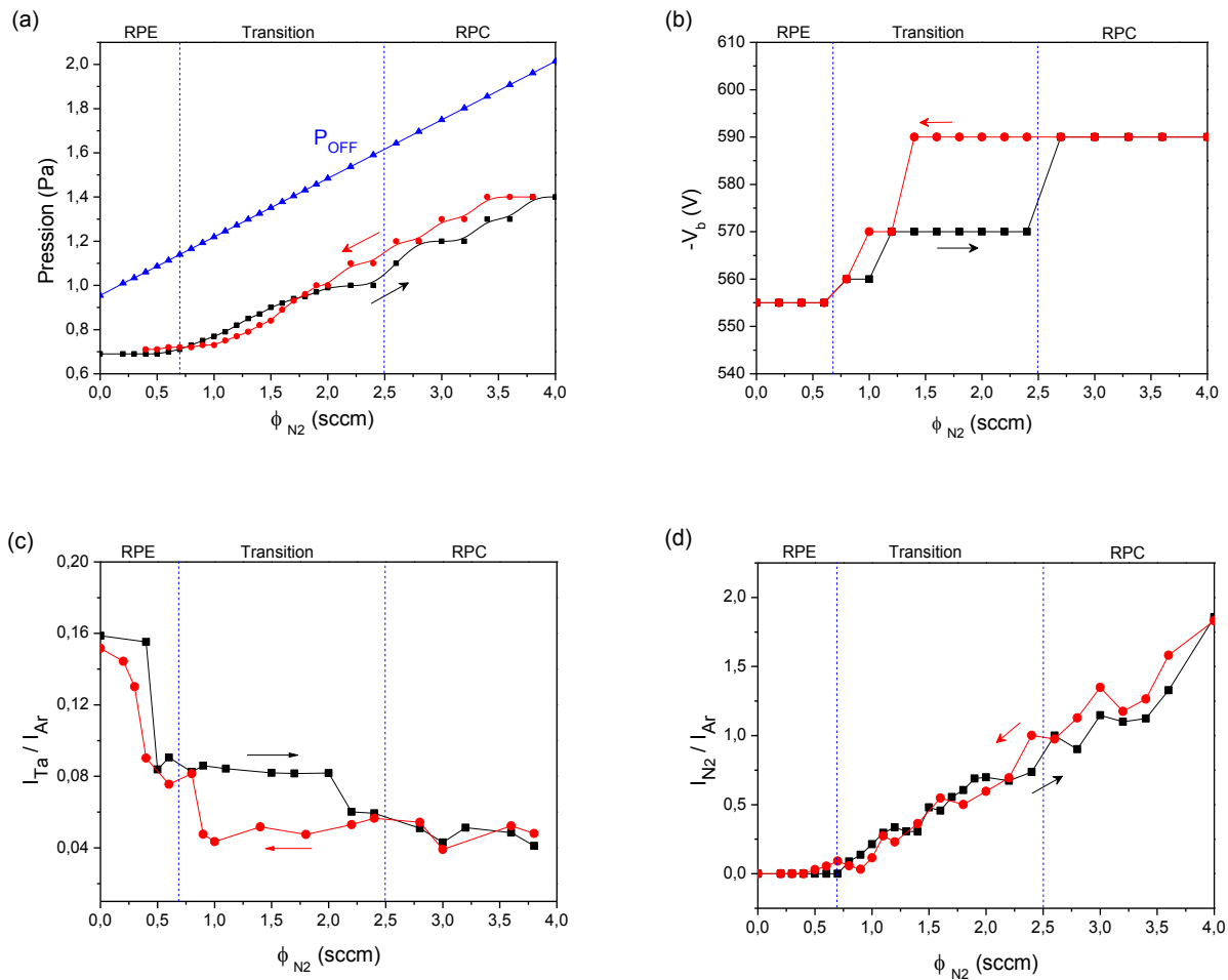
Figure 46. (a) Pression sans plasma ( P_{OFF} ) et avec plasma, (b) Tension d'autopolarisation de la cible, (c) I_{Ta}/I_{Ar} , (d) I_N/I_{Ar} pour un mélange Ar/N 2 .
