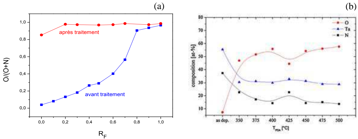
Figure 79. (a) Rapport de composition des couches minces de TaO_xN_y en oxygène et azote en fonction de R_F pour les couches avant et après traitement thermique à 900^\circ\text{C} sous air et (b) L'incorporation de l'oxygène dans les couches de nitrure de tantale en fonction de la température de recuit sous air ambiant obtenu par Grosser et al. [98].
