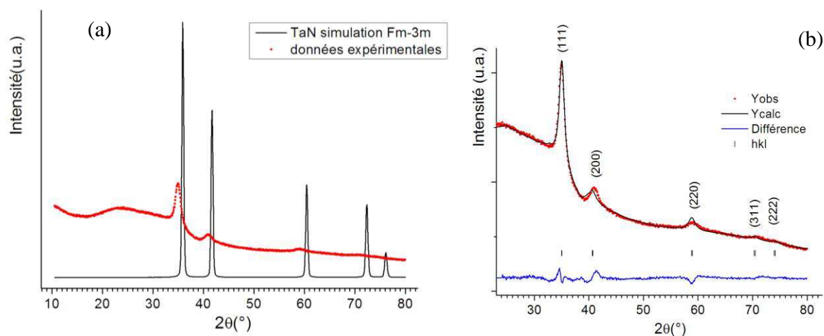
Figure 63. Analyse par diffraction des rayons X du dépôt obtenu dans un plasma d'argon/azote « TaO 0,07 N 1,85 » : (a) comparaison avec le diagramme simulé de TaN cristallisant dans une maille cubique (groupe d'espace Fm-3m) ; (b) résultat de l'affinement par la méthode de Le Bail ( Yobs : données expérimentales ; Ycalc : diagramme calculé ; Différence : Yobs-Ycalc ; hkl : indices de Miller des plans atomiques qui diffractent).
