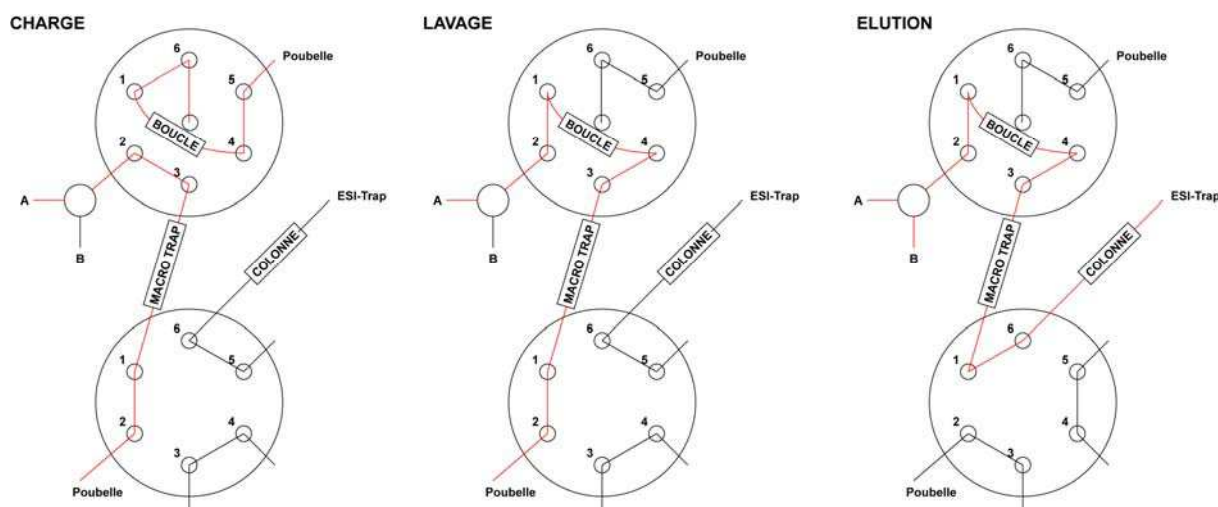
Figure 67. Schéma du système de LC couplé à l'ESI-Trap
