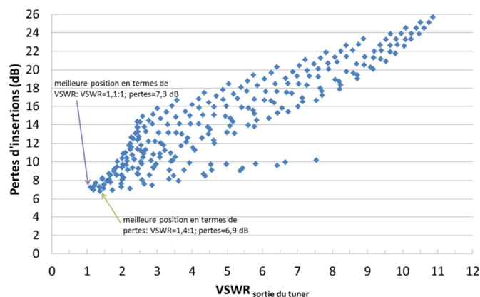
Figure 3 : Pertes d'insertions en fonction du VSWR_{\text{sortie du tuner}} , pour les 256 positions du tuner, chargé par l'antenne commerciale avec utilisateur
