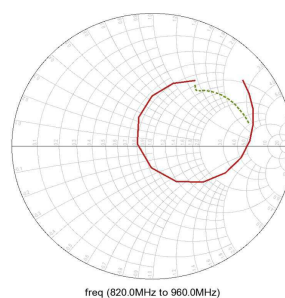
Figure 27 : Samsung Galaxy S 2 : S_{11} en fonction de la fréquence, comparaison en espace libre et avec la main de l'utilisateur (a) en dB, (b) bande basse sur abaque de Smith, (c) bande haute sur abaque de Smith
