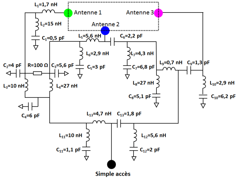
Figure 33 : Circuit permettant de recombinaer trois accès séparés en un accès unique
