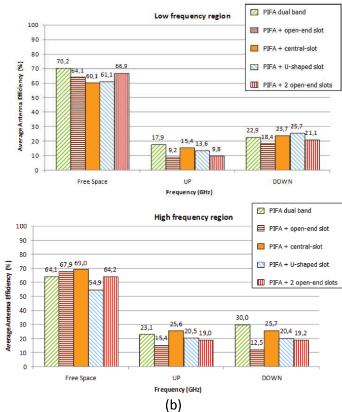
Figure 15 : Effet de la tête de l'utilisateur sur une antenne (a) description des deux positions de mesures avec tête, (b) mesure d'efficacité avec et sans la tête dans les 2 positions mentionnées en (a) moyennées dans les zones de fréquence où l'antenne avait un S_{11} < -6 dB [17]
