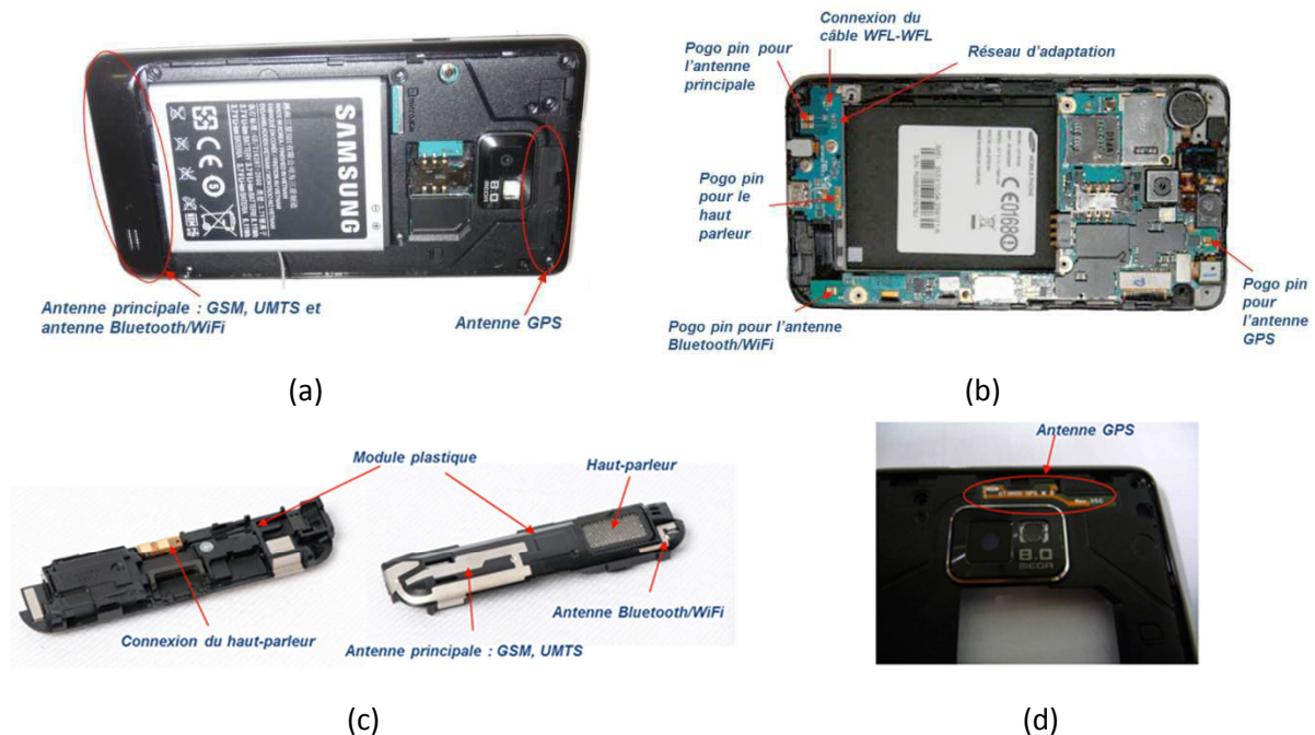
Figure 23 : Samsung Galaxy S 2 (a) vue du téléphone sans la partie du boîtier couvrant la batterie, (b) détail du PCB, (c) vues de dessus et de dessous du module antennaire, (d) antenne GPS
