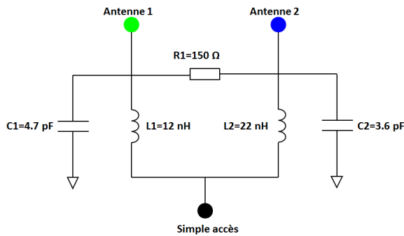
Figure 13 : Structure de combineur/diviseur de puissance
