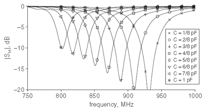
Figure 42 : Coefficient de réflexion d'une antenne reconfigurable [26]
