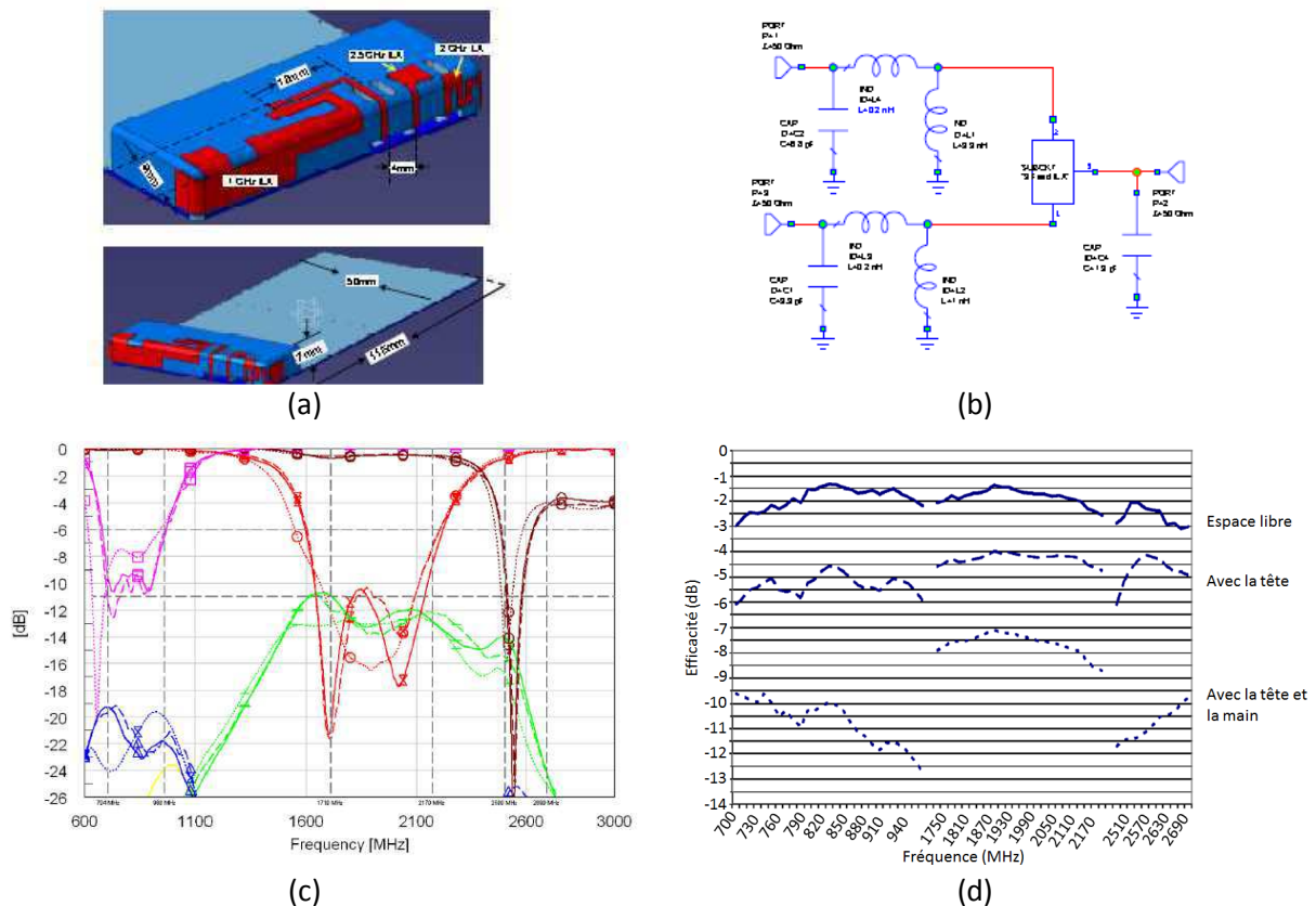
Figure 43 : Solution de Pulse Electronics (a) éléments rayonnants, (b) circuits, (c) S_{11} mesuré en espace libre (trait plein), avec la tête (pointillés larges), avec la tête et la main (pointillés), (d) efficacité mesurée en espace libre (trait plein), avec la tête (pointillés larges), avec la tête et la main (pointillés) [27]
