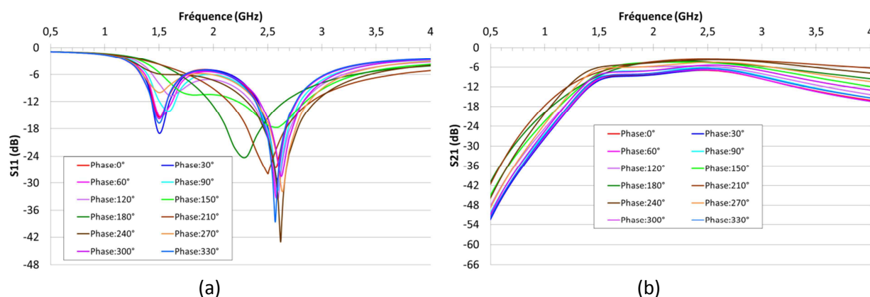
Figure 48 : Performances large bande du tuner pour les meilleures positions mesurées, optimisées à 2,6 GHz, présentées sur la bande [400 MHz-6 GHz], pour VSWR_{\text{antenne}}=5:1 (a) S_{11} , (b) S_{21} [37]
