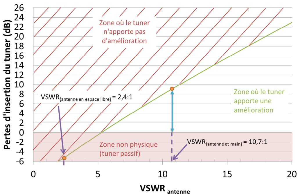
Figure 22 : Pertes d'insertion du tuner en fonction du \text{VSWR}_{\text{antenne}} en prenant en compte la désadaptation, la susceptibilité du PA à sa charge et la dégradation de l'efficacité de l'antenne par l'utilisateur
