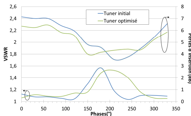
Figure 57 : Comparaison des VSWR et pertes d'insertion des deux tuneurs mesurés, pour les meilleures positions absolues de chaque tuner, à 2,6 GHz, pour un \text{VSWR}_{\text{antenne}}=5:1 [38]
