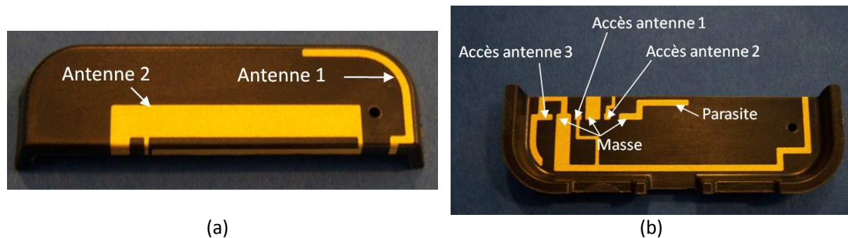
Figure 31 : Prototype d'antenne pour un fonctionnement sur trois bandes (a) vue de dessus, (b) vue de dessous
