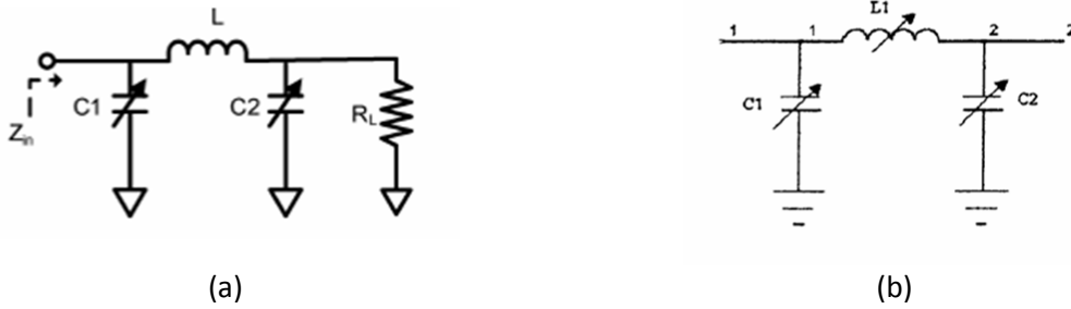
Figure 24 : Structures en pi à l'ordre 3 (a) avec inductance fixe [9], (b) avec inductance variable (non réalisée) [31]
