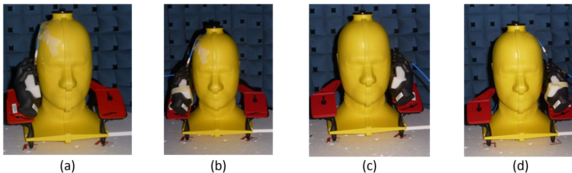
Figure 28 : Configuration de mesures (a) tête et main droite : cheek , (b) tête et main droite : tilt , (c) tête et main gauche : cheek , (d) tête et main gauche : tilt
