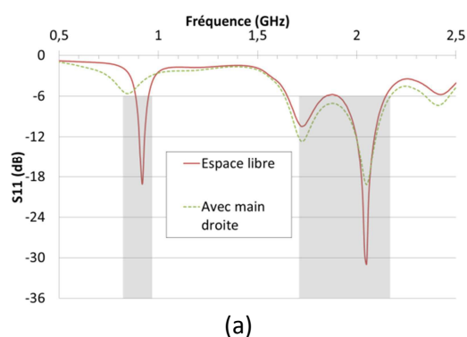
Figure 27 : Samsung Galaxy S 2 : S_{11} en fonction de la fréquence, comparaison en espace libre et avec la main de l'utilisateur (a) en dB, (b) bande basse sur abaque de Smith, (c) bande haute sur abaque de Smith
