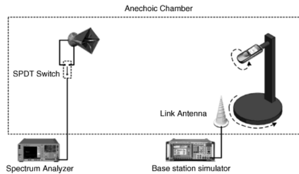
Figure 14 : Système de mesure de la TRP [1]
