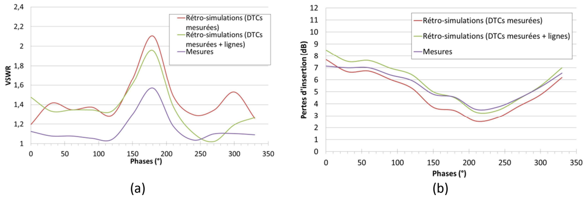
Figure 46 : Comparaisons entre les rétro-simulations (avec ou sans lignes) et les mesures, pour les meilleures positions mesurées pour VSWR_{antenne}=5:1 , à 2,6 GHz (a) VSWR, (b) pertes d'insertion [37]
