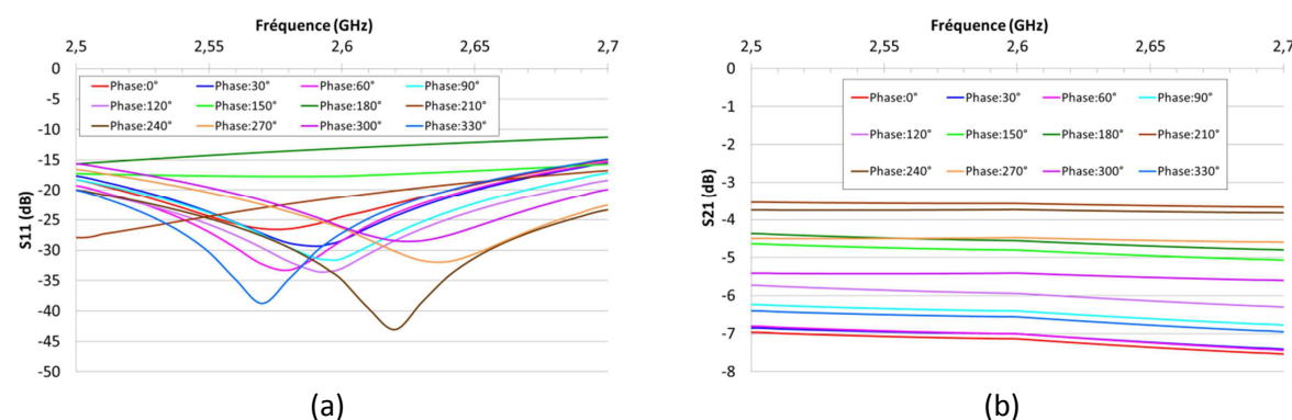
Figure 49 : Performances du tuner pour les meilleures positions mesurées, optimisées à 2,6 GHz, présentées sur la bande de fonctionnement [2,5-2,69 GHz], pour VSWR_{\text{antenne}}=5:1 (a) S_{11} , (b) S_{21} [37]
