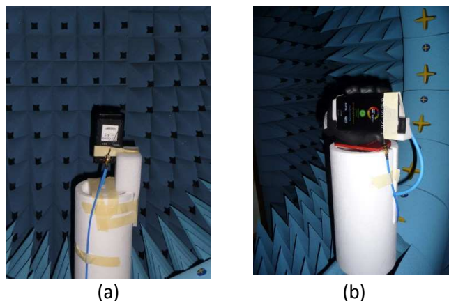
Figure 26 : Configuration de mesure du S_{11} du Samsung Galaxy S 2 (a) espace libre, (b) avec la main droite
