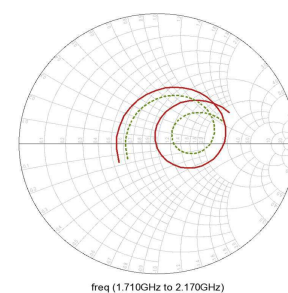
Figure 27 : Samsung Galaxy S 2 : S_{11} en fonction de la fréquence, comparaison en espace libre et avec la main de l'utilisateur (a) en dB, (b) bande basse sur abaque de Smith, (c) bande haute sur abaque de Smith
