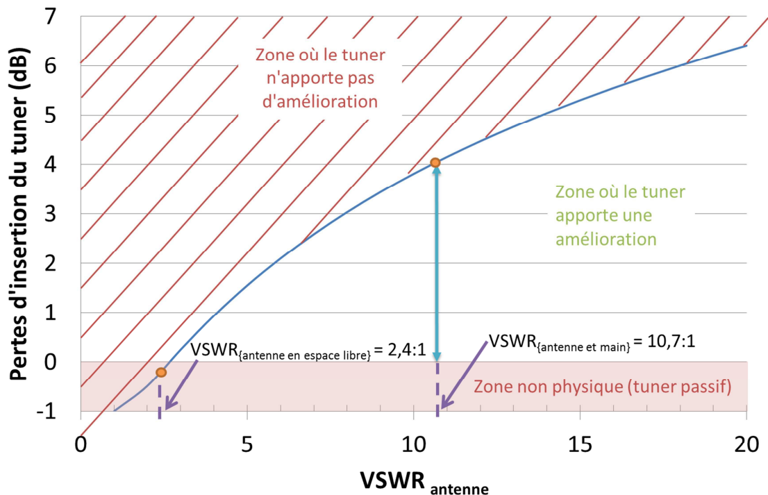
Figure 5 Pertes d'insertion du tuner en fonction du VSWR_{antenne}
