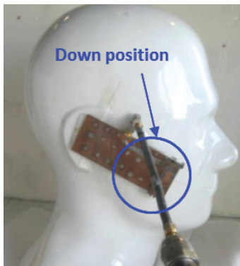
Figure 15 : Effet de la tête de l'utilisateur sur une antenne (a) description des deux positions de mesures avec tête, (b) mesure d'efficacité avec et sans la tête dans les 2 positions mentionnées en (a) moyennées dans les zones de fréquence où l'antenne avait un S_{11} < -6 dB [17]
