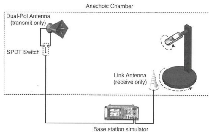
Figure 16 : Système de mesure de la TIS [1]
