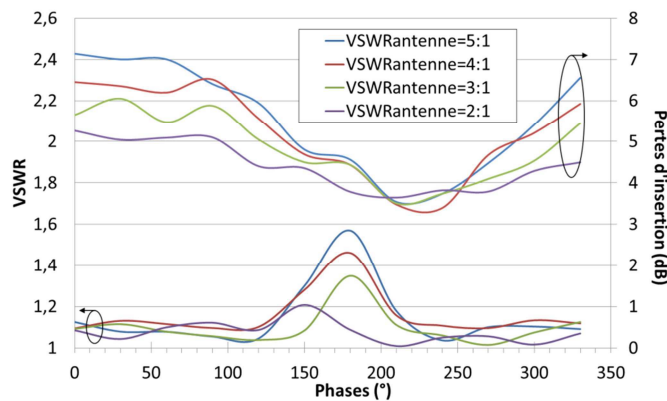
Figure 47 : VSWR et pertes d'insertion pour VSWR_{antenne}=5:1 , à 2,6 GHz [37]
