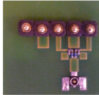
Figure 14 : Réalisation du combineur/diviseur de puissance sur PCB
