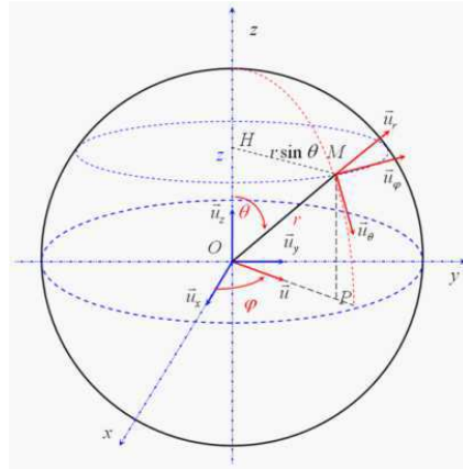
Figure 1 : Repère de coordonnées sphériques [5]
