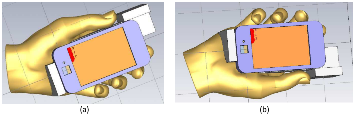
Figure 36 : Simulation MWS de l'antenne multibande en présence d'une main PDA [25] (a) main gauche, (b) main droite
