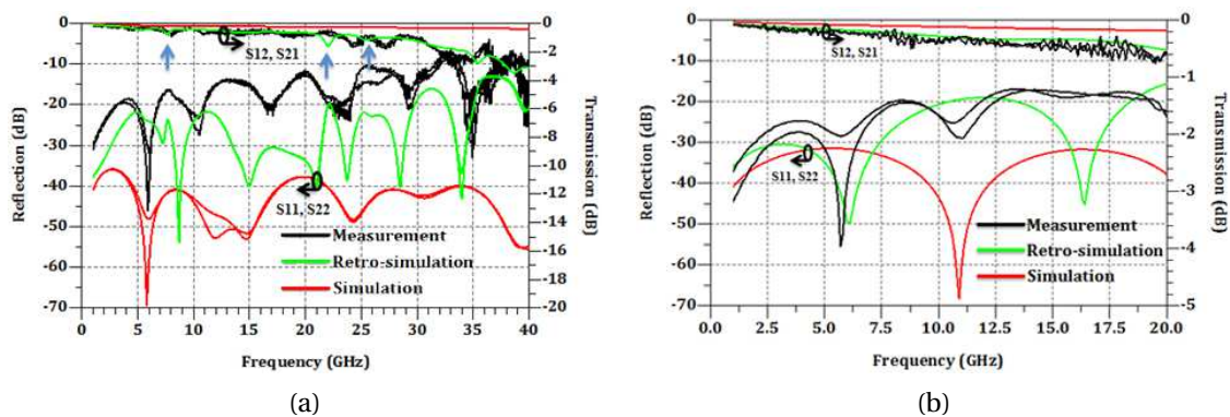
Figure 5: Simulation, mesure and retro-simulation des lignes de transmission : (a) Ligne micro-ruban. (b) Ligne coplanaire avec un plan de masse en dessous
