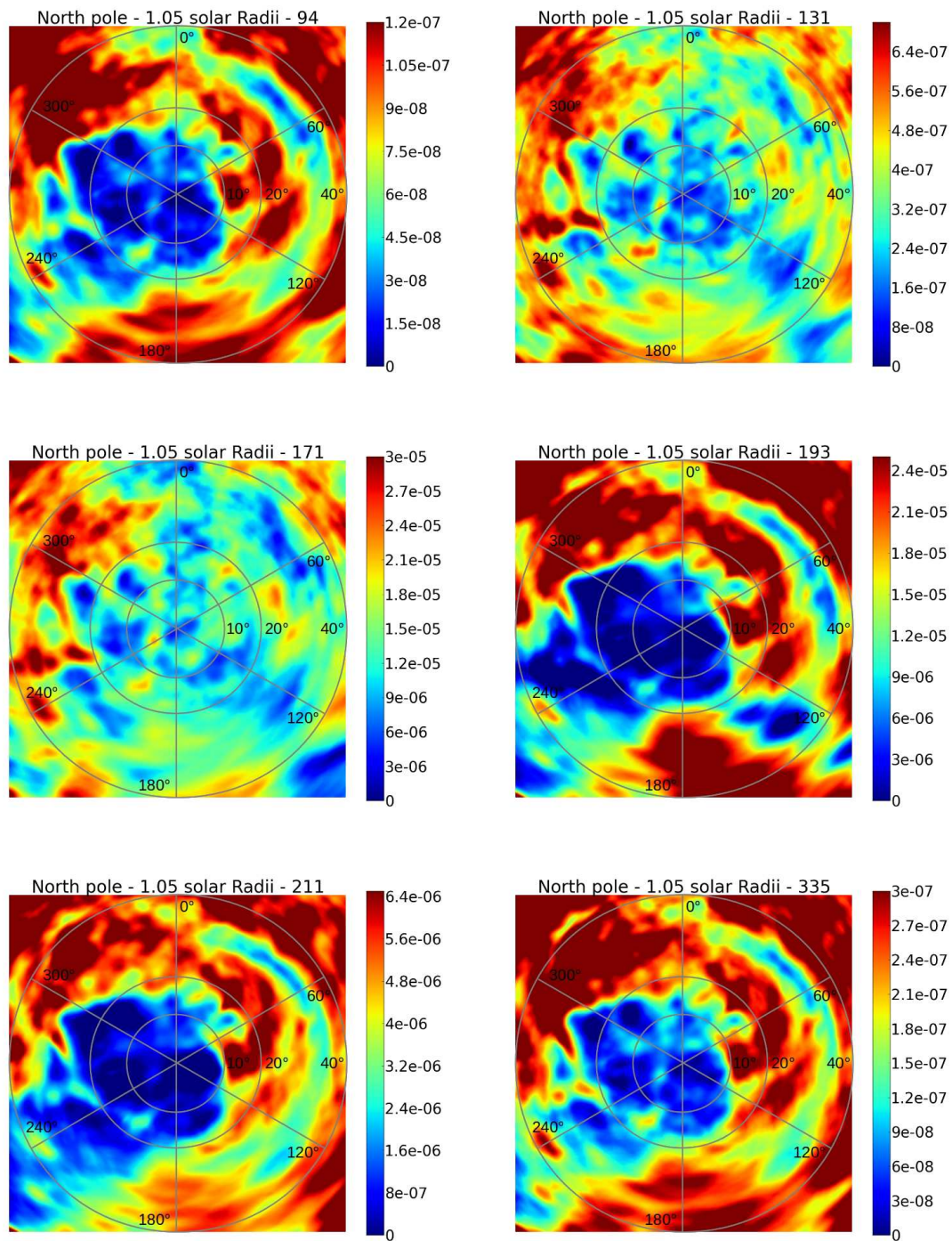
FIGURE 5.6: Projections gnomoniques du pôle Nord de l'émissivité [ \text{DN.m}^{-1} ] à l'altitude constante de 1.05 R_{\odot} , pour les 6 bandes spectrales de l'instrument AIA, et obtenues à partir des reconstructions calculées pour 14 jours de données.
