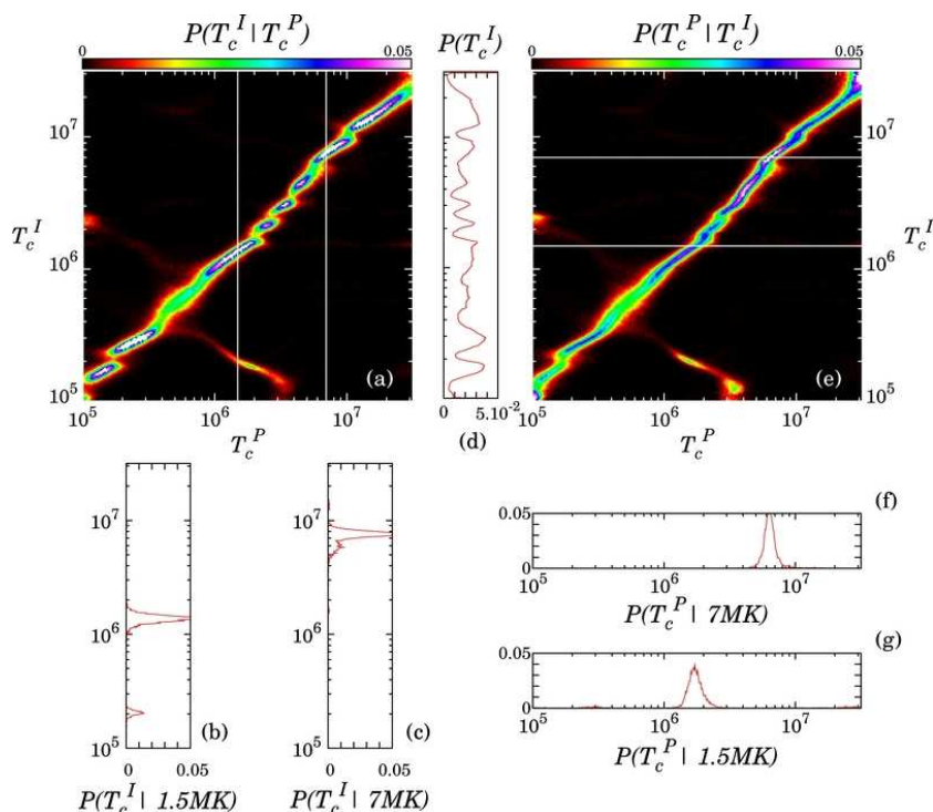
FIGURE 3.14: Cartes de probabilités identiques à la figure 3.8, mais dans le cas où le plasma observé est caractérisé par une DEM Gaussienne de largeur \sigma^P = 0.1 \log T_e (i.e plasma multitherme).
