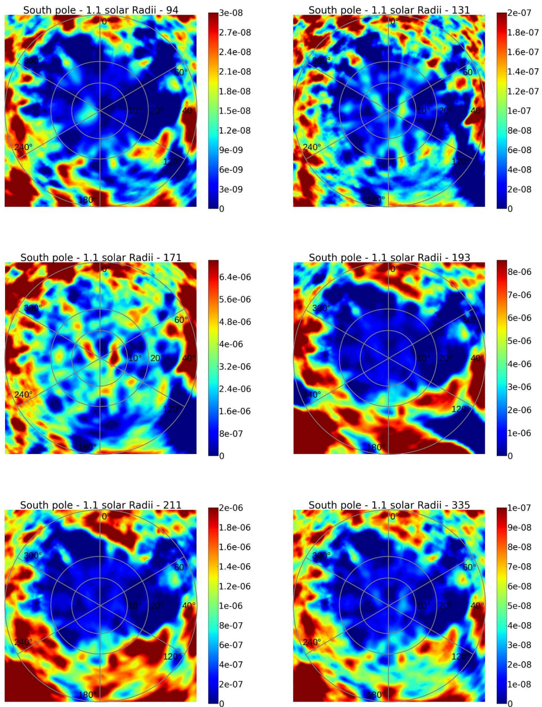
FIGURE 5.8: Projections gnomoniques du pôle Sud de l'émissivité [\text{DN}\cdot\text{m}^{-1}] à l'altitude constante de 1.1 R_{\odot} , pour les 6 bandes spectrales de l'instrument AIA, et obtenues à partir des reconstructions calculées pour 14 jours de données.
