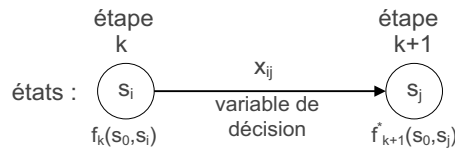
Figure 1.11 : Structure basique de la programmation dynamique
