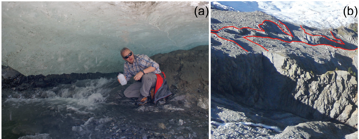
Figure 2.9 : (a) Photographie d'un chenal sous-glaciaire au front du glacier des Bossons en 2009 ; (b) Paléocheanal récemment exposé incisant le substratum à l'avant du glacier des Bossons.
