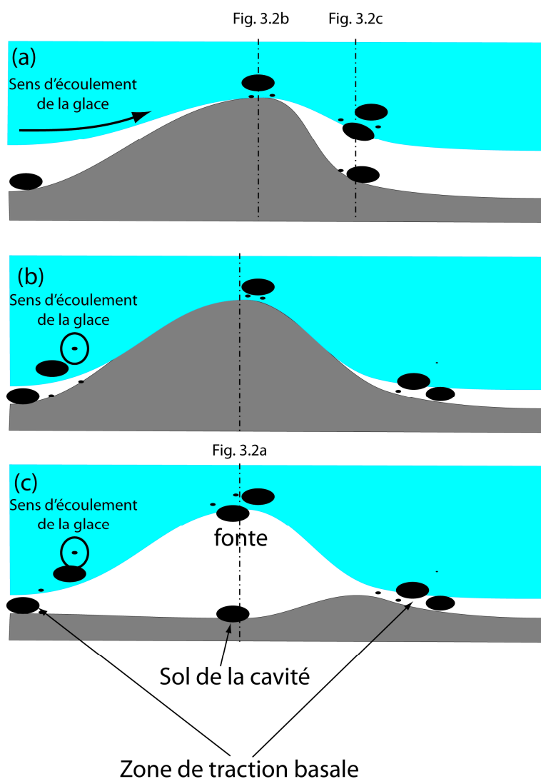
Figure 3.2 : Représentation schématique d'une cavité sous-glaciaire à l'aval d'une bosse du socle (a) et transport des sédiments dans la glace basale, et coupes schématisées transverses au sens d'écoulement de la glace en amont de la cavité (b) et dans la cavité (c).
