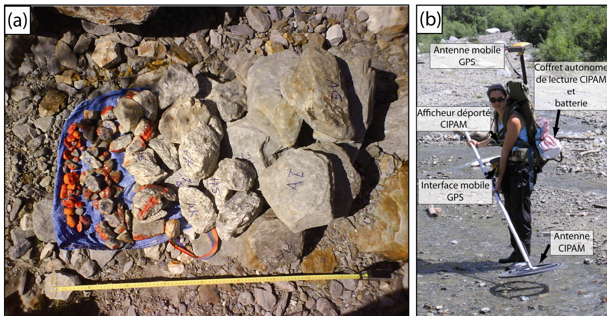
Figure 5.9 : a. Galets des différentes classes granulométriques pucés, b. Dispositif de suivi radiofréquence des galets, c. Antenne base HiPer®pro Topcon.
