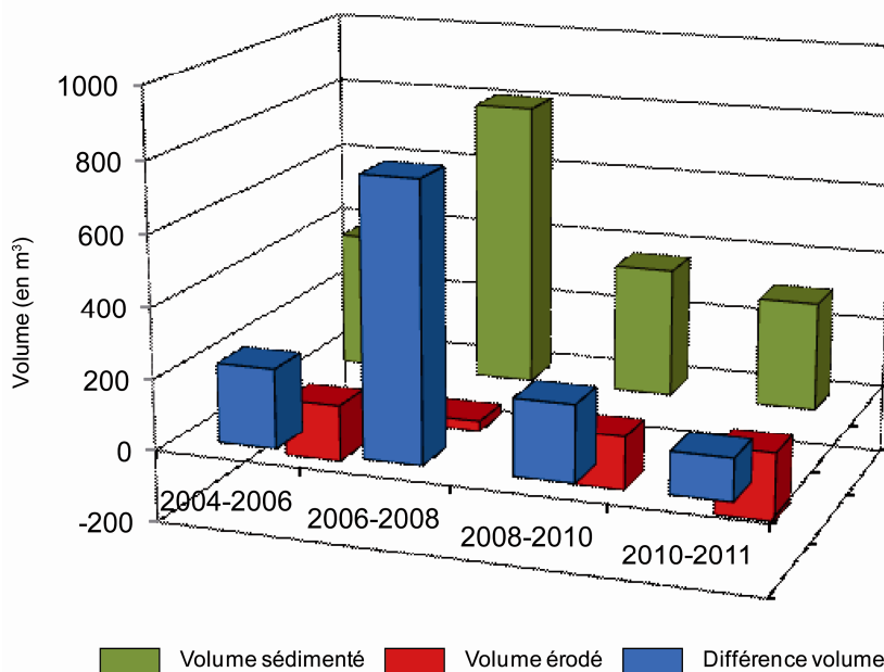
Figure 5.4 : Volumes annuels de sédiments accumulés (en vert) et érodés (en rouge) et différence (en bleu) entre les années 2004-2006, 2006-2008, 2008-2010 et 2010-2011 dans la partie aval du plan des eaux.
