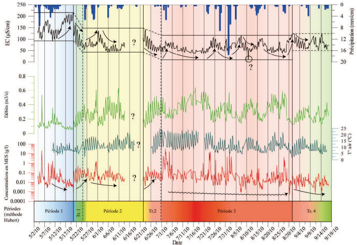
Figure 2.11 : Comparaison entre signaux des conditions de températures et de précipitations et du débit au cours de la saison d'ablation 2010 et signaux sédimentaires observés sur le torrent des Bossons : EC (conductivité électrique) et concentrations de matières en suspension (MES). Le cartouche en bas de graphique délimite différentes périodes et transitions au cours de la saison de fonte obtenues par la segmentation de Hubert (Goupy, 2011).
