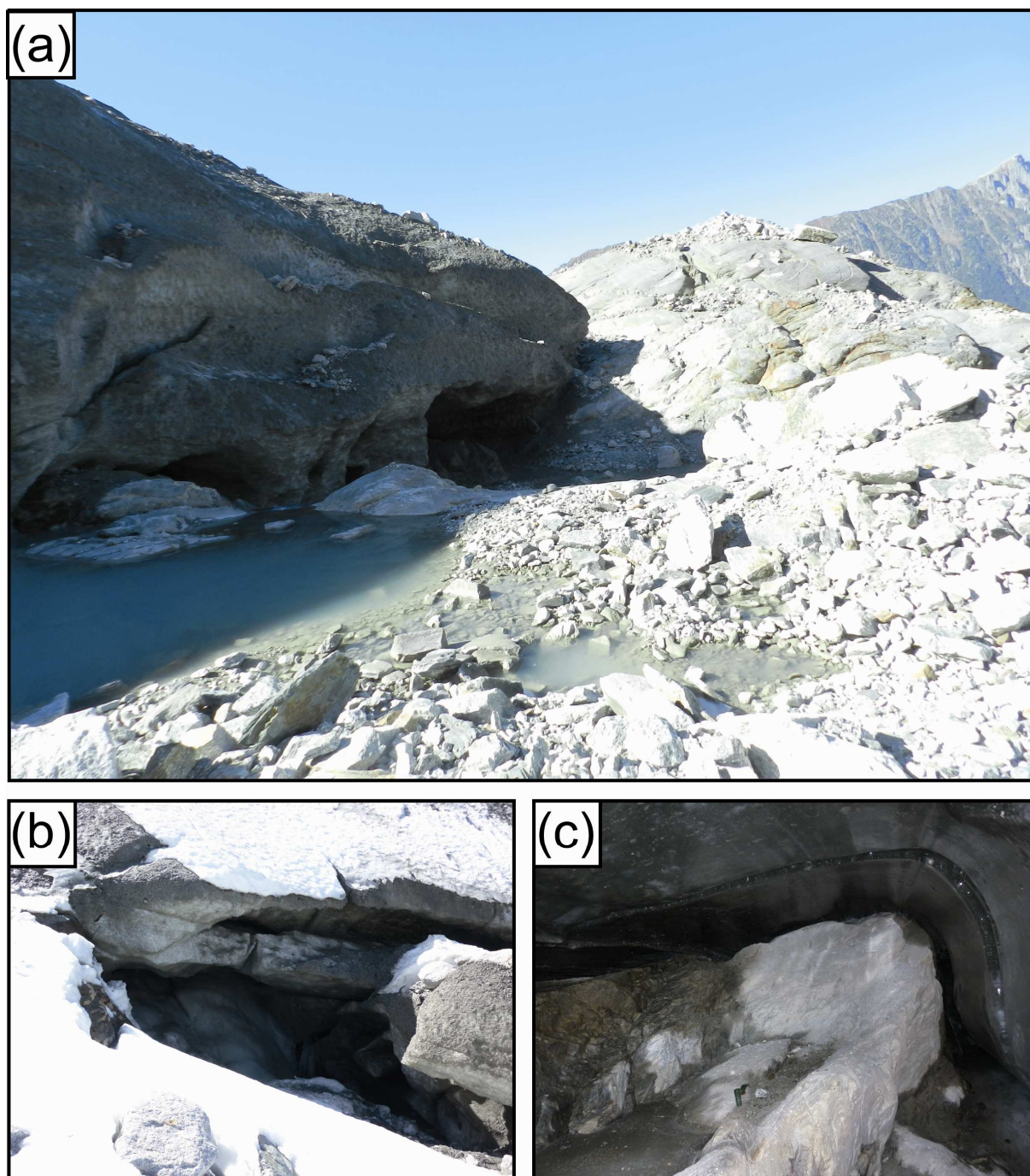
Planche 3.1 : a. Nombreuses cavités au front du flanc droit du glacier des Bossons ; b. Entrée d'une cavité sous glaciaire ; c. Relief rocheux sous glaciaire à l'amont d'une cavité.
