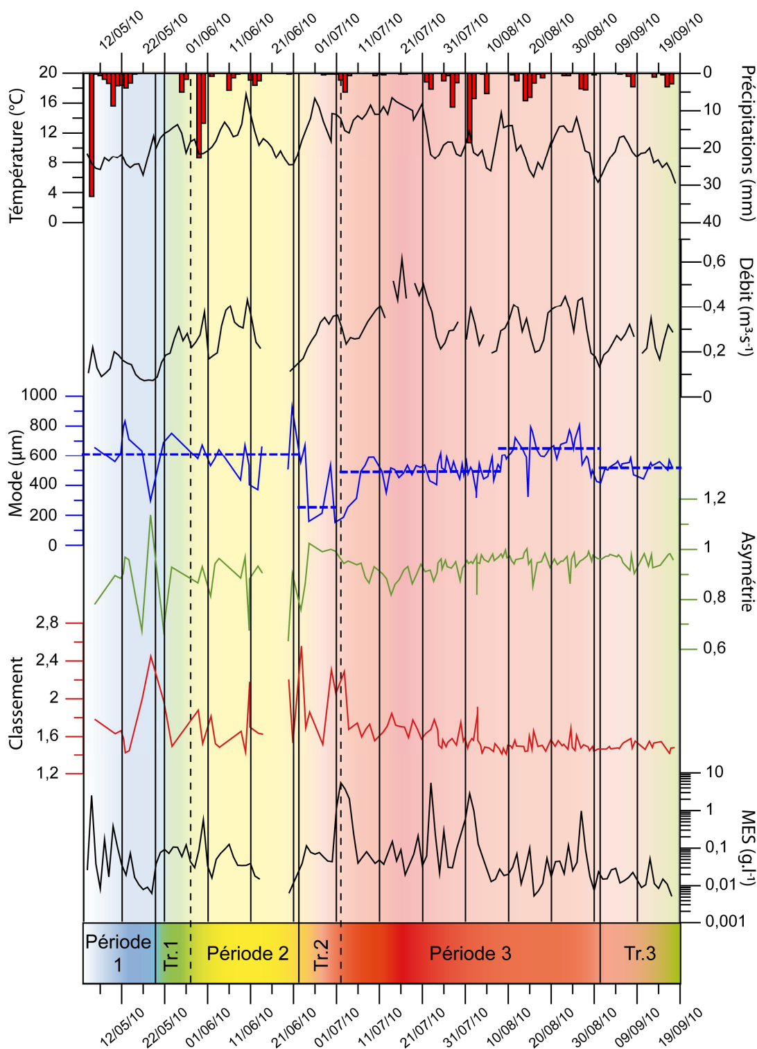
Figure 4.17 : Evolution temporelle de la température de l'air moyenne quotidienne (premier graphique, courbe noire) des précipitations quotidiennes cumulées (histogramme rouge), des débits, des paramètres granulométriques de la charge piégée à 5cm du fond (mode, asymétrie et classement) et de la concentration moyenne journalière en MES du torrent des Bossons entre le 3 Mai 2010 et le 17 Septembre 2010. Les différentes périodes et transitions au cours de la saison de fonte obtenues par la segmentation de Hubert par Goupy (2011) sont indiquées dans le cartouche en bas des graphiques. Les moyennes du mode principal de la charge piégée à 5cm du fond de chaque segment obtenu par la segmentation de Hubert sont représentées par des traits pointillés bleus sur la courbe correspondante.
