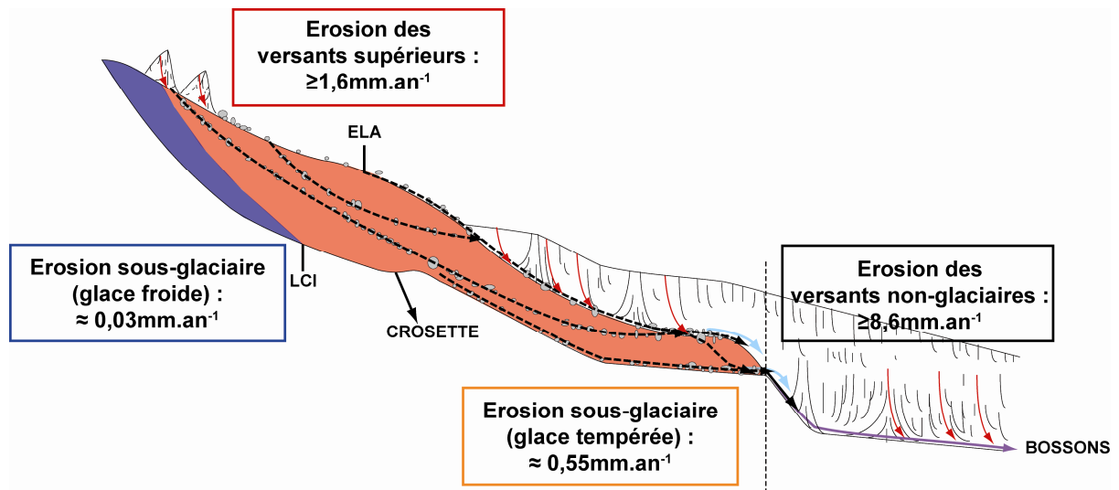
Figure II : Taux d'érosion glaciaire et non glaciaire ( \text{mm.an}^{-1} ) sur une représentation schématique du Glacier des Bossons. La glace froide est représentée en bleu et la glace tempérée en rouge. Ces taux ont été obtenus en pondérant les flux calculés (Fig. 3.25) par les surfaces des différents domaines (Annexe C).
