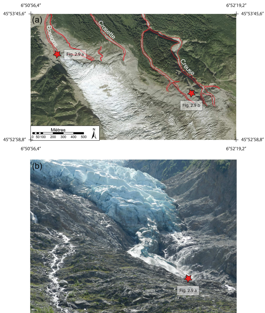
Figure 2.10 : a) Photographie aérienne de la partie basse du glacier des Bossons montrant les principaux exutoires et la marque de certains paléo-chenaux ; b) Photographie de la surface dégagée à l'avant du front du glacier montrant la structure des roches moutonnées ainsi que les suintements d'eaux en Juin 2011.
