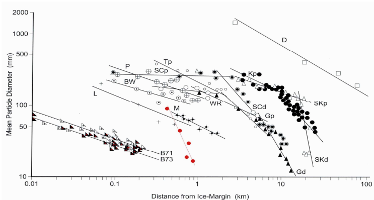
Figure 2.24 : Affinement granulométrique spatial du diamètre moyen des particules dans divers torrents d'eau de fonte glaciaire modernes. B71 et B73 : Bossons (respectivement en 1971 et 1973) (Maizels, 1976) ; ronds rouges : Bossons 2011 (Godon, cette thèse) ; BW : Bow River, Alberta (Mc Donald et Banerjee, 1971) ; D : Donjek River, Yukon (Rust, 1972) ; G : Gigjukvisl, Skeiðararsandur, Island (Boothroyd et Nummedal, 1978) ; K : Knik River, Alaska (Bradley et al. , 1972) ; L : Lewis River, Baffin Island (Church, 1972) ; M : Mendehall outwash, Alaska (Ehrlich et Davies, 1968) ; P : Peyto outwash, Alberta (McDonald et Banerjee, 1971) ; SC, Scott outwash, Alaska (Boothroyd et Nummedal, 1978) ; T : Tingine outwash (Church, 1972) ; WR, White River, Washington State (Fahnestock, 1963) ; d : zone distale et p : zone proximale. (modifié de Maizels, 1976).
