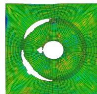
délamination (pli 3//pli 4 de la plaque)
