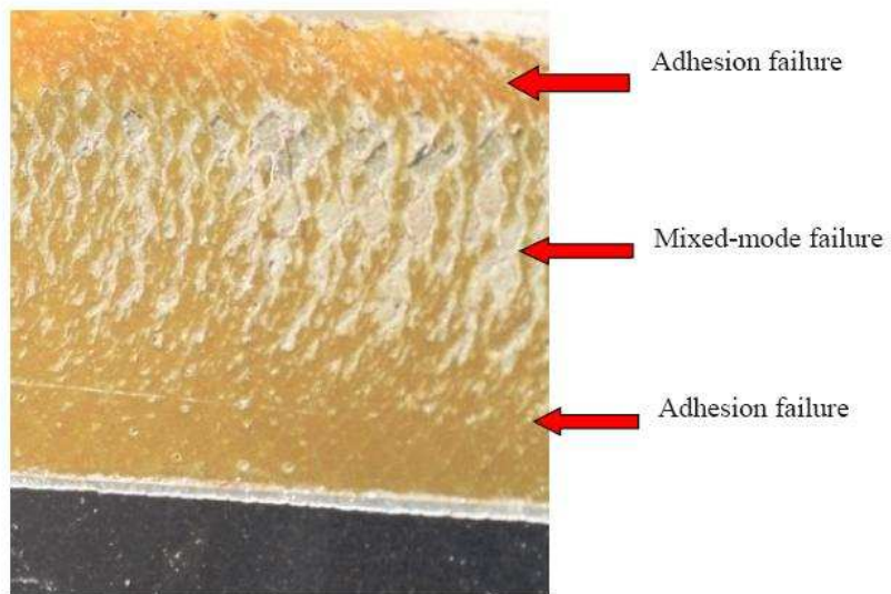
Figure I.26 Rupture mixte [23]
