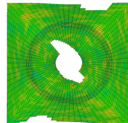
délamination pli 1//pli 2 de la plaque
