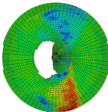
délamination (adhésif//patch)
