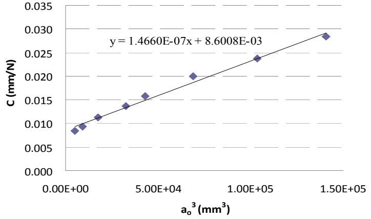
Figure II.18 Interpolation de C en fonction d 3 (MMF)
