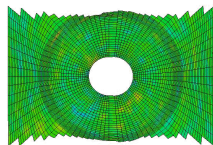
délamination (pli 4//pli -4 de la plaque)
