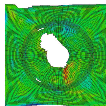
délamination (pli 1//pli 2 de la plaque)
