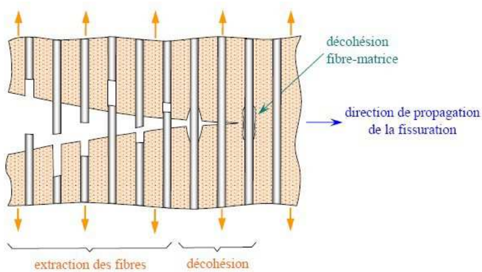
Figure I.16 Propagation de la rupture dans le cas d'une faible adhérence fibre-matrice [14]
