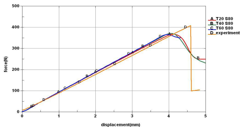
Figure II.35 Influence de la résistance d'interface en traction \sigma_{I,max} sur le mode mixte
