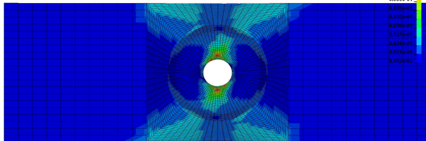
rupture en cisaillement (pli 1 de la plaque)
