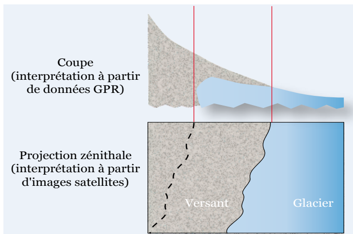
Figure 68 – La limite glacier/versants est extrêmement difficile à déterminer à cause de l'instabilité des versants, dont les débris ennoient une partie des flancs du glacier. Les mesures au GPR ont montré une configuration proche de celle représentée ici.
