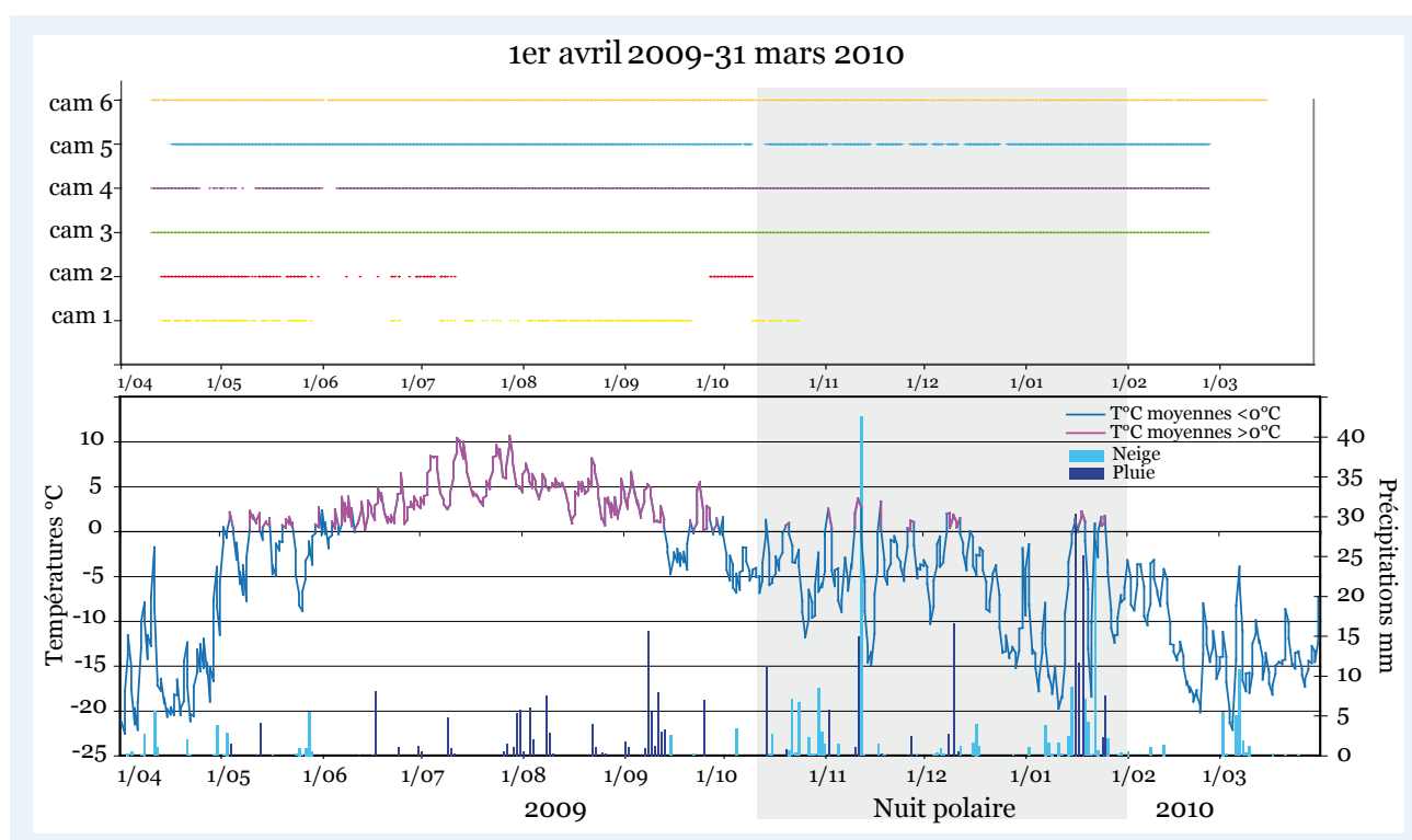
Figure 96 – Fonctionnement des stations-photos. Chaque point représente une photo prise. On constate la majorité des dysfonctionnements dans la zone autour de 0°C et avec un climat humide. Les stations les plus hautes (1 et 2, col du Slatto) sont les plus exposées et les moins performantes sans doutes parce que les moins souvent visitées.
