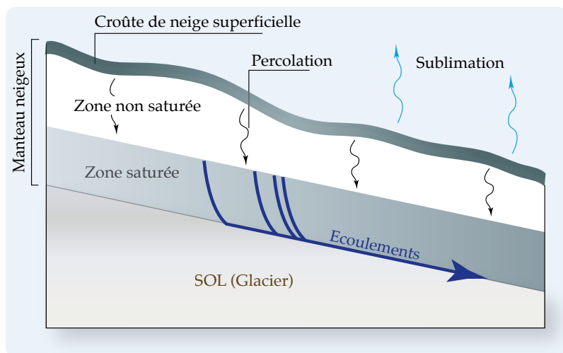
Figure 63 – Les écoulements au sein du manteau neigeux.
