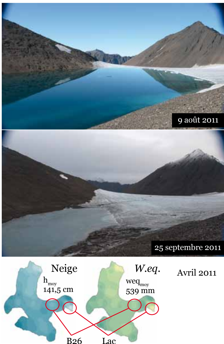
Figure 185 – Le lac supra-glaciaire et ses répercussions sur la fonte nivale. La vidange du lac s'effectue par un chenal dont l'exutoire est situé plus bas dans la pente au niveau du point B26. Les hauteurs de neige comme les équivalents-eau sont, à ces endroits, nettement moindres.
