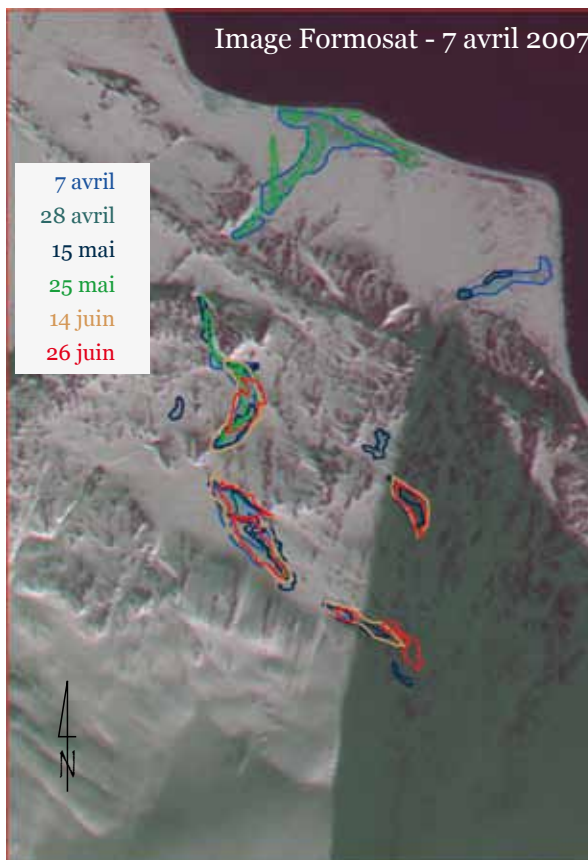
Figure 153 – Détourage des marges glacées. Les images satellite permettent de suivre l'enneigement, mais ne sont pas représentatives de ces dynamiques. En revanche, le suivi des marges glacées est efficace et permet d'observer l'avancée de l'eau au printemps (d'après HSF).
