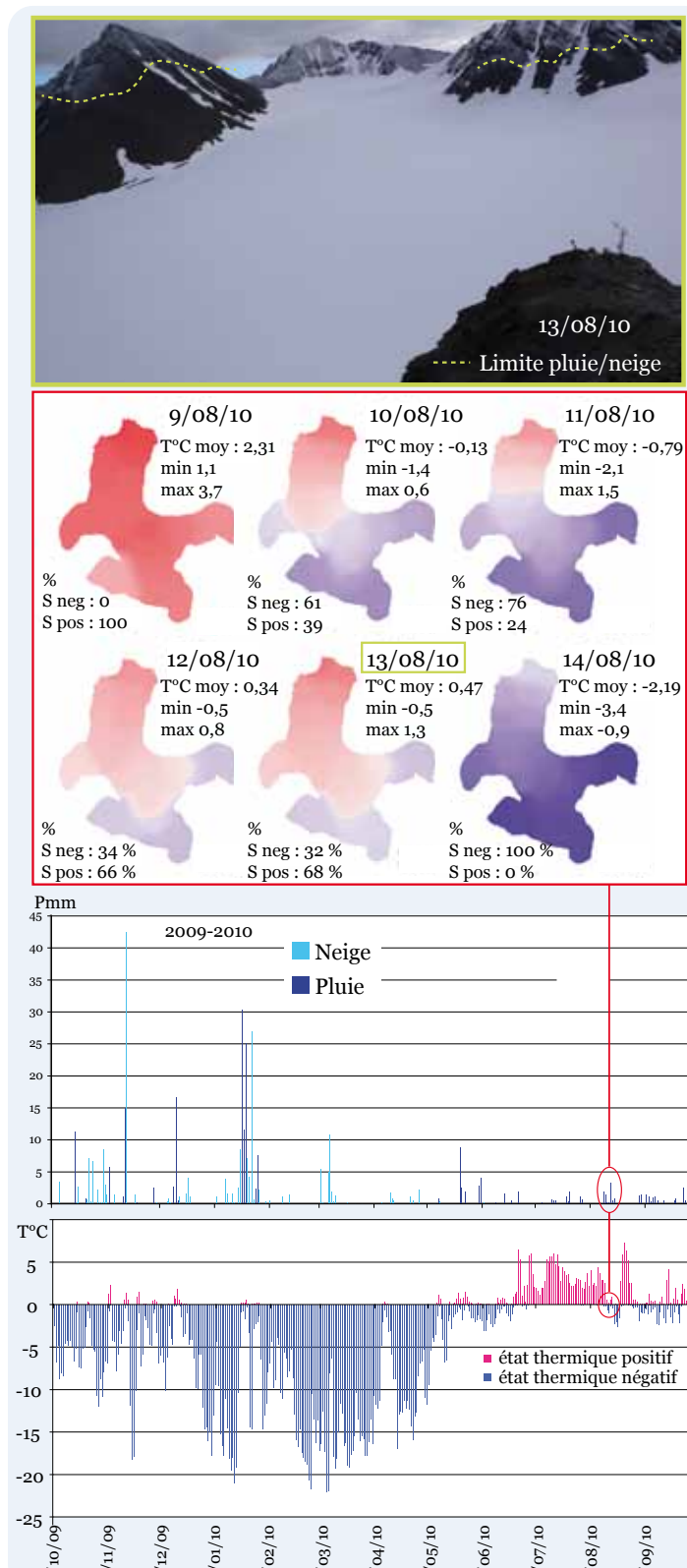
Figure 151 – L'événement froid d'août 2010. La combinaison des états thermiques de l'Austre Lovénbreen et l'utilisation des images in situ permet de déterminer la limite pluie neige. Sur cet exemple, il faut chercher haut la neige alors que la pluie est tombée sur une bonne partie du glacier.
