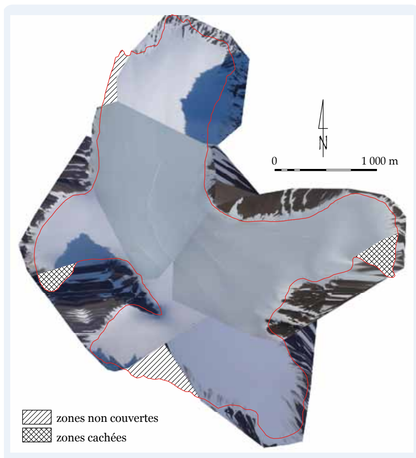
Figure 139 – La mosaïque construite avec les photos référentielles (celles où le plus de marqueurs étaient visibles) donne une couverture optimale du glacier. Sa surface est couverte à 96 % avec quelques zones cachées à cause de la topographie. Les versants présentent un aspect « étiré » dû au choix de favoriser la qualité de la correction géométrique sur le glacier.
