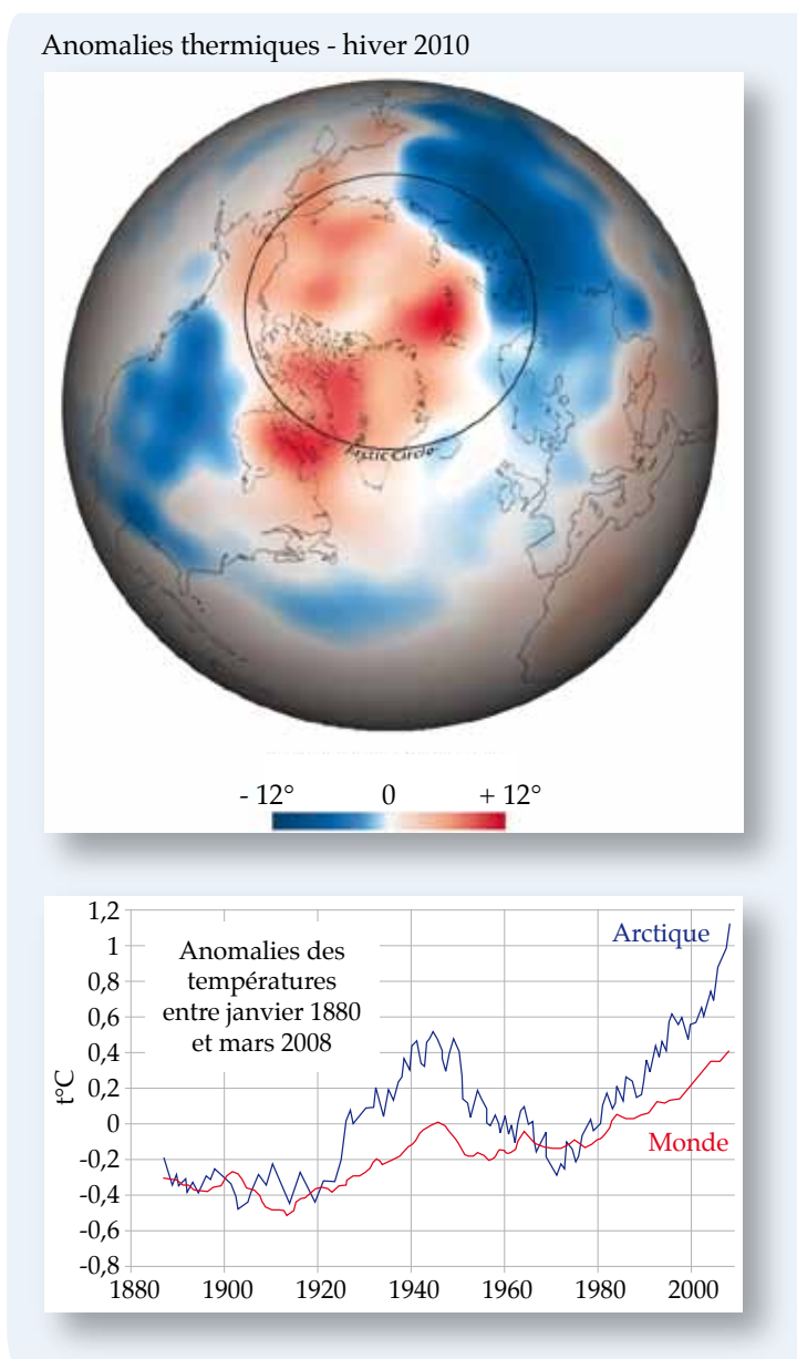
Figure 8 – L'Arctique face aux anomalies climatiques globales semble plus touché par le réchauffement. L'hiver 2010 représenté sur la mappemonde en est un bon exemple. Les glaciers et grandes calottes en sont ainsi les premiers affectés comme le montre le graphique issue des travaux du SWIPA (Snow, Water, Ice, Permafrost in Arctic, d'après SWIPA 2011).
