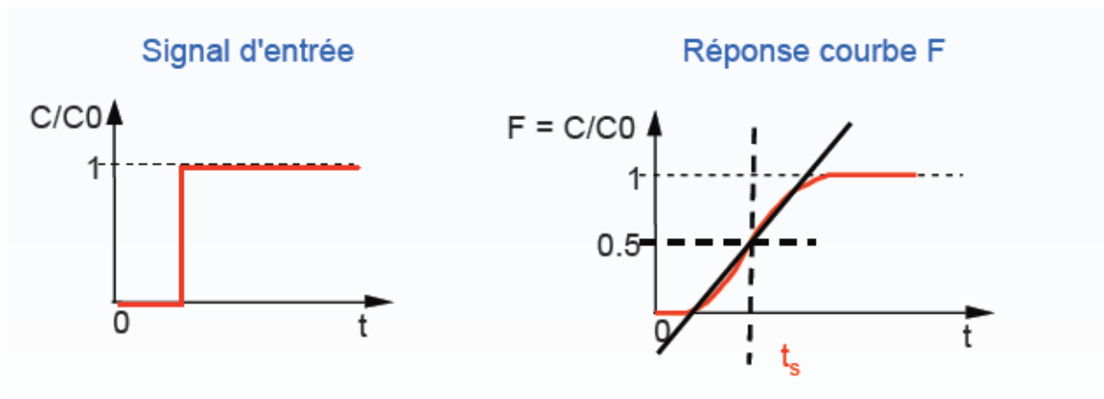
Figure 22 : Type d'injection adoptée et courbe d'élution associée
