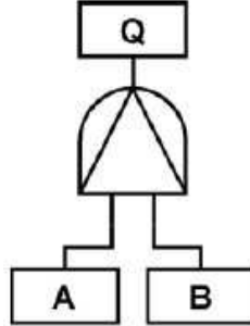
Figure 1.3 – Représentation d'une porte PAND
