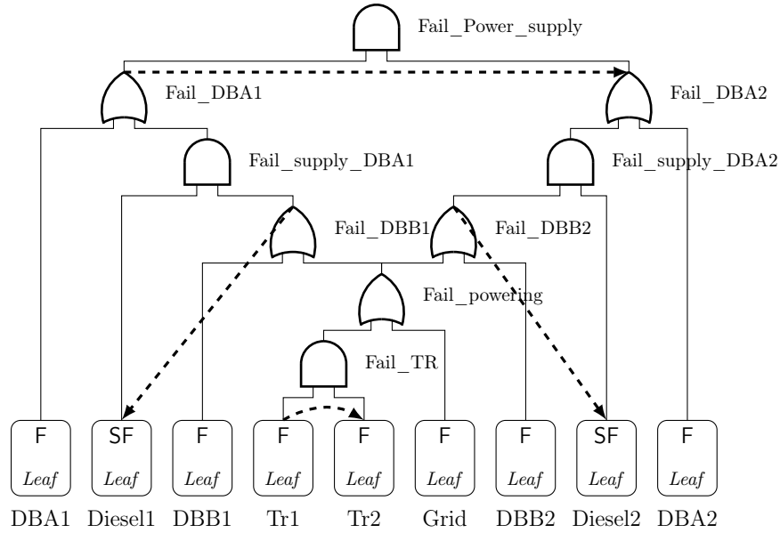
Figure 4.8 – Modèle BDMP du système d'alimentation
