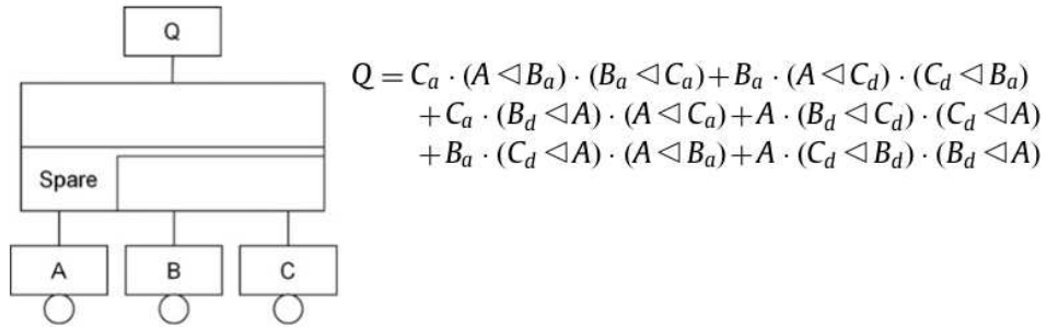
Figure 1.7 – Traduction formelle du comportement d'une porte Spare [MRL11].
