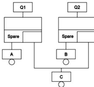
Figure 1.5 – Partage de composant entre deux portes SPARE
