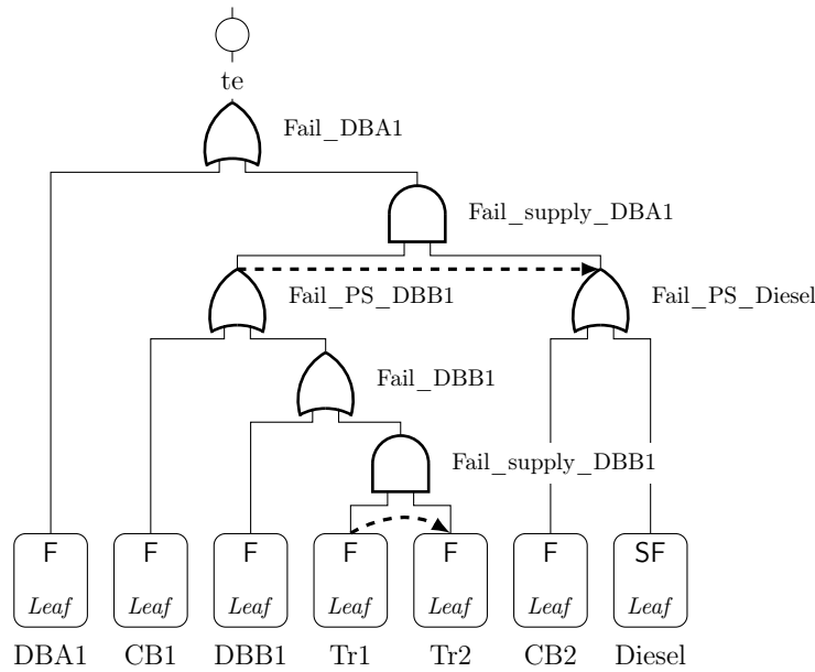
Figure 1.16 – Exemple de BDMP
