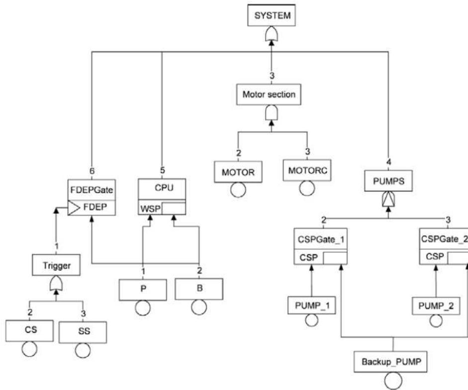
Figure 1.10 – Arbre de défaillance dynamique représentant la sûreté du système HCAS [BD05].
