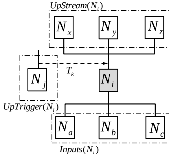
Figure 3.3 – Situation d'un noeud N_i \in N d'un BDMP
