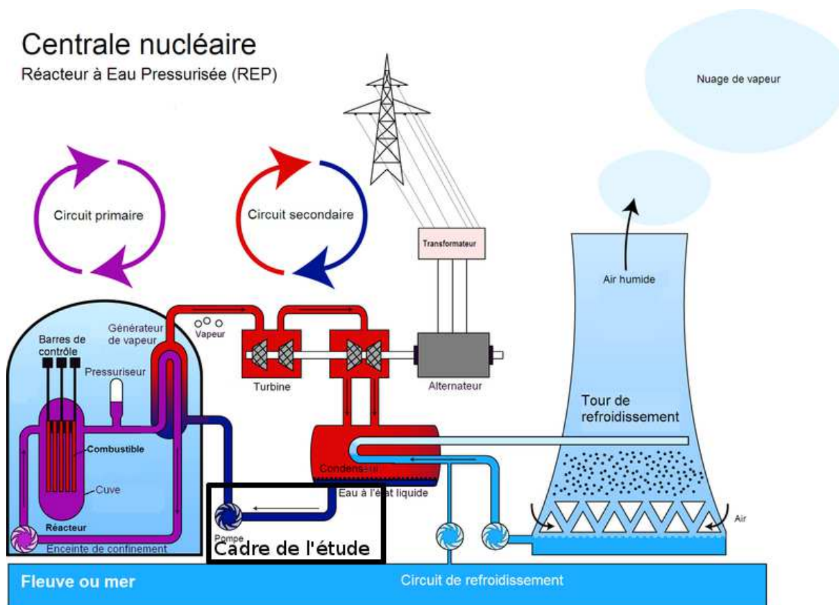
Figure 4.1 – Architecture simplifiée d'un Réacteur à Eau Pressurisée (REP)
