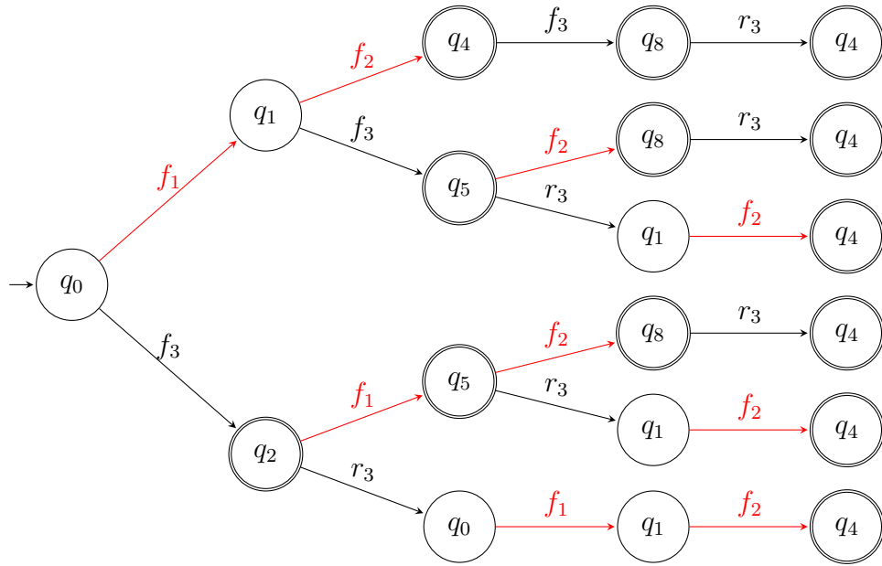
Figure 2.12 – Séquences générées par ajout de \delta = f_3r_3 dans \sigma = f_1f_2 .
