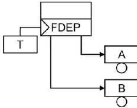
Figure 1.6 – Représentation d'une porte FDEP
