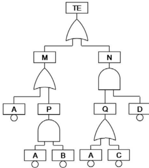
Figure 1.1 – Exemple d'arbre de défaillance
