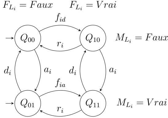
Figure 3.4 – Enveloppe du comportement d'une feuille L_i .
