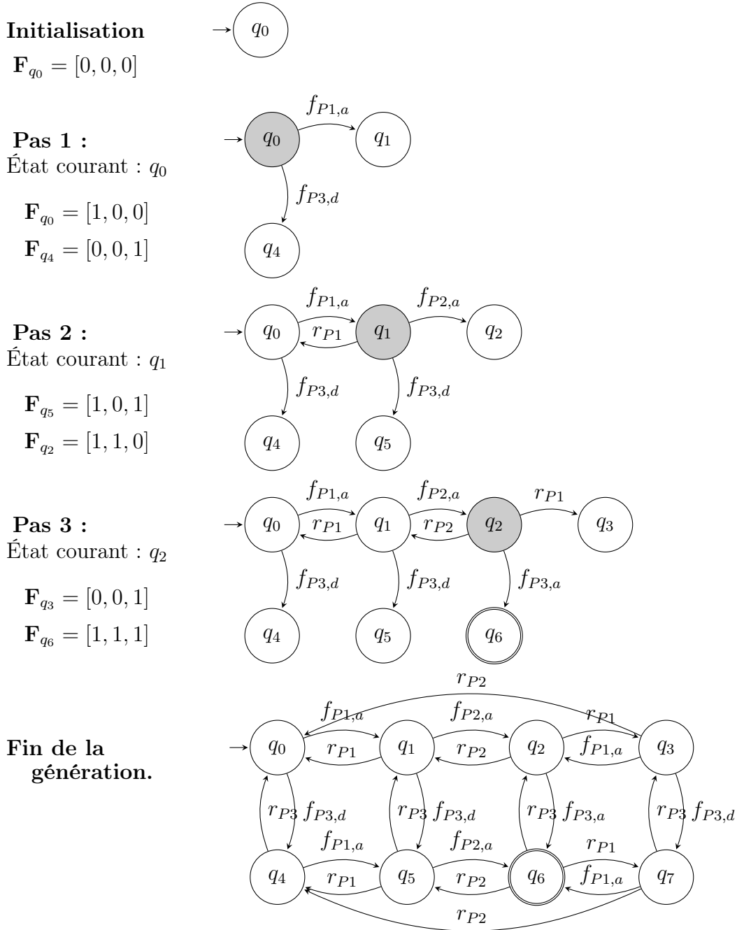
Figure 3.6 – Phases de calcul de l'automate fini equivalent au BDMP de la figure 3.2.
