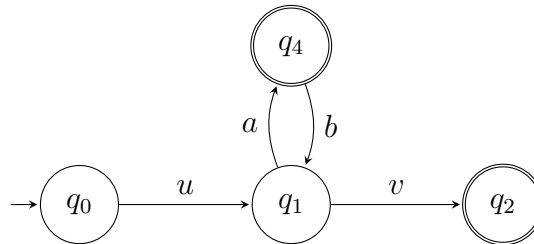
Figure 2.15 – Exemple de séquence défaillante passant deux fois dans le même état
