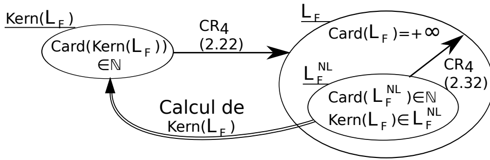
Figure 2.16 – Relations entre le noyau du langage défaillant, l'ensemble des séquences défaillantes sans boucles et le langage défaillant.
