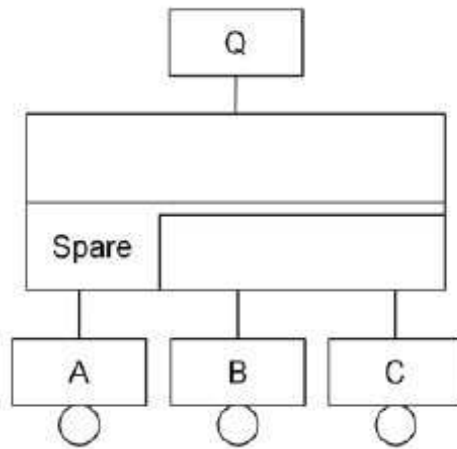
Figure 1.4 – Représentation d’une porte SPARE
