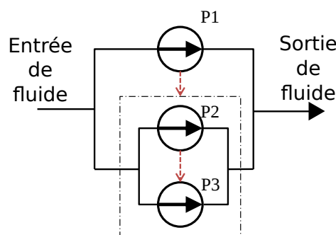
Figure 3.1 – Exemple support pour l'analyse d'un BDMP
