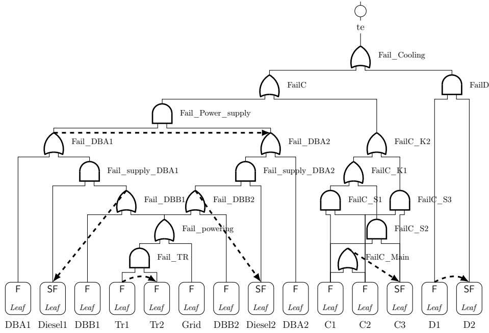
Figure 4.9 – Modèle BDMP de la sûreté du système aval au condenseur.
