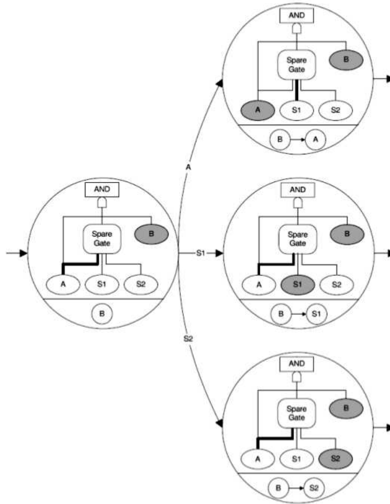
Figure 1.8 – Représentation des scénarios d'un ADD par un failure automaton.
