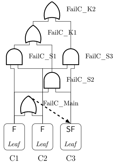
Figure 4.7 – Modèle BDMP des pompes d'extraction
