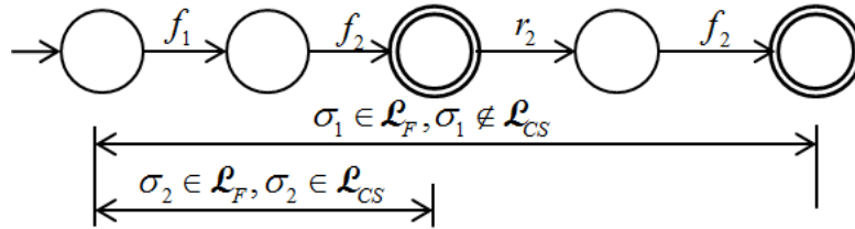
Figure 2.3 – Relation d'inclusion entre séquences de coupes et séquences défaillantes
