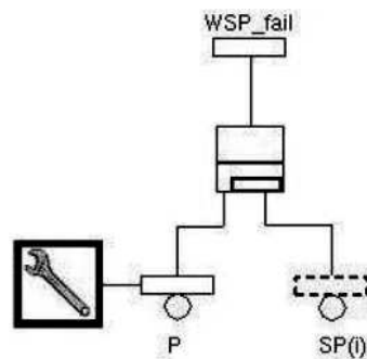
Figure 1.11 – Ajout de la réparabilité d'un composant par Repair Box[BR04]
