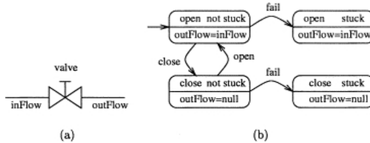
Figure 1.19 – Exemple d'automate de mode pour la description de comportement d'une vanne [Rau02]
