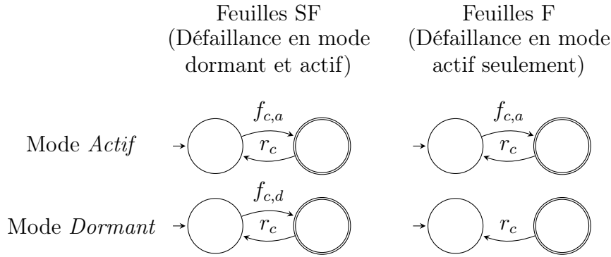
Figure 3.8 – Modèle de composant c d'un BDMP
