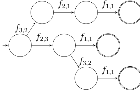
Figure 3.9 – Ajout d'un événement de défaillance dans une séquence défaillante de composants multimodes
