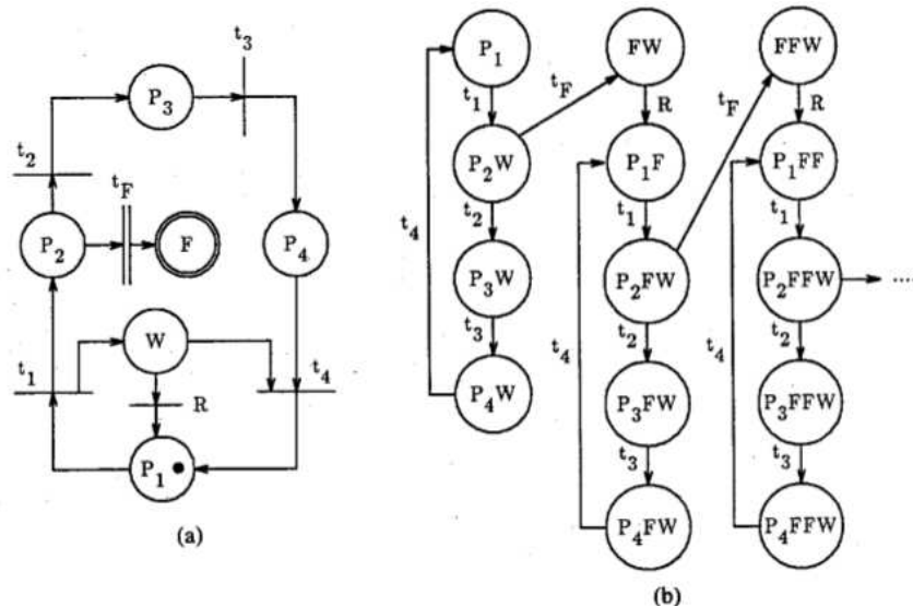
Figure 1.22 – Exemple de réseau de Petri modélisant une faute à l'aide d'une transition t_F (a) et son graphe d'accessibilité (b) [LS87]
