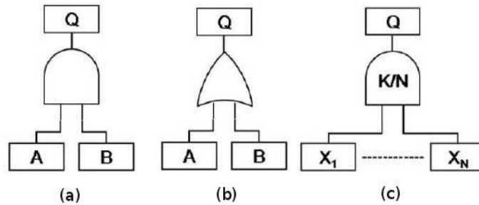
Figure 1.2 – Représentation des portes d'un arbre de défaillance
