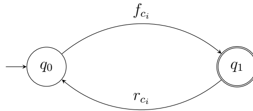
Figure 2.4 – Modèle générique d'un composant réparable d'un système dynamique
