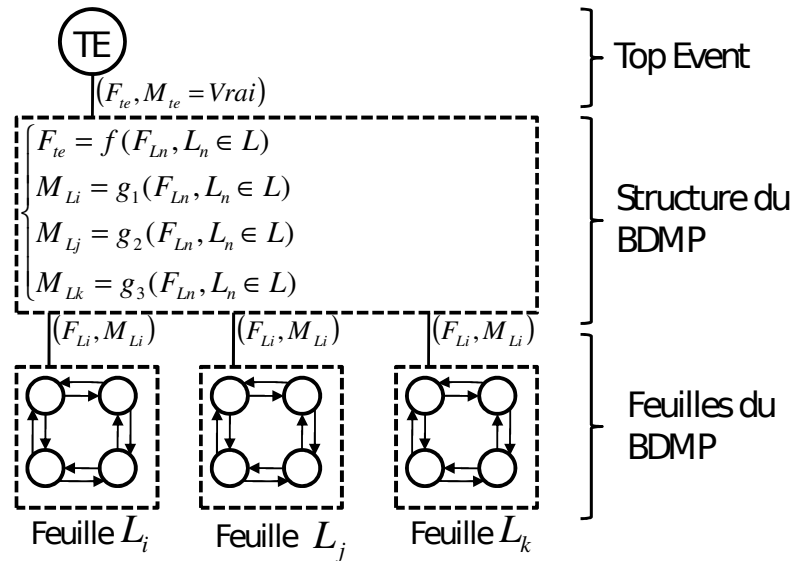
Figure 3.5 – Structure de la représentation d'un BDMP.
