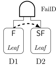
Figure 4.6 – Modèle BDMP des turbopompes
