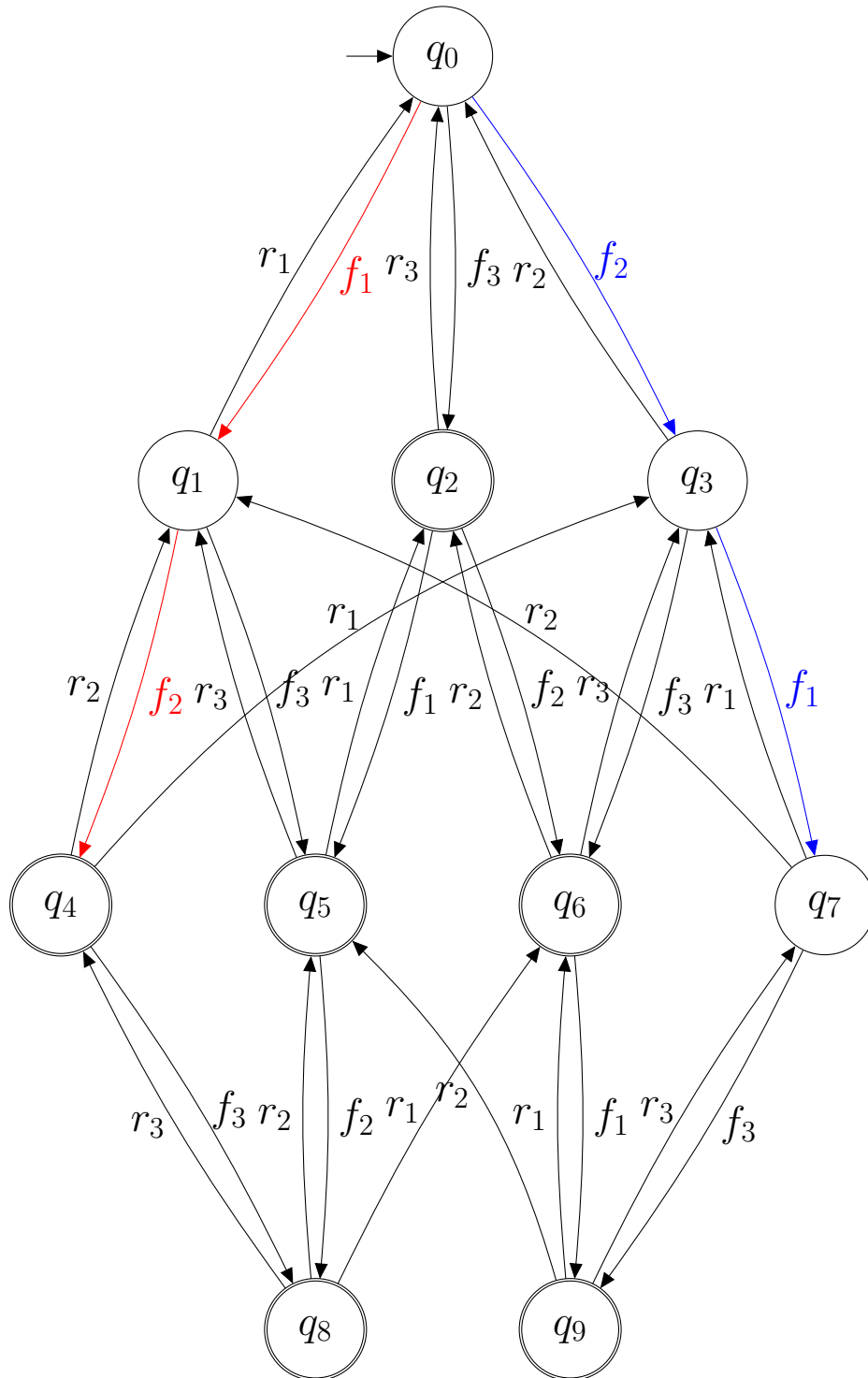
Figure 2.6 – Fonction de structure d'un système dynamique à 3 composants réparables sous forme d'automate.
