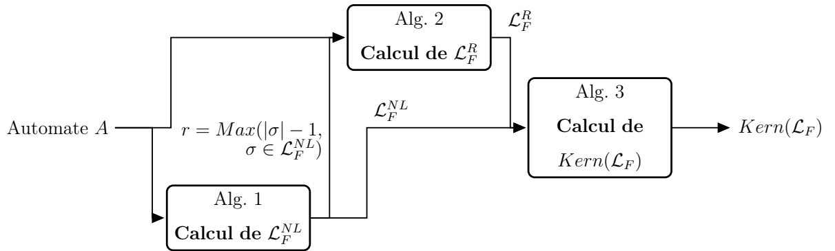
Figure 2.19 – Utilisation des algorithmes
