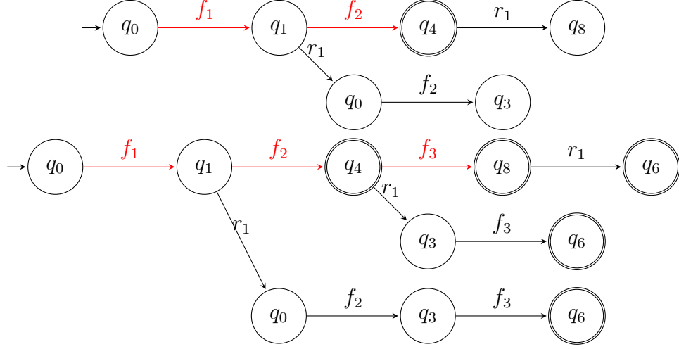
Figure 2.8 – Ajout d'un événement de réparation dans des séquences défaillantes.
