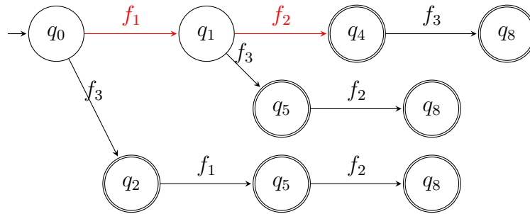
Figure 2.7 – Exemple d'automate fini représentant une fonction de structure dynamique.
