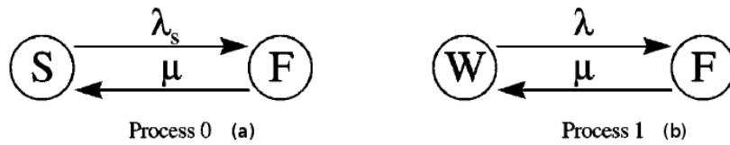
Figure 1.18 – Processus de Markov associés à une feuille SF possédant des taux de défaillance différents dans son mode dormant (a) et actif (b) [BB03].
