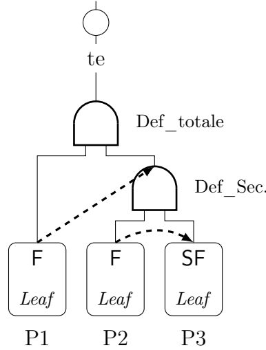
Figure 3.2 – Modèle BDMP du système à trois pompes
