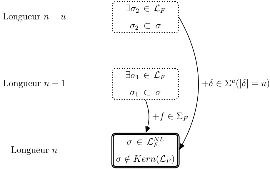
Figure 2.17 – Principe de calcul du noyau
