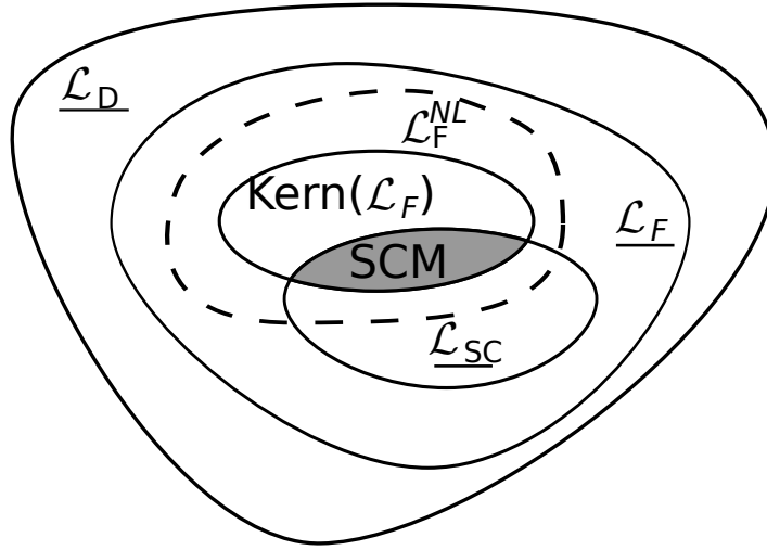
Figure 2.22 – Relations d'inclusion entre les différents langages et ensembles de séquences
