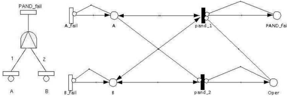
Figure 1.9 – Traduction d'une porte PAND en Well formed Stochastic Net [BR04]
