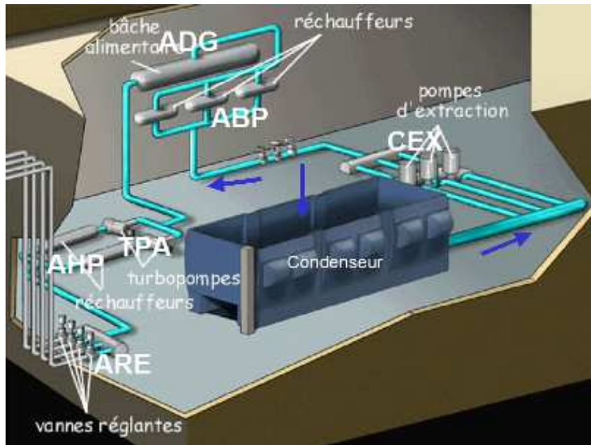
Figure 4.2 – Système Aval du condenseur.
