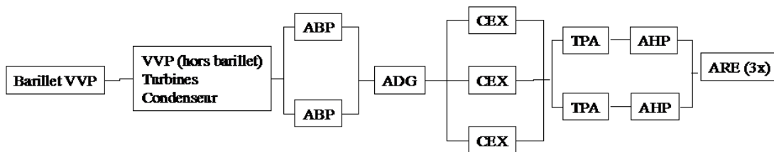
Figure 4.3 – Diagramme de fiabilité complet du système aval du condenseur.
