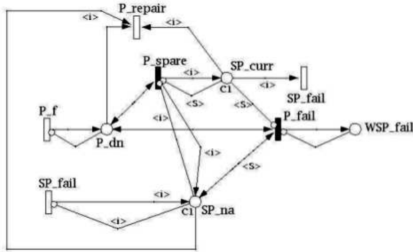
Figure 1.12 – Modèle RdP d'une porte WARM SPARE prenant en compte la réparabilité du composant principal [BR04]
