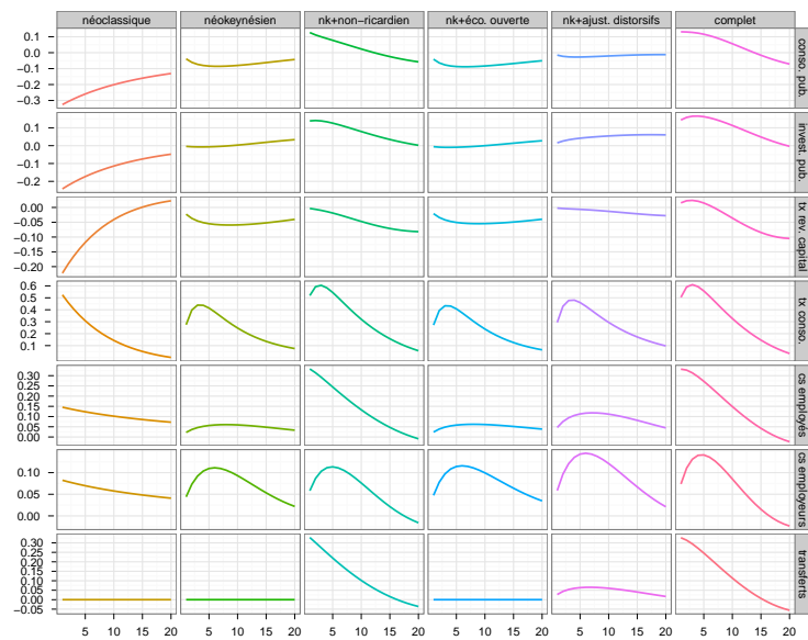
Graphique 2.13 – Réponses impulsionnelles de la consommation en fonction du modèle et du choc
