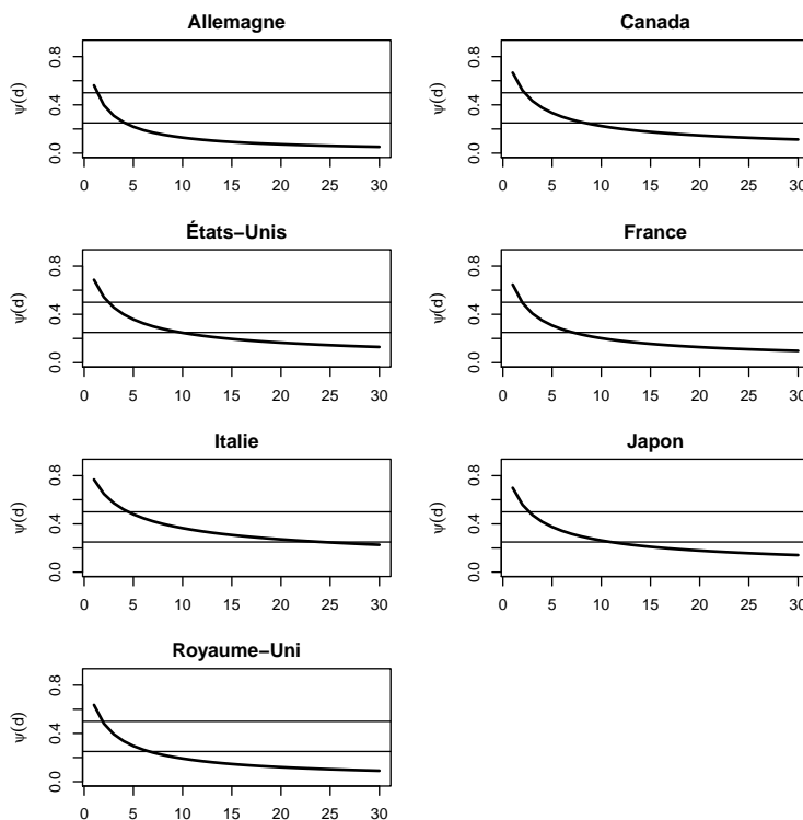
Graphique 1.5 – Réponses impulsionnelles des séries résiduelles I(d)
