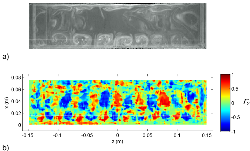
Figure 56 : Identification des instabilités centrifuges dans un plan horizontal situé à y/H = -0,3 pour L/H = 1,5 , S/H = 6 et Re_H = 2\,300 : a) visualisation, b) mesures PIV et critère G_2 .
