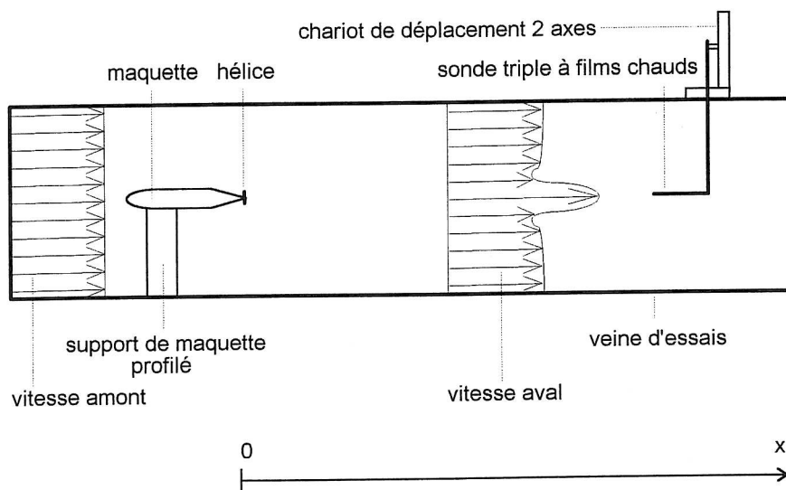
Fig. 1. – Dispositif expérimental.
