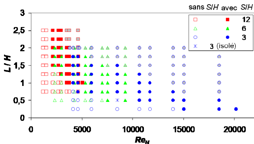
Figure 55 : Diagramme d'existence d'instabilités centrifuges en fonction du rapport L/H et du nombre de Reynolds Re_H pour S/H = 12, 6, \text{ et } 3 : symboles creux : absence, symboles pleins : présence, symboles gris : écoulement transitionnel et croix : instabilité isolée.
