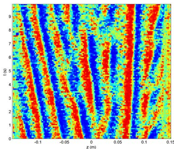
Figure 57 : Diagramme espace-temps du critère G_2 pour L/H = 1,5 , S/H = 6 et Re_H = 2\,300 .
