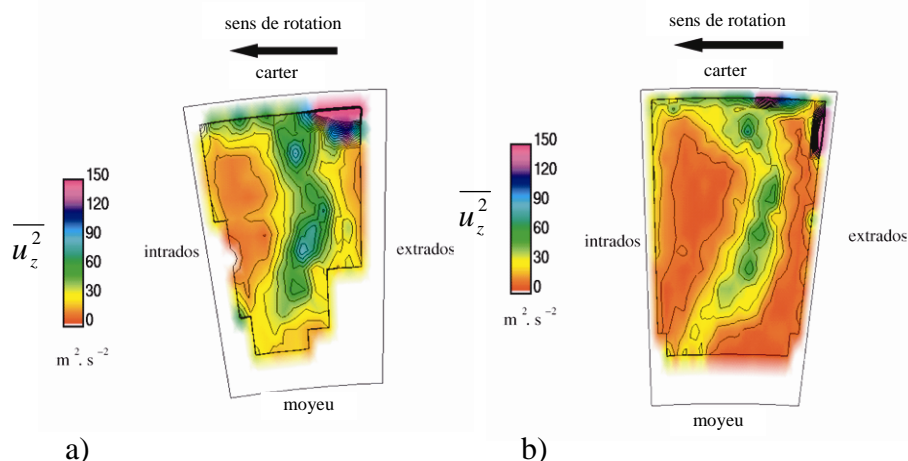
Figure 34 : Comparaison de la variance des fluctuations de vitesse axiale obtenue par a) une quadruple mesure sans filtre de coïncidence et b) une mesure avec filtre de coïncidence.
