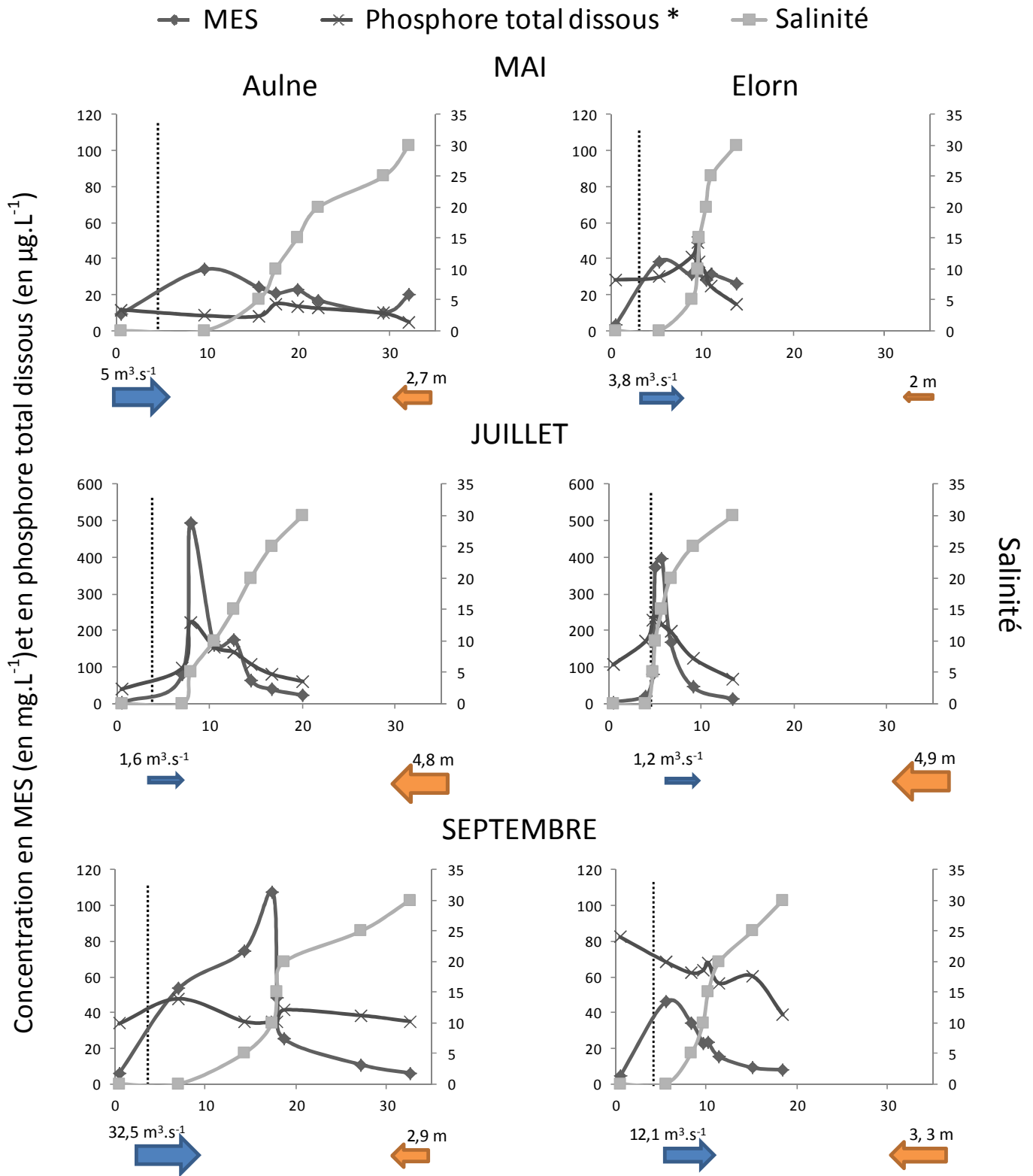
Fig.5 1 Variations spatiales et saisonnières de la salinité, et des concentrations en MES ( \text{mg} \cdot \text{L}^{-1} ) en Phosphore total dissous (en \mu\text{g} \cdot \text{L}^{-1} ) dans l'estuaire de l'Aulne (à gauche) et de l'Elorn (à droite). En juillet, le phosphore total (dissous + particulaire) est représenté (le phosphore total dissous n'a pas pu être dosé). Sur chaque graphique, le point situé à gauche du trait en pointillé représente la valeur du site en rivière pour chaque paramètre. Les flèches bleues représentent le débit des rivières, les flèches oranges le marnage de la marée.
