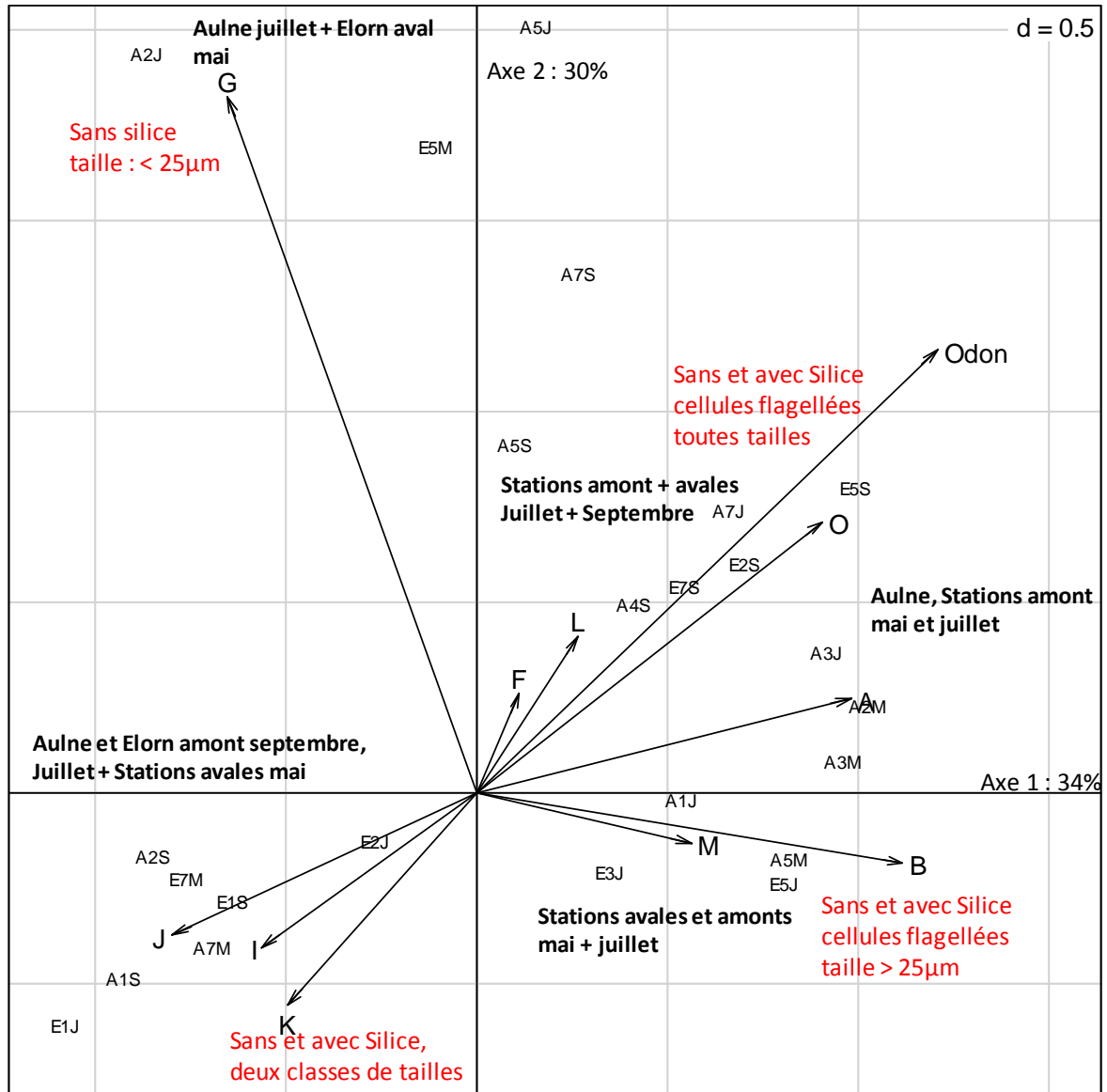
Fig.5 4 AFC réalisée à partir des biovolumes des groupes fonctionnels présents dans le long de l'estuaire de l'Aulne et de l'Elorn. Les deux premiers axes expliquent 64% de l'inertie totale. Une synthèse des groupes de sites (en noir) ainsi que les traits fonctionnels qui les caractérisent (en rouge) est représentée. Explication des codes : A pour Aulne, E pour Elorn, les chiffres de 1 à 7 rendent compte de la salinité (l'augmentation d'une unité correspond à une augmentation de 5 de salinité, 1 étant la salinité 0 et 7 la salinité 30), M pour Mai, J pour Juillet et S pour Septembre.
