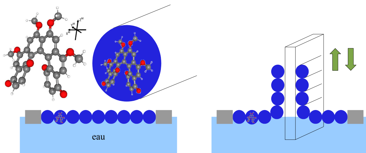
Figure II.3: Schéma de la structure des films de HBQ. A gauche, les molécules s'assemblent en couche de Langmuir pour former des fibres. A droite, le film dense de fibres est transféré sur substrat de verre par technique Langmuir-Blodgett. La molécule est représentée sans les chaînes alcanes C_{12}H_{25} latérales.
