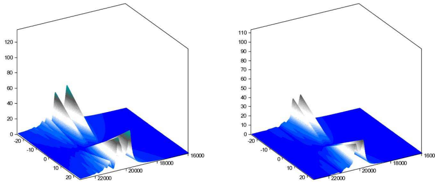
Figure III.8: Module de D^{\text{CT}} pour deux modes en couplage vibronique (à gauche, mode 1 à 500\text{cm}^{-1} ; à droite mode 2 à 800\text{cm}^{-1} ). Abscisses et échelles identiques à la Figure III.7.
