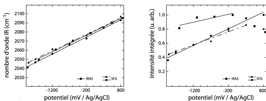
Figure I.7: Évolution comparée des paramètres de la résonance de CO sur Pt(110) en fonction du potentiel, obtenus en absorption infrarouge et en SFG, comme illustré sur la Figure I.6.
