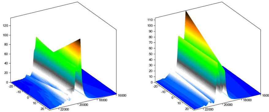
Figure III.7: Module de D_{1,2} pour deux modes en couplage vibronique (à gauche, mode 1 à 500\text{cm}^{-1} ; à droite mode 2 à 800\text{cm}^{-1} ). Abscisses : nombre d'onde ( \text{cm}^{-1} ) et angle de mélange (de -25^\circ à +25^\circ ).
