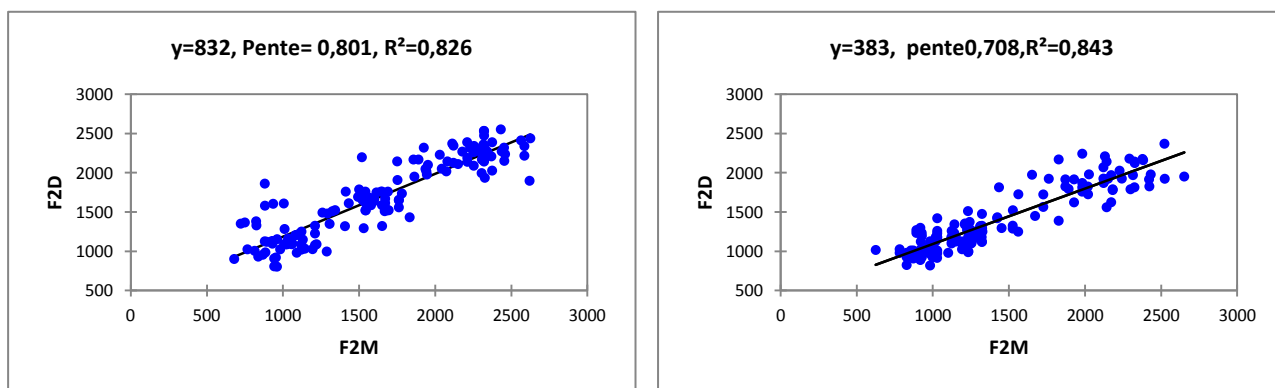
Figure 9 :L'équation de locus de la [s]à gauche et [sʰ] à droite, 10 locuteurs. [v3]
