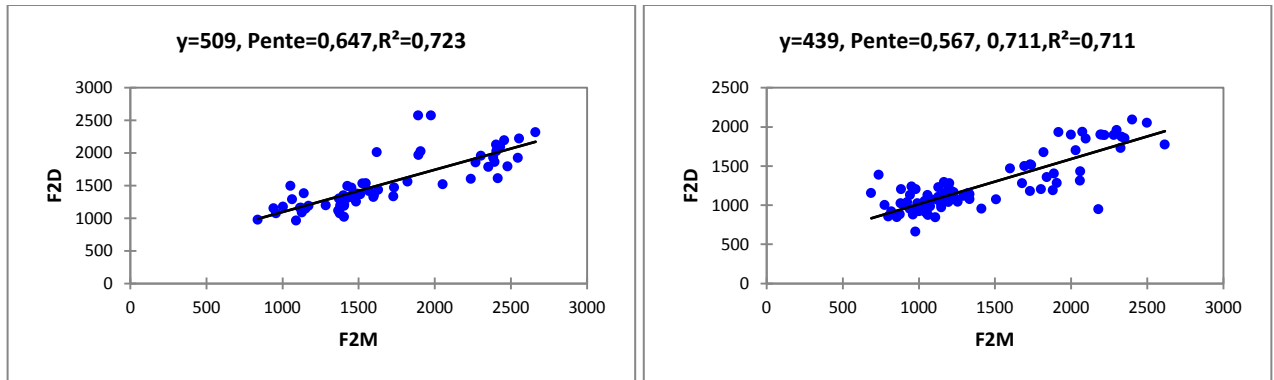
Figure 18 : Droit de régression de [tʰ] à gauche pour les femmes à droite pour les hommes [V 1 ]
