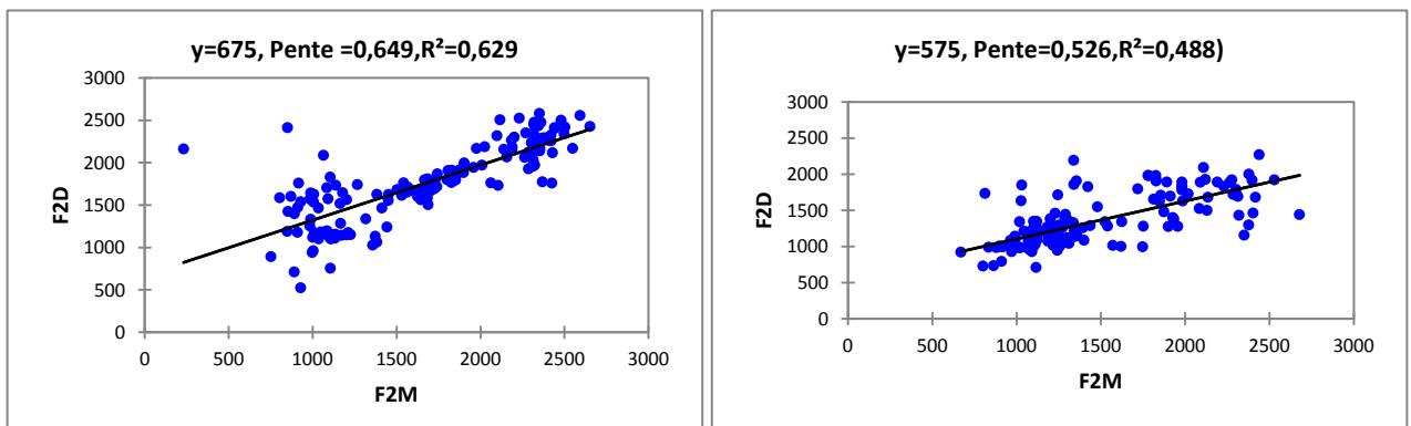
Figure 4 : L'équation de locus de la [d] à gauche et [dʰ] à droite, 10 locuteurs. [V1]
