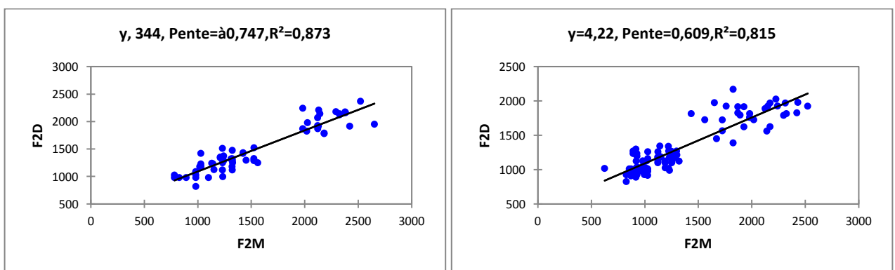
Figure 23 : Droit de régression de [s 6 ] à gauche pour les femmes à droite pour les hommes [V 3 ]
