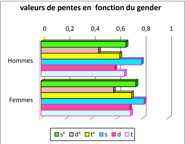
Figure 28 : Distribution des valeurs de pentes des consonnes pharyngalisées vs non pharyngalisées en fonction de sexe V3
