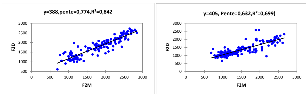
Figure 1 : L'équation de locus de la [t] à gauche et [tʰ] à droite, 10 locuteurs. [V1]
