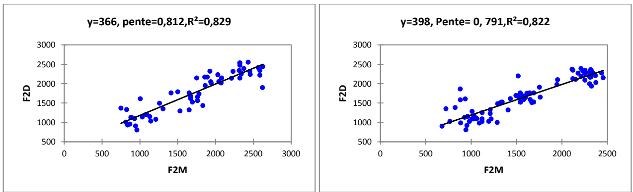
Droit de régression de [s] à gauche pour les femmes à droite pour les hommes [v3]
