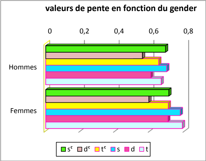
Figure 27 : Distribution des valeurs de pentes des consonnes pharyngalisées vs non pharyngalisées en fonction de sexe V2
