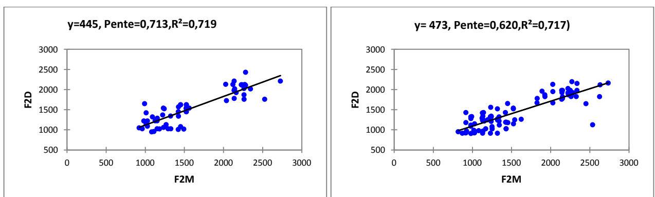
Figure 20 : Droit de régression de [tʰ] à gauche pour les femmes à droite pour les hommes [V 3 ]
