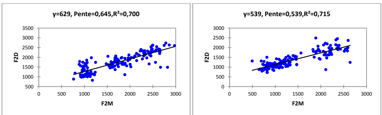
Figure 5 : L'équation de locus de la [d] à gauche et [dʰ] à droite, 10 locuteurs. [v2]
