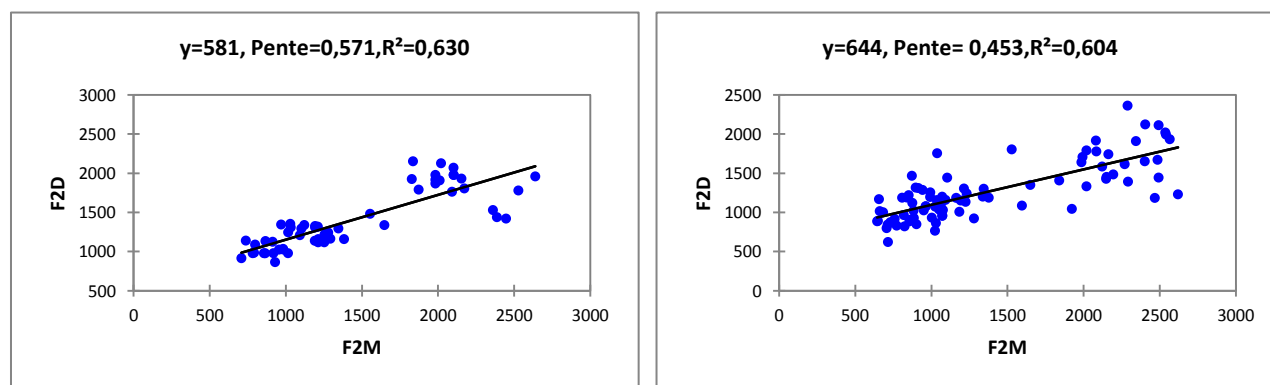
Figure 26 : Droit de régression de [d ɛ ] à gauche pour les femmes à droite pour les hommes [V 3 ]
