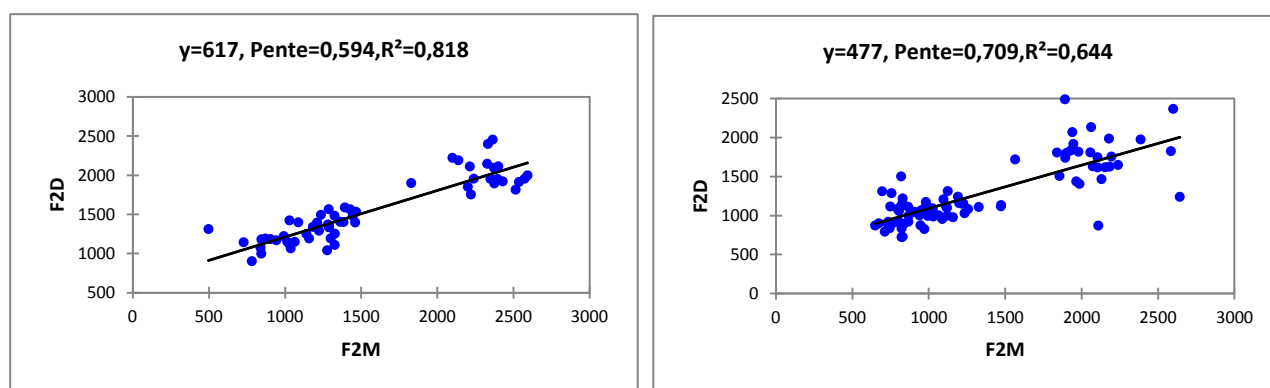
Figure 25 : Droit de régression de [d ɛ ] à gauche pour les femmes à droite pour les hommes [V 2 ]
