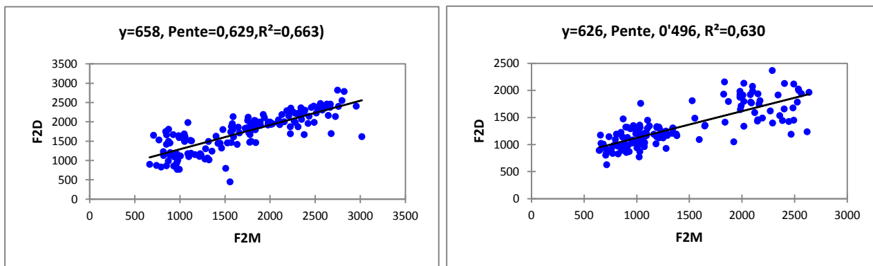
Figure 6 : L'équation de locus de la [d] à gauche et [dʰ] à droite, 10 locuteurs. [v3]
