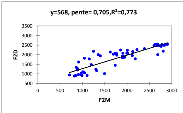
Figure 12 : Droit de régression de [t] à gauche pour les femmes à droite pour les hommes [v3]
