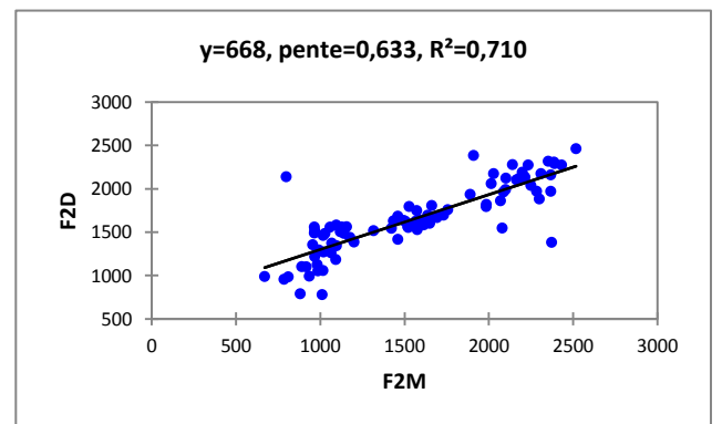
Figure 13 : Droit de régression de [s] à gauche pour les femmes à droite pour les hommes [V1]
