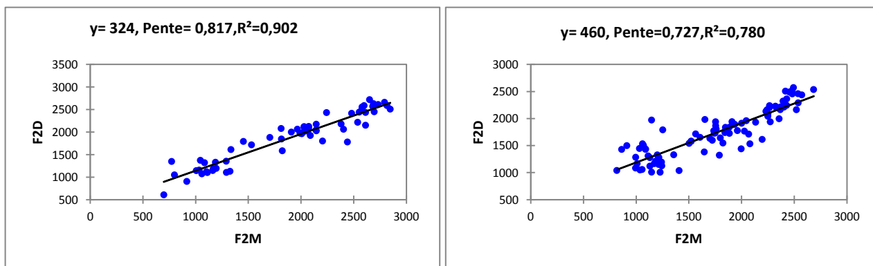
Figure 10 : Droit de régression de [t] à gauche pour les femmes à droite pour les hommes [V1]
