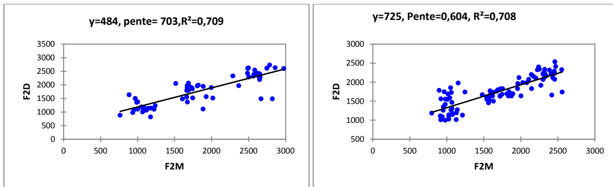
Figure 16 : Droit de régression de [d] à gauche pour les femmes à droite pour les hommes [v2]
