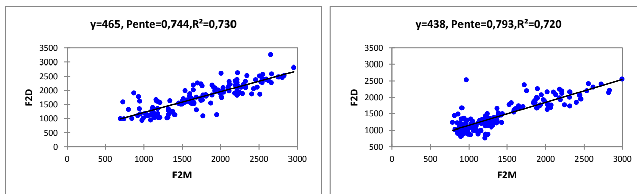
Figure 8 :L'équation de locus de la [s] à gauche et [sʰ] à droite, 10 locuteurs. [v2]
