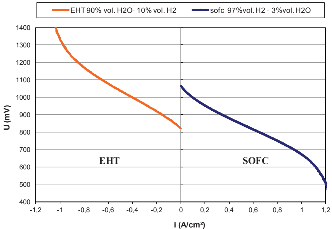
Figure III-3 : Courbe intensité-potentielle de la cellule CSC4 en EHT à 800°C sous 90% vol. H 2 O-10% vol. H 2 côté cathodique et 100% vol. air côté anodique, et en SOFC à 800°C sous 97% H 2 - 3% H 2 O côté cathodique et 400% vol. air côté anodique, débits d'entrée dans le compartiment H 2 =12 NmL/min/cm 2
