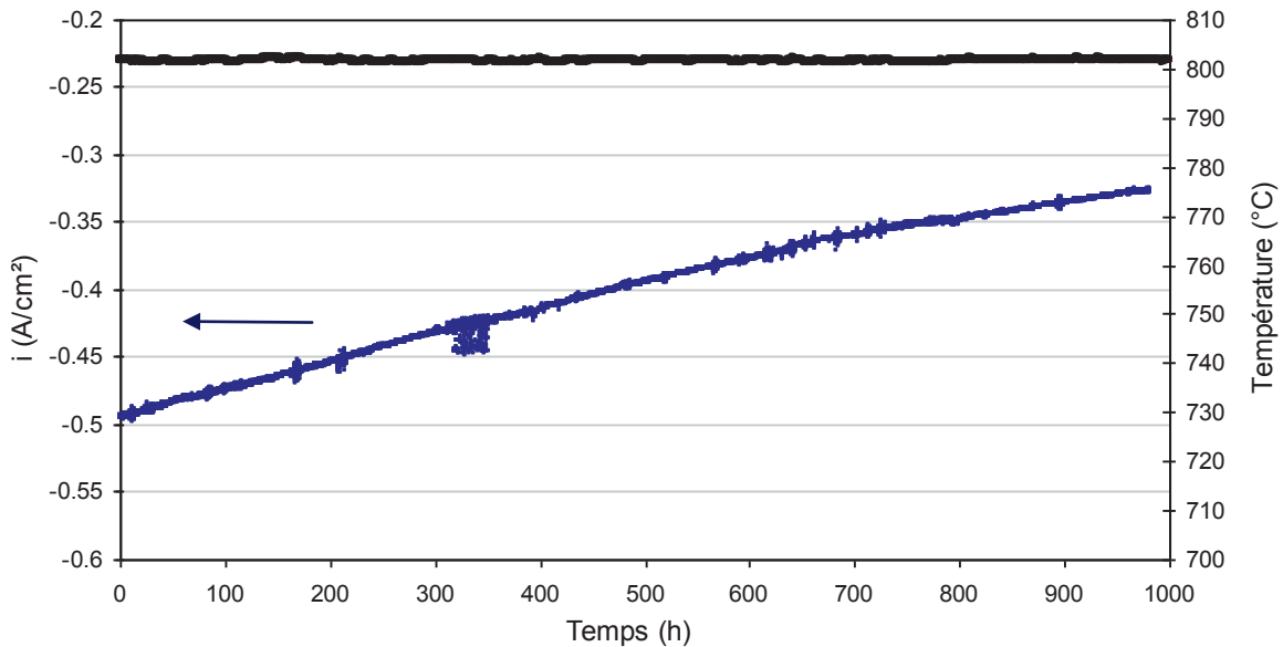
Figure V-4 : Evolution de l'intensité et de la température lors de l'étude en pilotage potentiostatique à U=1036 mV= U_{i=-0,5A/cm^2} à t=0 h à 800°C sous 90% vol. H 2 O-10% vol. H 2 côté cathodique, 100% vol. air côté anodique pendant 1000 heures
