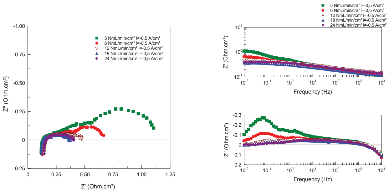
Figure IV-8 : Diagrammes d'impédances de la cellule CSC4 à i=-0,5 \text{ A/cm}^2 à 800^\circ\text{C} sous 90% vol. \text{H}_2\text{O} -10% vol. \text{H}_2 côté cathodique et 100% vol. air côté anodique à différents débits
