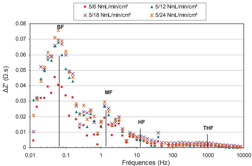
Figure IV-10: Le diagramme différentiel \partial Z'(f) / \partial \ln(f) = f(\text{fréquences}) de la CSC4 à différents débits à 800^\circ\text{C} , à i = -0,5 \text{ A/cm}^2 sous 90% vol. \text{H}_2\text{O} , 10% vol. \text{H}_2 côté cathodique et 100% vol. air côté anodique
