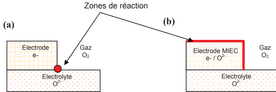
Figure II-1 : Représentation schématique des zones de contacts triples (a) dans le cas d'une électrode à O 2 conductrice purement électronique et (b) d'une électrode conductrice mixte MIEC
