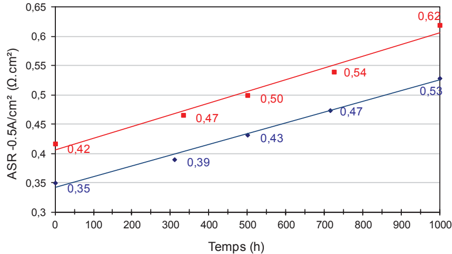
Figure V-10 : Evolution des ASRs mesurées à i=-0,5 A/cm 2 de deux cellules CSC4 fonctionnant à 800°C, sous 90% vol. H 2 O-10% vol. H 2 côté cathodique, 100% vol. air côté anodique pendant 1000 heures à i=-0,5 A/cm 2 , débits cathodique/anodique= 12 NmL/min/cm 2
