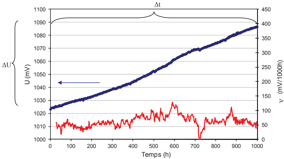
Figure III-12: Suivi de la tension et du taux de dégradation absolu instantané lors d'une étude en conditions stationnaires à i=-0.5A/cm^2 à 800^{\circ}C , 90% vol. H_2O -10% vol. H_2 côté cathodique, 100% Air côté anodique
