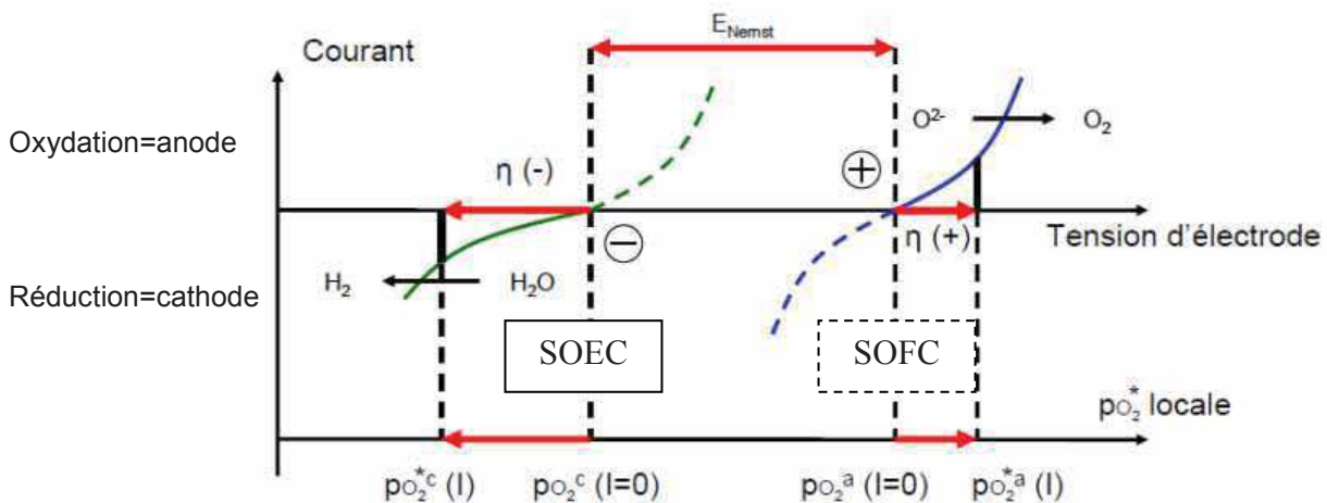
Figure I-7 : Représentation schématique des surtensions aux électrodes d'un électrolyseur [Guan2006]
