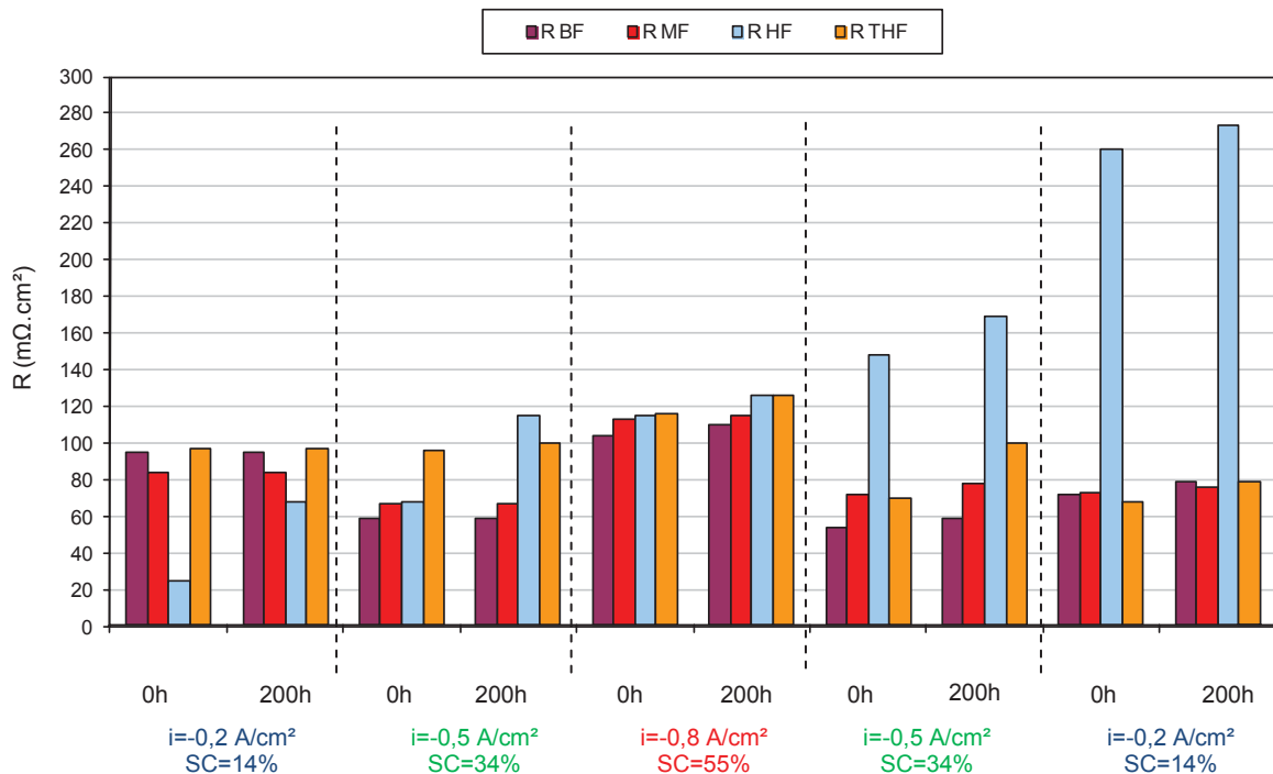
Figure V-36 : Evolution des résistances des quatre contributions lors de l'étude à 800°C sous 90% vol. H 2 O-10% vol. H 2 côté cathodique, 100% vol. air côté anodique, à débits d'entrée cathodique/anodique constants=12 NmL/min/cm 2
