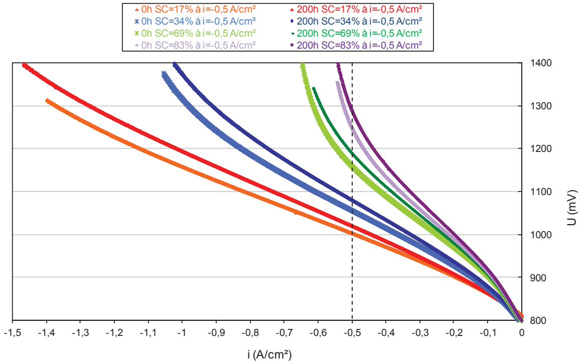
Figure V-15 : Evolution des courbes i - V au cours du temps lors de l'étude séquentielle de l'effet du taux de conversion à 800°C, à i=-0,5 A/cm 2 sous 90% vol. H 2 O-10% vol. H 2 côté cathodique, 100% vol. air côté anodique sur plusieurs paliers de 200 heures à différents débits cathodique/anodique; seulement un des trois paliers à SC=34% est représenté
