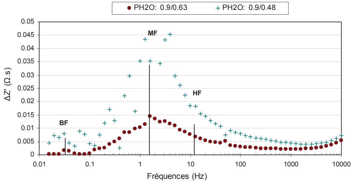
Figure IV-13: Le diagramme différentiel \partial Z'(f)/\partial \ln(f)=f(\text{fréquences}) de la CSC4 à différentes dilutions à 800°C sous 90% vol. H 2 O, 10% H 2 et 100% air, i=-0,5 \text{ A/cm}^2
