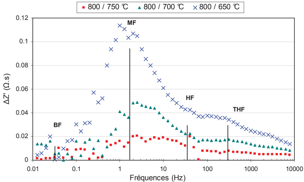
Figure IV-17: Diagramme différentiel \partial Z'(f) / \partial \ln(f) = f(\text{fréquences}) de la CSC4 à différentes températures sous 90% vol. H 2 O, 10% vol. H 2 côté cathodique et 100% vol. air côté anodique, à i=0 A/cm 2 , débits d'entrée cathodique/anodique=12 NmL/min/cm 2
