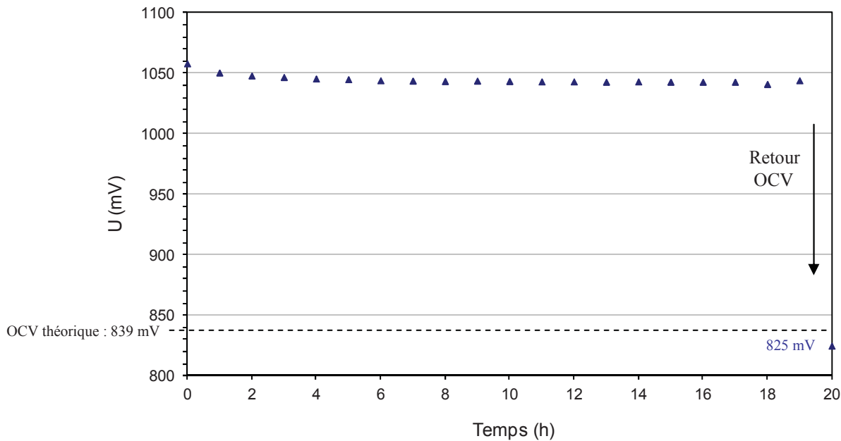
Figure III-7 : Suivi de la tension lors du conditionnement à 800°C, sous 90% vol. H 2 O-10% vol. H 2 côté cathodique, 100% air côté anodique à i = -0,6 \text{ A/cm}^2 , débits cathodique/anodique d'entrée=12 Nml/min/cm 2
