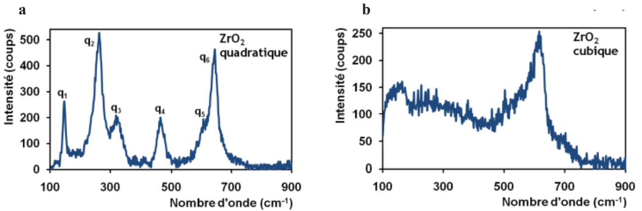
Figure V-52 : Spectres Raman acquis sur des échantillons de référence de a) zirconium quadratique et b) zirconium cubique
