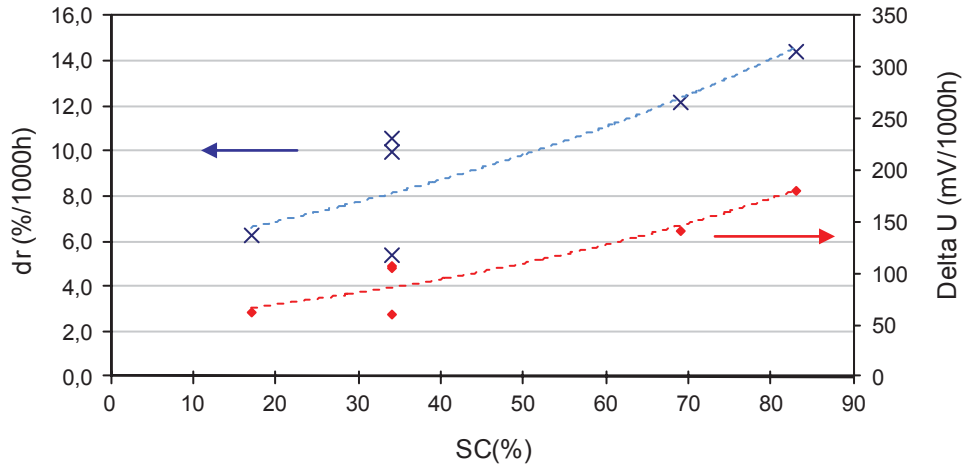
Figure V-14 : Evolution du taux de dégradation de la tension (croix bleues) et de l'augmentation de la tension (losange rouges) extrapolés à 1000 heures de fonctionnement pour chaque palier à i=-0,5 A/cm 2 en fonction du taux de conversion ; les trois paliers à 34% sont représentés
