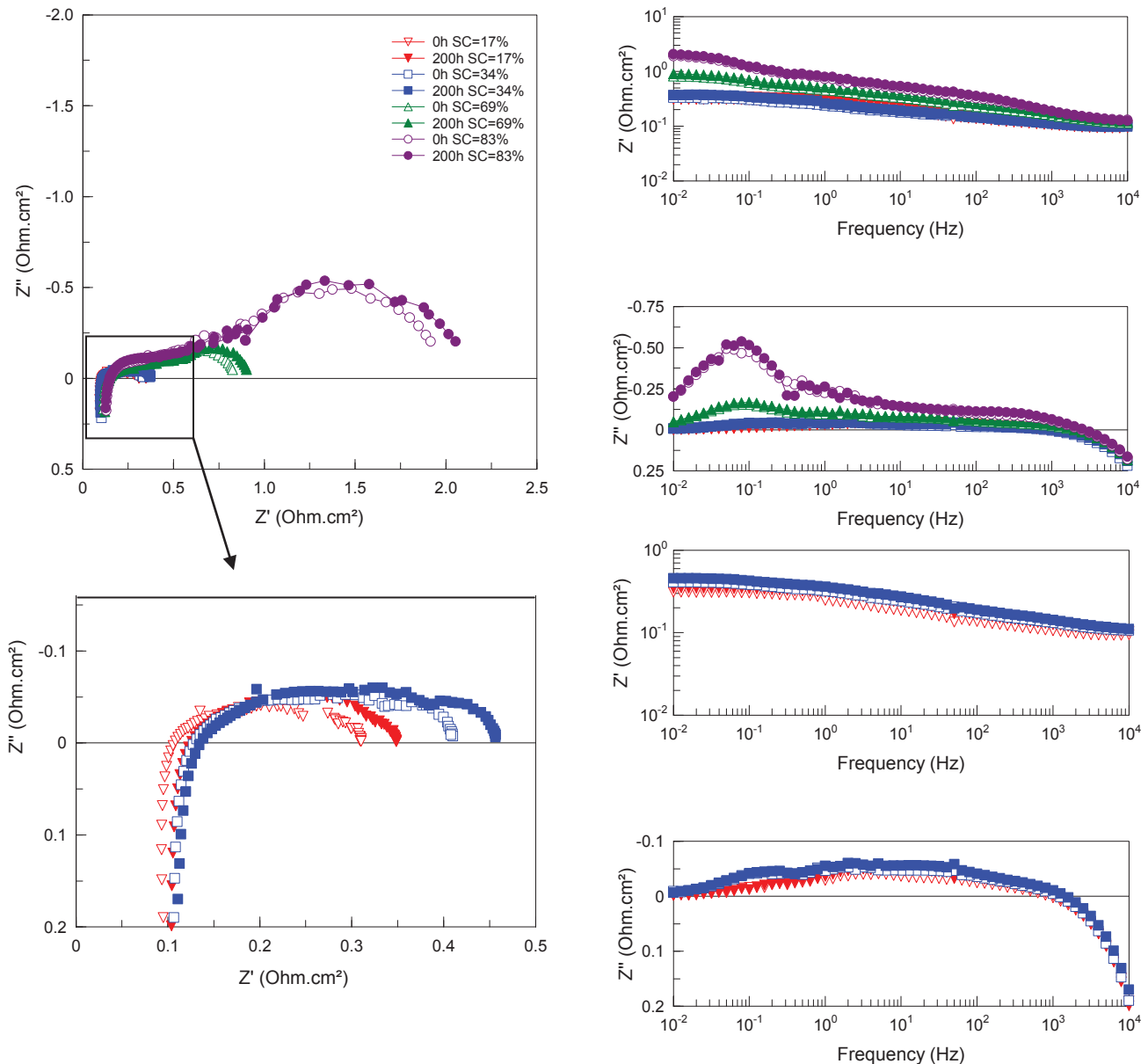
Figure V-18 : Diagrammes d'impédance mesurés en début et fin de chaque palier de 200 heures lors de l'étude séquentielle de l'effet du taux de conversion à 800°C, à i = -0.5 \text{ A/cm}^2 sous 90% vol. \text{H}_2\text{O} -10% vol. \text{H}_2 côté cathodique, 100% vol. air côté anodique; seulement un des trois paliers à SC=34% est représenté
