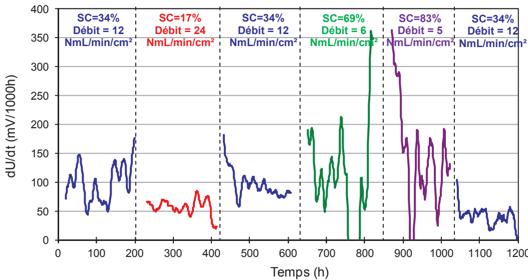
Figure V-13 : Evolution du taux de dégradation instantané au cours du temps lors de l'étude séquentielle de l'effet du taux de conversion à 800°C, à i=-0.5 \text{ A/cm}^2 sous 90% vol. \text{H}_2\text{O} -10% vol. \text{H}_2 côté cathodique, 100% vol. air côté anodique sur plusieurs paliers de 200 heures à différents débits cathodique/anodique
