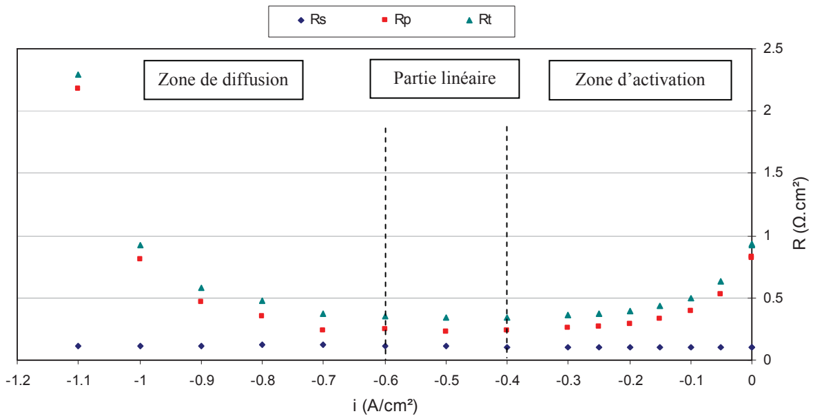
Figure IV-6 : Evolution des résistances série R s , de polarisation R p et totale R t aux différentes densités de courant à 800°C sous 90% vol. H 2 O-10% vol. H 2 côté cathodique et 100% vol. air côté anodique, débits cathodique/anodique=12 NmL/min/cm 2
