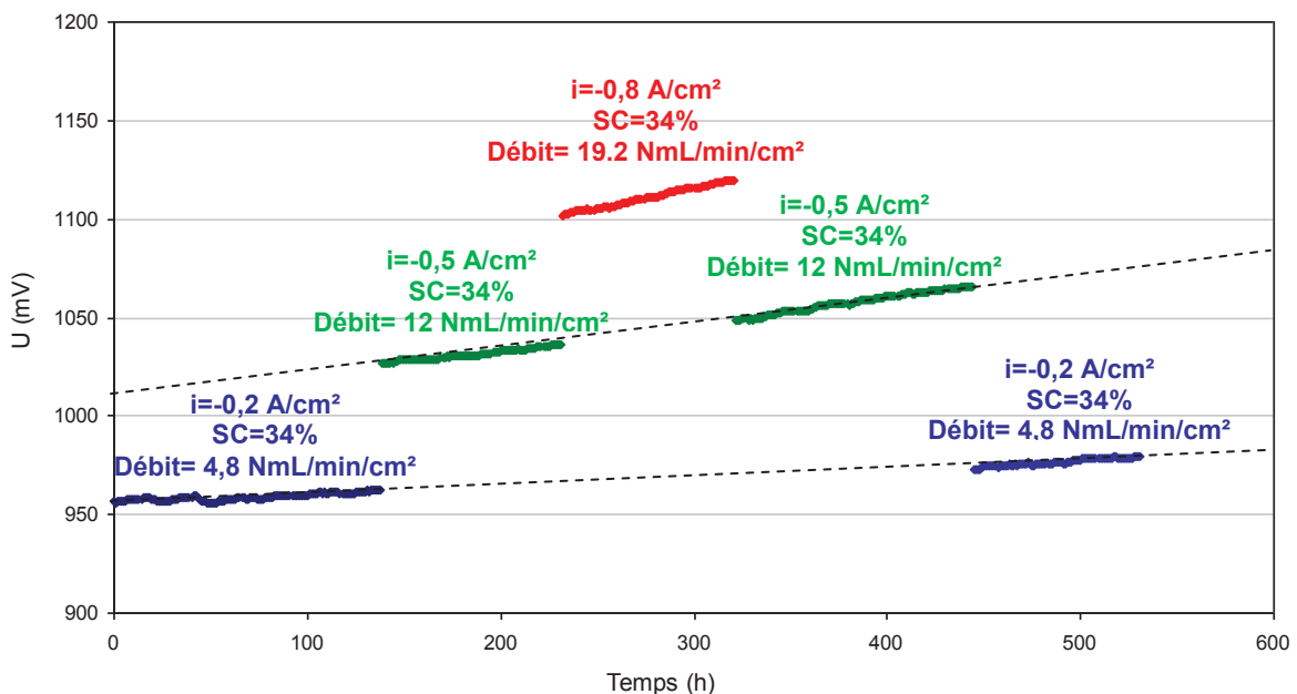
Figure V-22 : Suivi temporel de la tension lors de l'étude séquentielle de l'effet de la densité de courant à SC=34% à 800°C, sous 90% vol. H 2 O-10% vol. H 2 côté cathodique, 100% vol. air côté anodique
