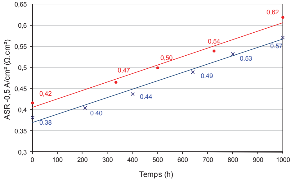
Figure V-8 : Evolution des ASRs calculées à i=-0,5 A/cm 2 de l'essai en pilotage galvanostatique (ronds rouges) et de celles issues de l'étude en pilotage potentiostatique calculées à l'aide des courbes i-V à i=-0,5 A/cm 2 (croix bleues).
