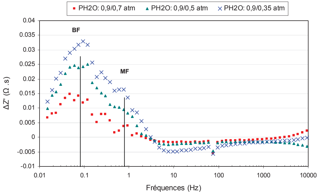
Figure IV-21: Le diagramme différentiel \partial Z'(f) / \partial \ln(f) = f(\text{fréquences}) de la CSC4 à différentes compositions des gaz cathodiques d'entrée à 800°C sous 90% vol. H 2 O, 10% vol. H 2 + N 2 côté cathodique et 100% vol. air côté anodique, à i = -0,5 \text{ A/cm}^2
