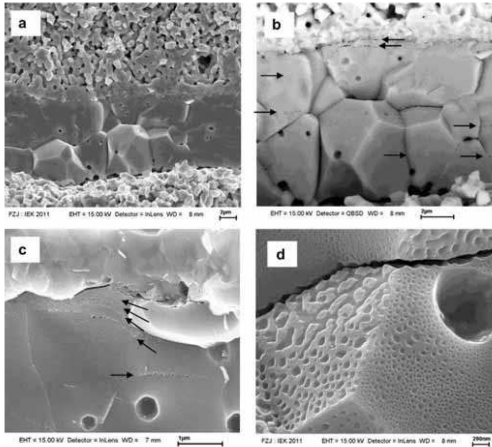
Figure II-10 : Micrographies MEB à différentes échelles de l'électrolyte 8YSZ après 9000h de fonctionnement en EHT à i=-1 A/cm 2 (SC=36%) à 778°C sous 90 NL.h -1 d'air synthétique côté anodique et 6 NL.h -1 d'H 2 - 7,08 NL.h -1 de N 2 - 42 NL.h -1 d'H 2 O côté cathodique [Tietz2013]
