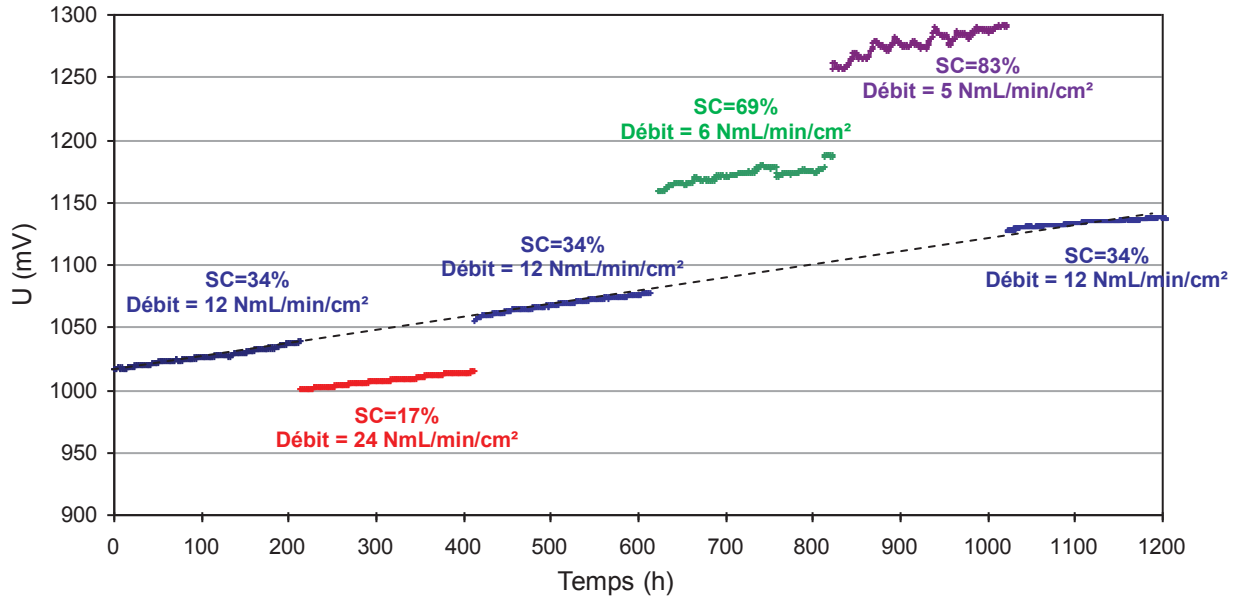
Figure V-12 : Evolution de la tension au cours du temps lors de l'étude séquentielle de l'effet du taux de conversion à 800°C, à i=-0.5 \text{ A/cm}^2 sous 90% vol. \text{H}_2\text{O} -10% vol. \text{H}_2 côté cathodique, 100% vol. air côté anodique sur plusieurs paliers de 200 heures à différents débits cathodique/anodique
