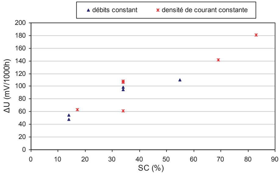
Figure V-41 : Vitesses de dégradation de la tension en fonction du taux de conversion suivant les conditions de fonctionnement choisies : débit cathodique d'entrée ou densité de courant constants
