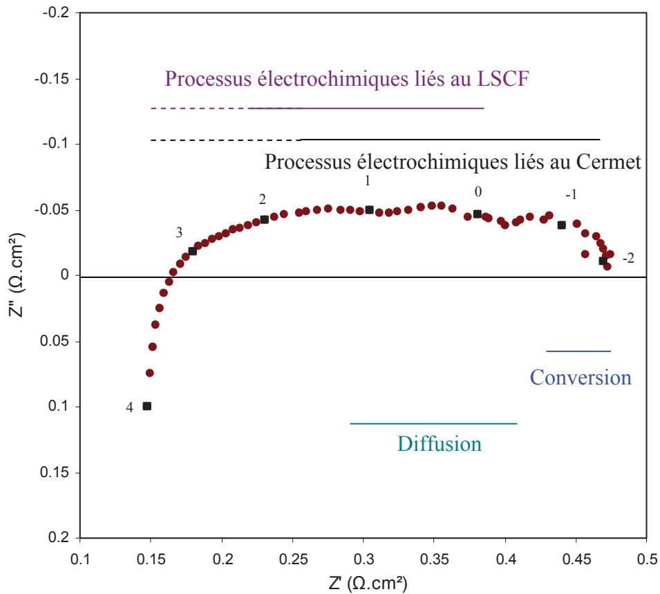
Figure IV-22 : Décomposition et identification des différents phénomènes se déroulant au sein de la cellule CSC4 à 800°C sous 90% vol. \text{H}_2\text{O} -10% vol. \text{H}_2 , 100% Air, à i = -0,5 \text{ A/cm}^2
