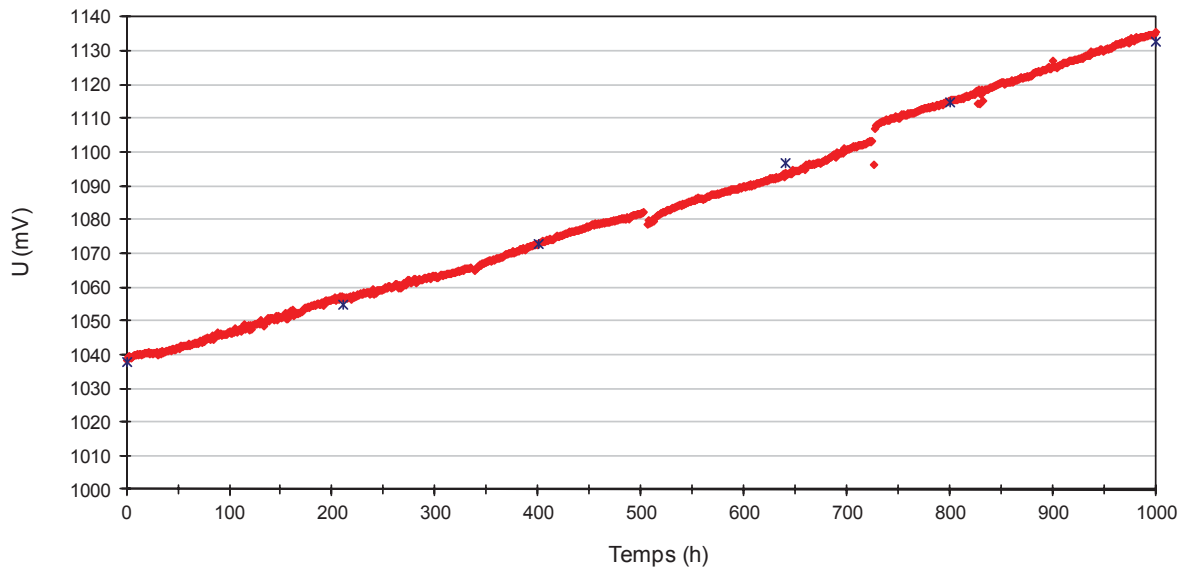
Figure V-7 : Evolution de la tension de l'essai en pilotage galvanostatique (rouge) et de celle issue de l'étude en pilotage potentiostatique relevée à l'aide des courbes i - V à i=-0,5 \text{ A/cm}^2 (croix bleues). Etudes de 1000 heures à 800^\circ\text{C} sous 90% vol. \text{H}_2\text{O} -10% vol. \text{H}_2 côté cathodique, 100% vol. air côté anodique, débits cathodique/anodique=12 NmL/min/cm 2
