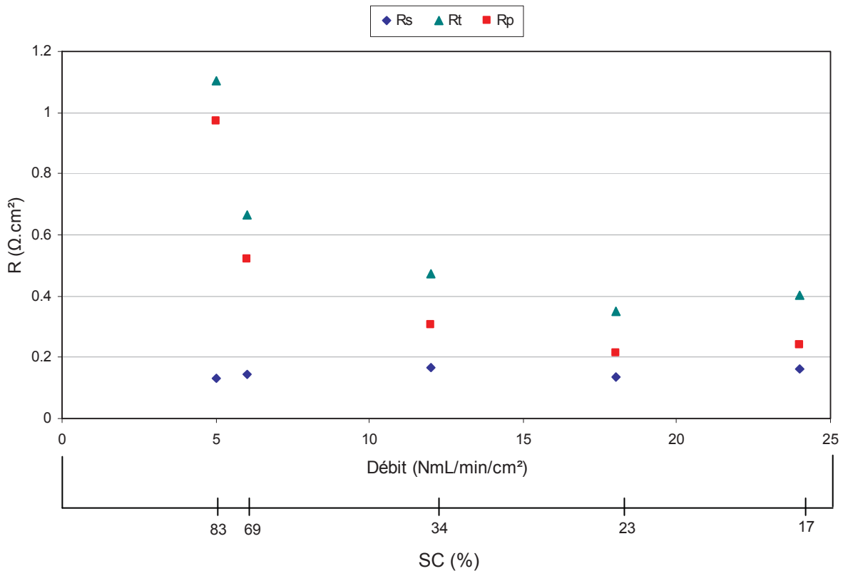
Figure IV-9 : Suivi des résistances série R_s , de polarisation R_p et totale R_t de la CSC4 pour différents débits cathodiques d'entrée à 800^\circ\text{C} à i=-0,5 \text{ A/cm}^2 sous 90% vol. \text{H}_2\text{O} -10% vol. \text{H}_2 côté cathodique et 100% vol. air côté anodique
