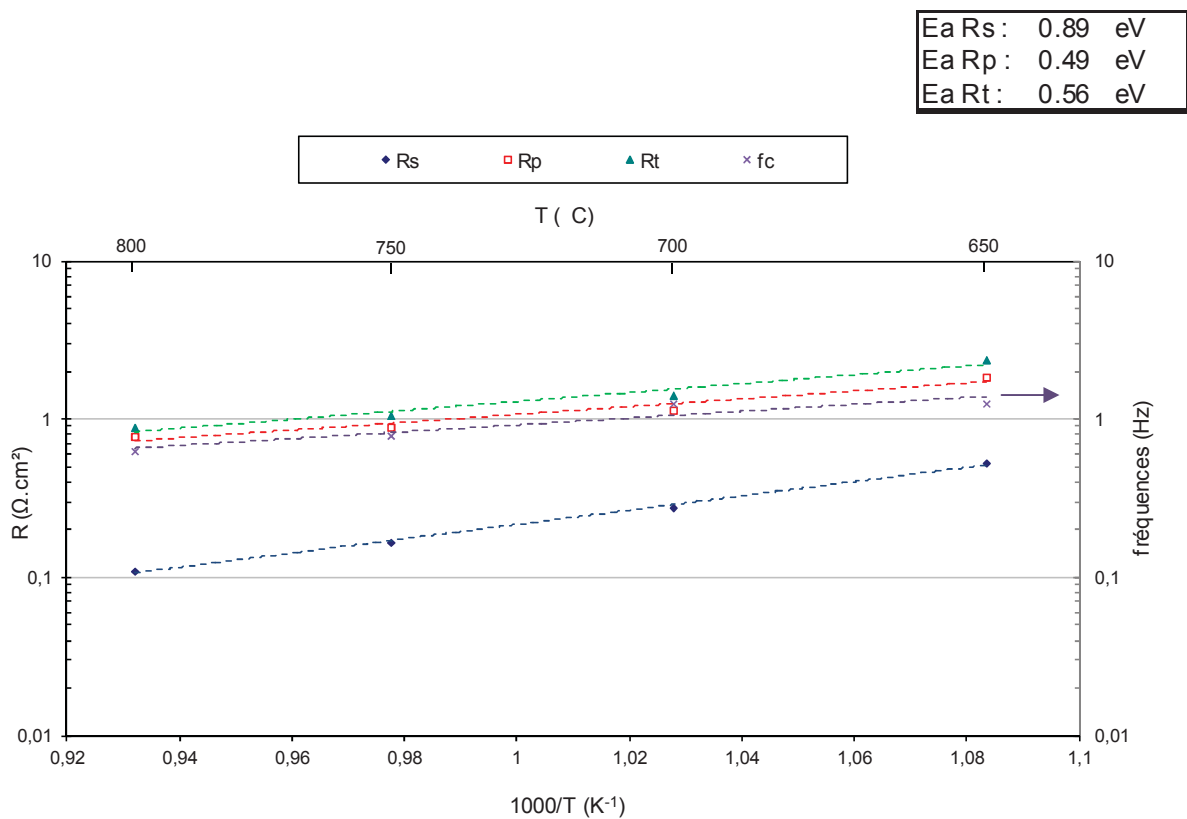
Figure IV-16 : Evolution des résistances de série R_s , de polarisation R_p et totale R_t et des fréquences caractéristiques en fonction de la température à i=0 A/cm 2 sous 90% vol. H 2 O-10% vol. H 2 , 100% vol. Air, débits d'entrée cathodique/anodique=12 NmL/min/cm 2
