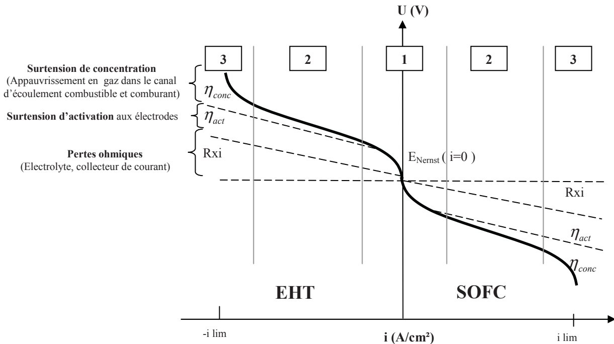
Figure I-8 : Décomposition d'une courbe intensité-potential ( i - V ) en mode EHT et SOFC (convention adoptée : i < 0 en EHT et i > 0 en SOFC)
