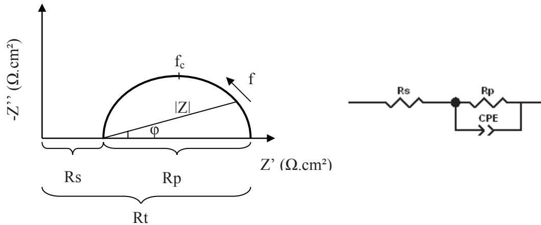
Figure III-11 : Circuit électrique équivalent à un demi-cercle dans le plan de Nyquist
