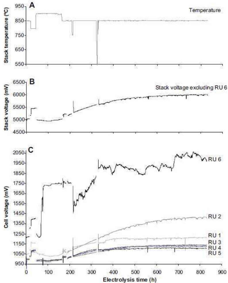
Figure II-23 : Evolution a) de la température b) de la tension aux bornes du stack et c) aux bornes de chaque cellule lors du fonctionnement du stack 6 cellules à électrodes support à 850°C à -0,25 \text{ A/cm}^2 sous 50% vol. \text{H}_2\text{O} -50% \text{H}_2 côté cathodique et de l'oxygène pour le côté anodique [Ebbesen2011]
