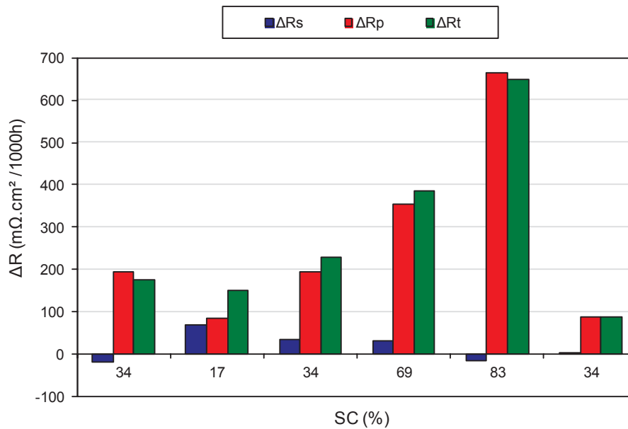
Figure V-19 : Evolution des résistances totale, de polarisation et série au cours du temps en fonction du taux de conversion, mesurées à i=-0.5\text{A/cm}^2 lors de l'étude séquentielle de l'effet du taux de conversion à 800^\circ\text{C} , à i=-0.5\text{ A/cm}^2 sous 90% vol. \text{H}_2\text{O} -10% vol. \text{H}_2 côté cathodique, 100% vol. air côté anodique
