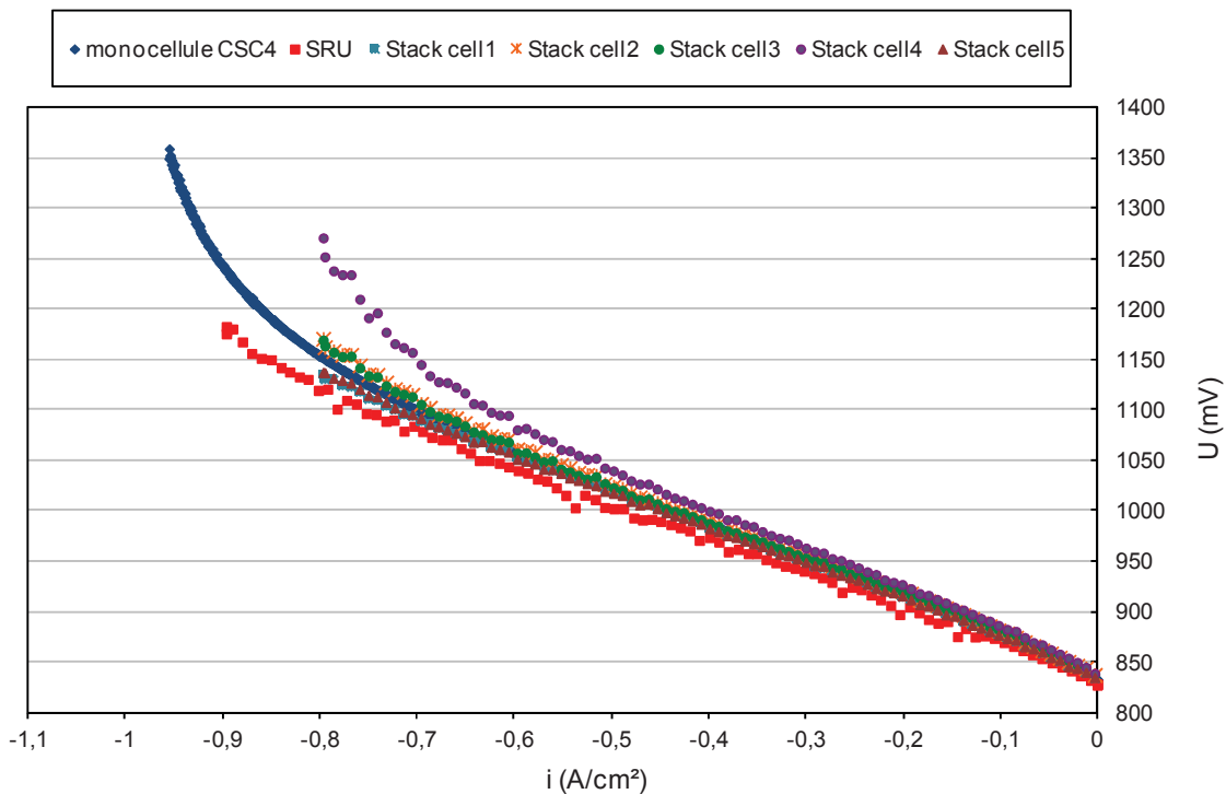
Figure VI-3 Caractéristiques i-V de la monocellule, du SRU et des 5 cellules de l'empilement stack, à 800 °C sous 90 % vol. \text{H}_2\text{O} + 10 % vol. \text{H}_2 côté cathodique, 100 % vol. air côté anodique, SC=55% à -0,8 \text{ A/cm}^2 [Petitjean2011]
