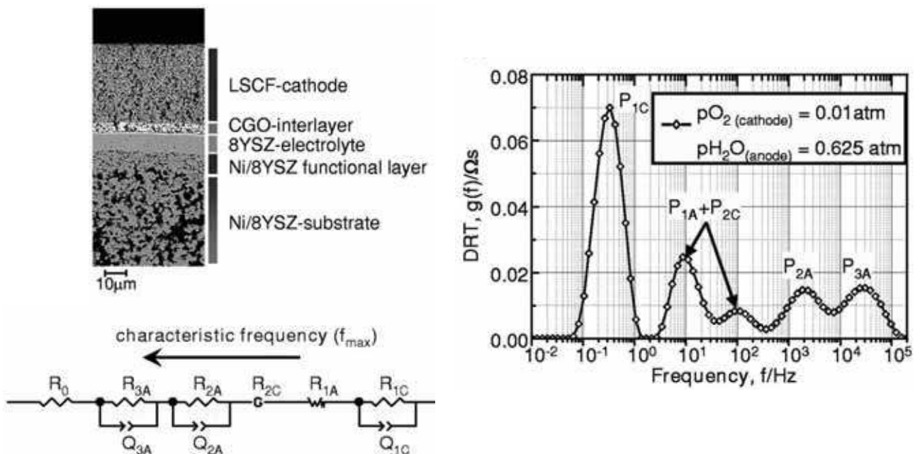
Figure IV-1 : Circuit électrique équivalent et représentation par la méthode DRT de la réponse de la cellule à électrode support LSCF/CGO/8YSZ/Ni-8YSZ en mode SOFC à T=800^{\circ}C , sous P_{H_2O}=0,625 atm. et P_{O_2}=0,01 atm. à i_{dc}=0A [Leonide2008]
