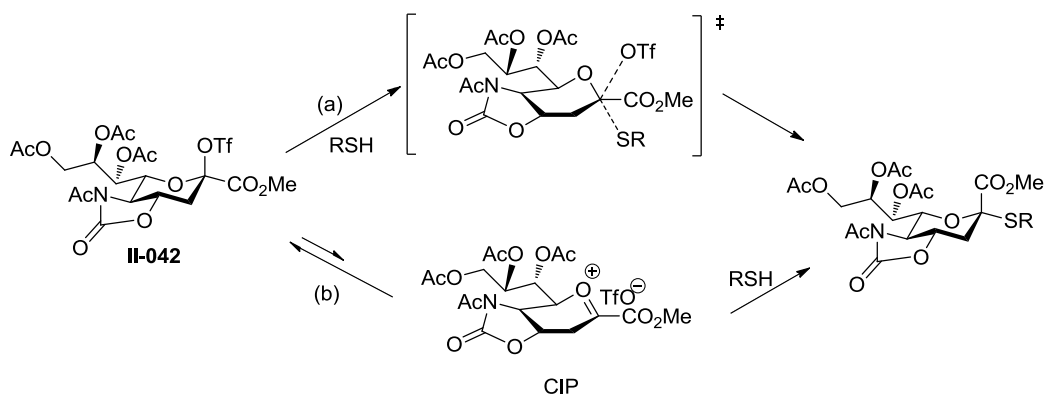
Schéma 158 : propositions de mécanisme associatif (a) ou dissociatif (b) pour les S-glycosylations.
