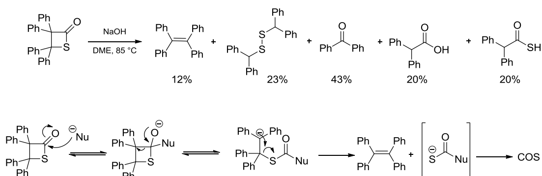
Schéma 22 : schéma réactionnel et mécanisme d'obtention d'alcène à partir de la tétraphényl-β-thiolactone en présence de soude.
