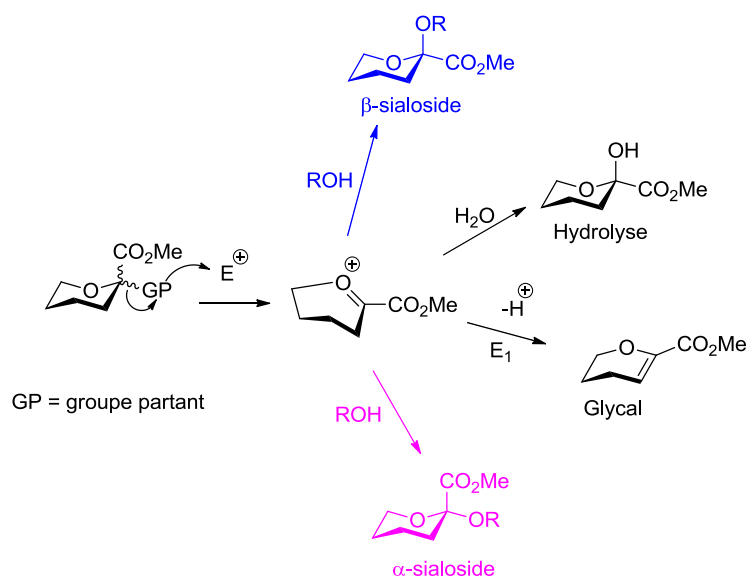
Schéma 108 : mécanisme général des réactions de sialylation.
