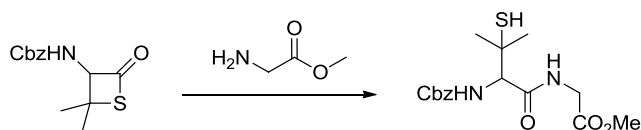
Schéma 54 : formation de liaison peptidique par ouverture de \beta -thiolactone.
