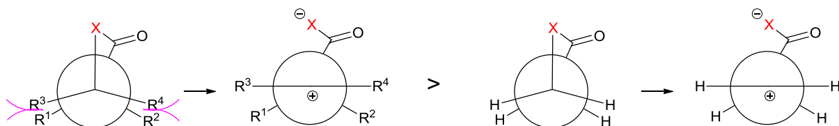
Schéma 51 : décompression stérique lors de l'extrusion de COX à partir d'une β-(thio)lactone.
