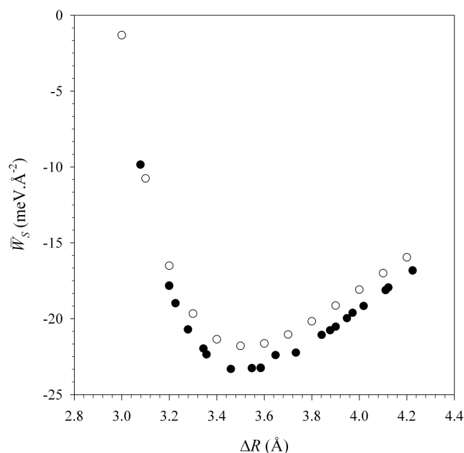
FIGURE 5.4 – Comportement de \bar{W}_S en fonction de \Delta R en utilisant le modèle discret (cercles noirs) et le modèle continu (cercles blancs).
