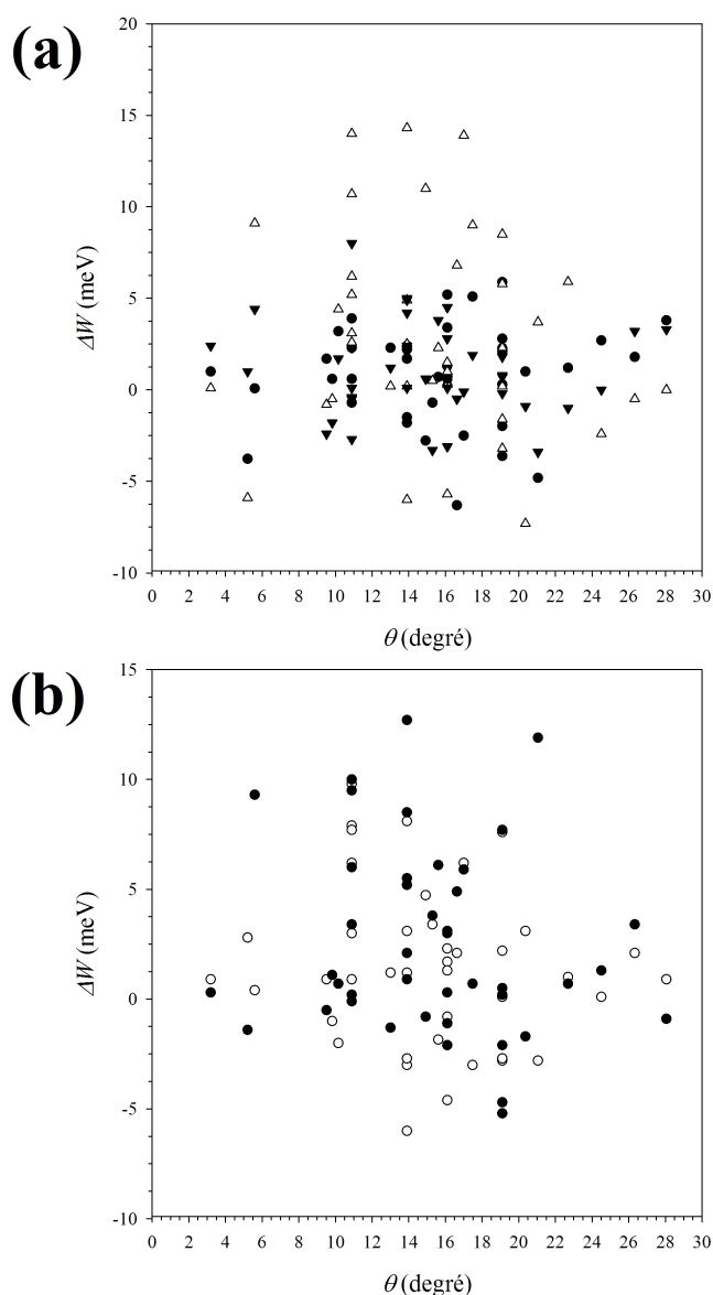
FIGURE 3.13 – Différence chirale d'énergie d'adsorption \Delta W en fonction de l'angle chirale \theta du nanotube lors de l'adsorption de (a) l'alanine (triangles noirs), de l'acide aspartique (cercles noirs) ou de l'acide glutamique (triangles blancs) ou de (b) la thréonine (2L,3L) (cercles blancs) ou de la thréonine (2R,3L) (cercles noirs).
