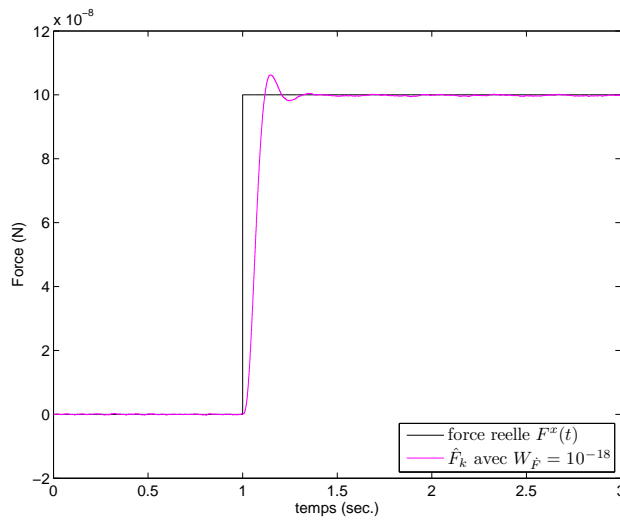
(a) Force réelle et estimée avec W_{\hat{F}} = 10^{-18} \text{ N}^2/\text{Hz} .
