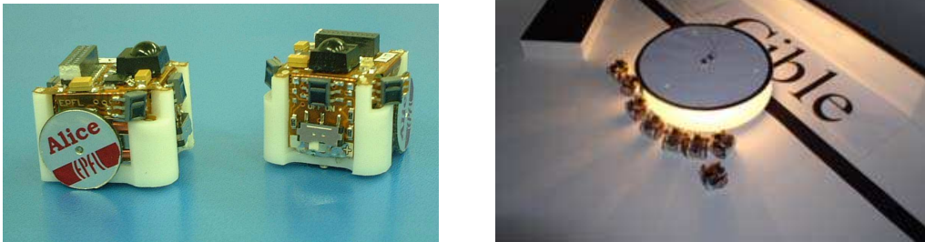
FIGURE 1.2 – Minirobots à roues Alice [13] travaillant en coopération pour pousser un objet vers une cible [4].
