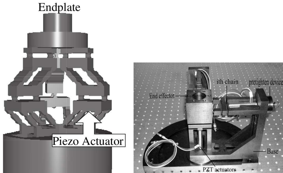
FIGURE 1.14 – Positionneurs tridimensionnels.
