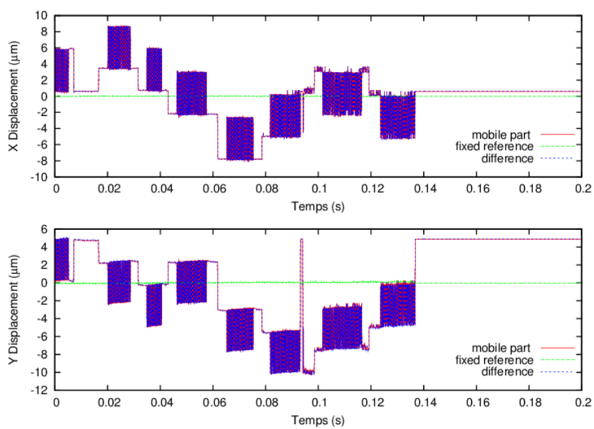
FIGURE C.3 – Résultats du MEMS Analyser lors de la mesure de l'espace de travail complet atteignable.
