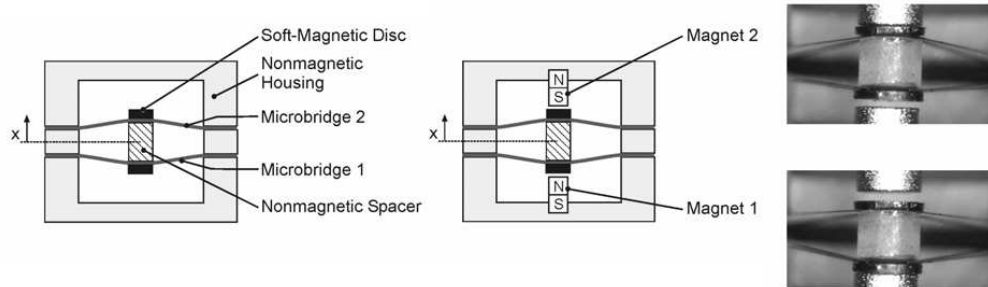
FIGURE 2.22 – Microsysteme binaire alliant actionneurs en alliage à mémoire de forme et aimants permanents [5].
