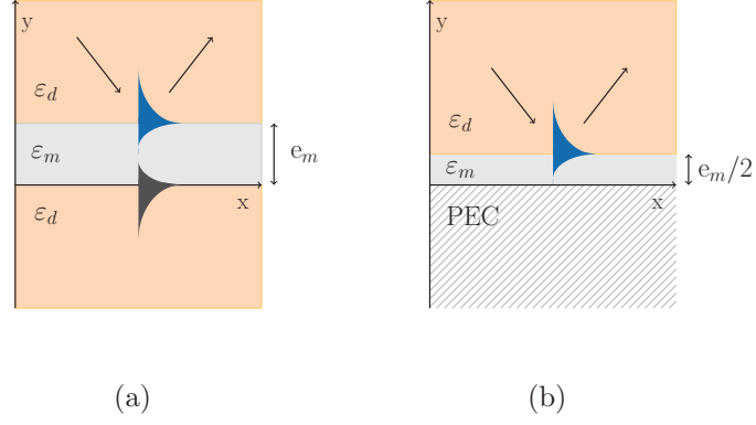
Figure B.3: (a) Film métallique ( \varepsilon_m ) d'épaisseur e_m dans un milieu diélectrique ( \varepsilon_d ) symétrique. (b) Film métallique ( \varepsilon_m ) d'épaisseur e_m/2 déposé sur un milieu infiniment conducteur dans un milieu diélectrique ( \varepsilon_d ).
