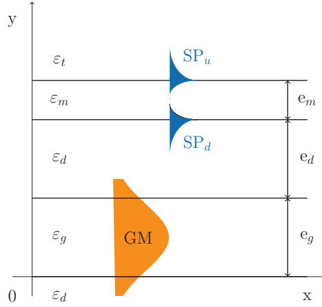
Figure B.7: Structure guidante plane qui permet le couplage fort entre le plasmon de surface SP_d et le mode guidé GM . Les permittivités diélectriques de chaque couche sont \varepsilon_d = 2.1025 , \varepsilon_g = 4.84 , \varepsilon_t = 3 , et \varepsilon_m . Les épaisseurs du coeur du guide est e_g et du film métallique est e_m sont fixées. Seule l'épaisseur e_d , la distance entre les deux modes couplés, est modifiée pour obtenir le régime de couplage fort.
