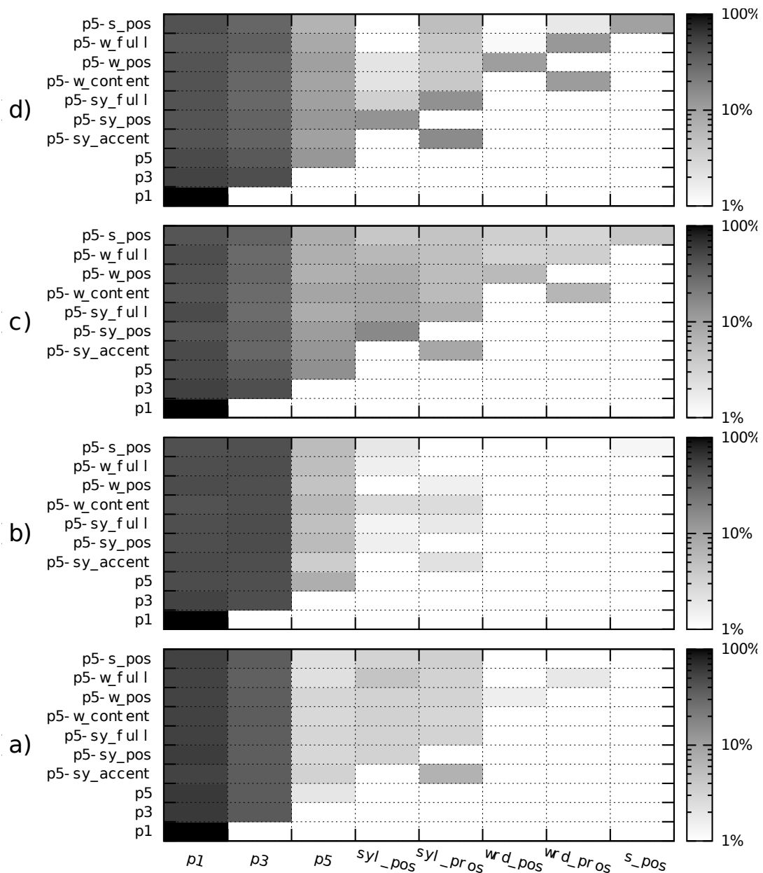
FIGURE 5.12 – Proportion des catégories de questions utilisées pour caractériser les segments du corpus de test pour les coefficients MGC (a), les coefficients d’apériodicité (b), le \log(F_0) (c) et la durée (d). Cette proportion est calculée pour chacun des jeux de descripteurs et représentée par un niveau de gris à l’échelle logarithmique. L’axe des abscisses identifie les catégories de questions : p1, p3, p5 correspondent aux questions liées à l’échelle du segment phonétique et en tenant compte, respectivement des horizons 0, 1 et 2 ; syl_pos, wrd_pos et s_pos correspondent aux informations de position pour, respectivement, les horizons de la syllabe, du mot et de la phrase ; syl_pros et wrd_pros correspondent aux informations d’accentuation pour, respectivement, les horizons de la syllabe et du mot.
