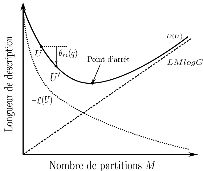
FIGURE 2.7 – Illustration du critère MDL. Figure inspirée de [Yamagishi2006a]
