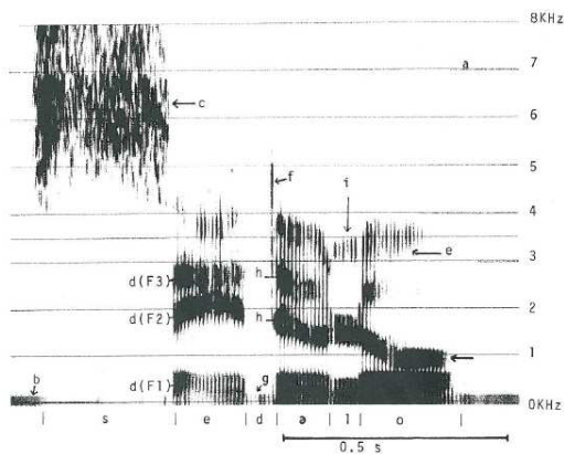
FIGURE 1.3 – Spectrogramme de la phrase "C'est de l'eau". Cette figure est extraite de [Calliope1989].
