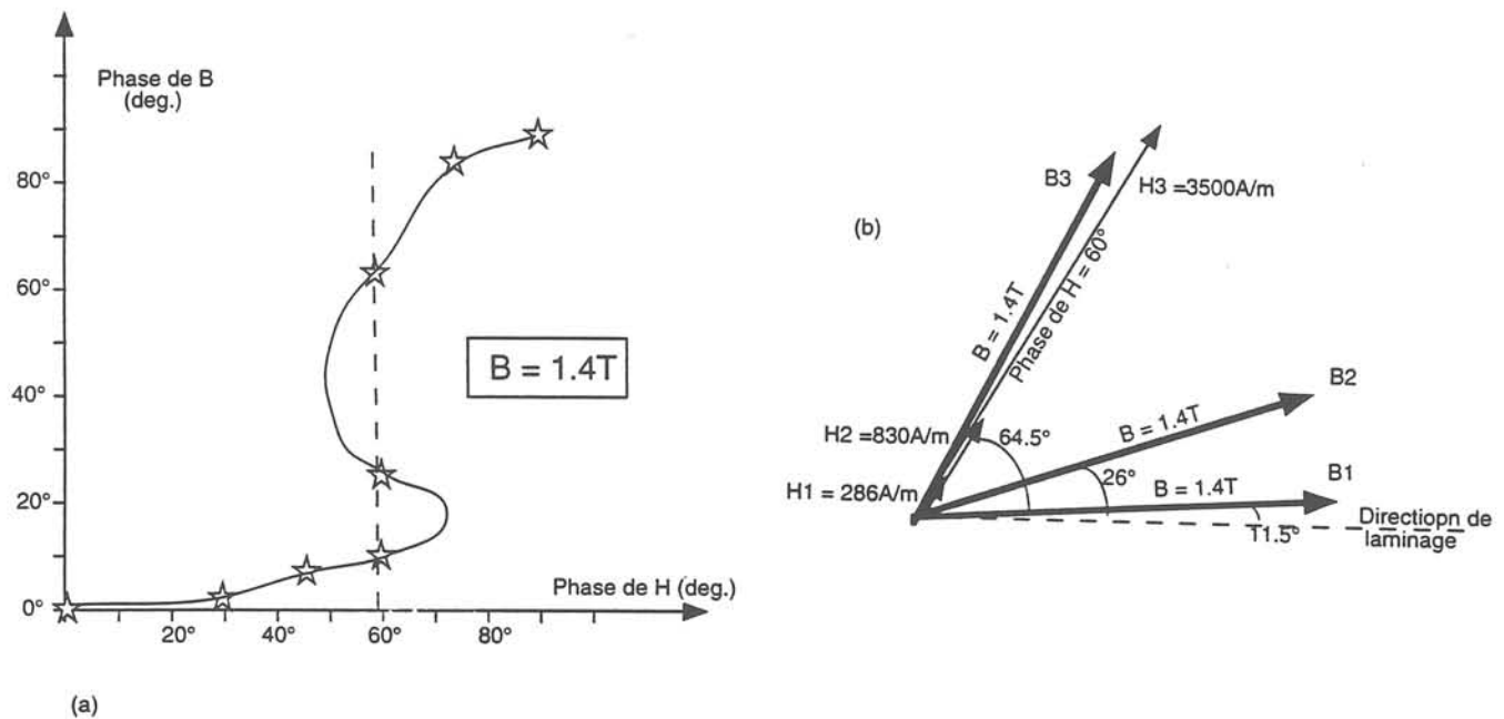
Fig. 4.25 : (a) Relation entre phases de B et H à 1.4 T. Mise en évidence de 3 phases d'équilibre possibles (b) Relation d'anisotropie B-H à module d'induction imposé (1.4 T) et phase de H imposée (60°). Cas de tôles Fe3%Si G.O. M6H d'après Hofman [3]
