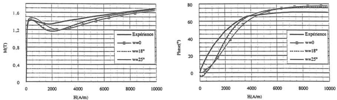
Fig.4.31 : Comparaison du modèle des 2 familles avec l'expérience dans le cas d'une texture Goss, pour différentes désorientations (W) de la texture ; cas d'un champ appliqué à 60^\circ de la direction de laminage
