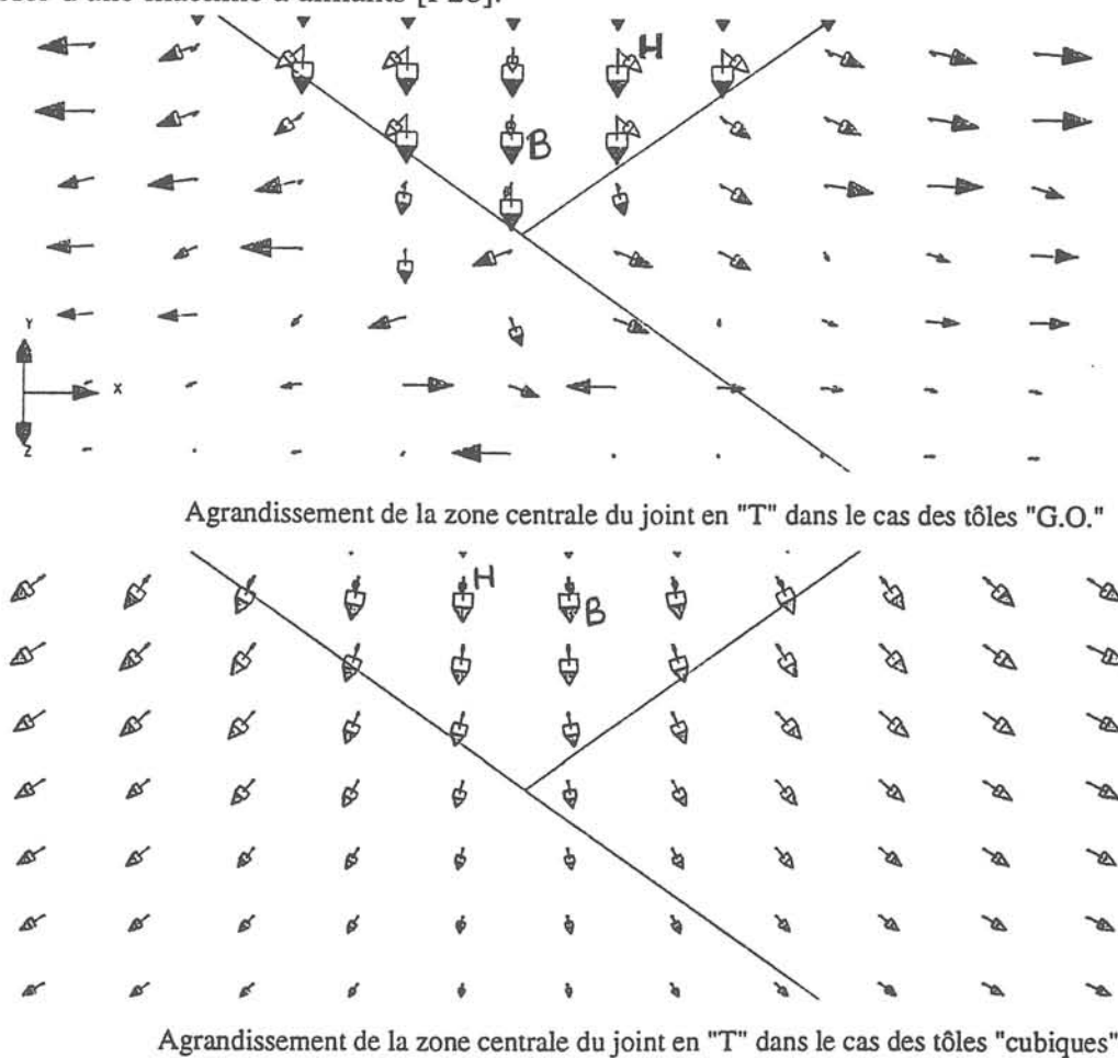
Fig.4.26 : Modélisation d'un joint de transformateur triphasé : mise en évidence des hétérogénéités spatiales locales de \mathbf{H} et \mathbf{B} dans les zones de forte instabilité magnétique dans le cas d'une tôle G.O. (fig.4.26.a) ; transitions spatiales de \mathbf{H} et \mathbf{B} beaucoup plus progressives dans le cas d'une tôle à texture "cubique" (fig.4.26.b)
