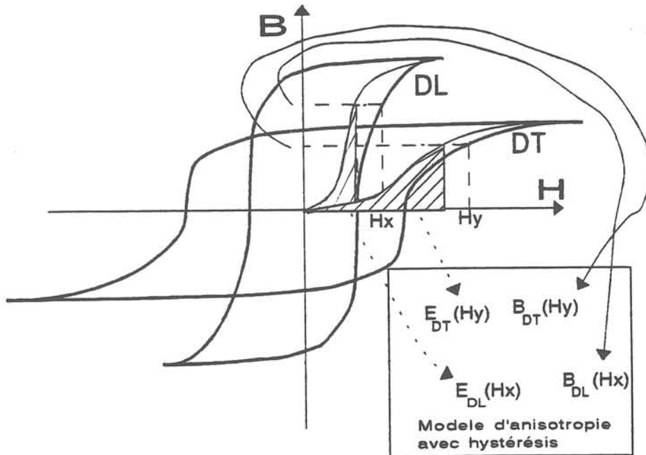
Fig.4.32 : Principe de construction d'un modèle anisotrope anhystérique
