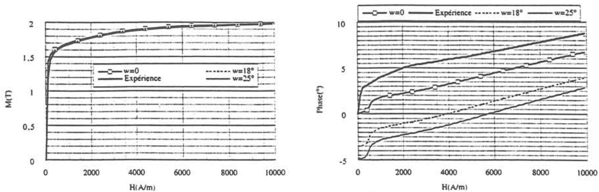
Fig.4.30 : Comparaison du modèle des 2 familles avec l'expérience dans le cas d'une texture de Goss, pour différentes désorientations (W) de la texture ; cas d'un champ appliqué à 30^\circ de la direction de laminage
