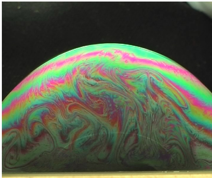
FIG. 3.7: Photographie de la demi-bulle en convection à \Delta T = 21^\circ\text{C} .
