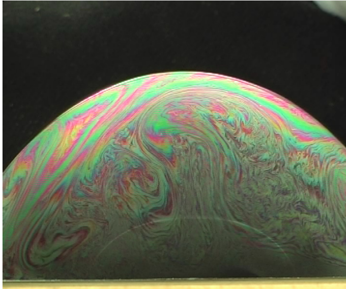
FIG. 3.8: Photographie de la demi-bulle en convection à \Delta T = 40^\circ\text{C} .
