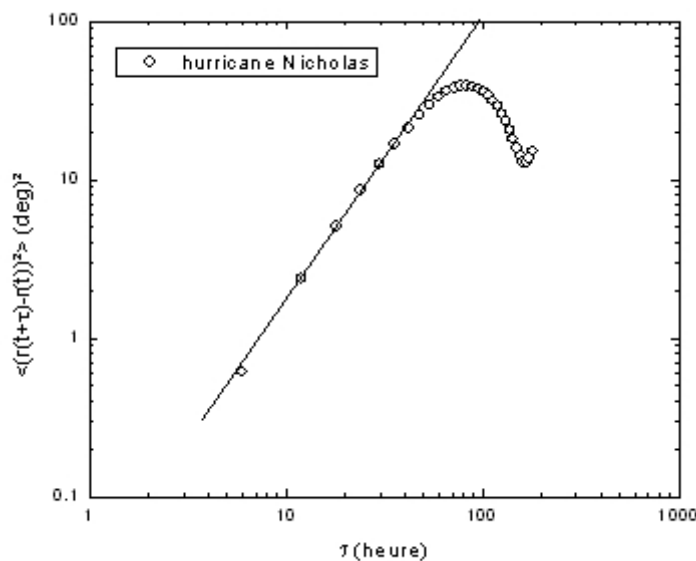
FIG. 5.10: Déplacement quadratique moyen de l'ouragan Nicholas.
