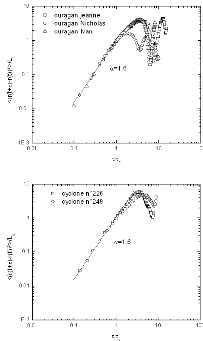
FIG. 5.11: Déplacement quadratique moyen d'ouragans du bassin Atlantique nord.
