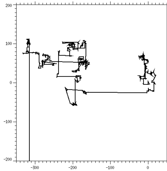
FIG. 4.18: Exemple de "saut de Lévy" en deux dimension.
