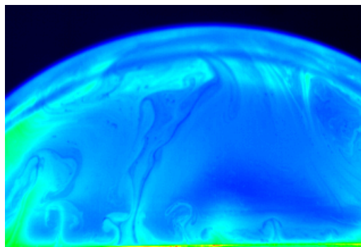
FIG. 8.1: Champ de température pour \Delta T = 40^\circ C .
