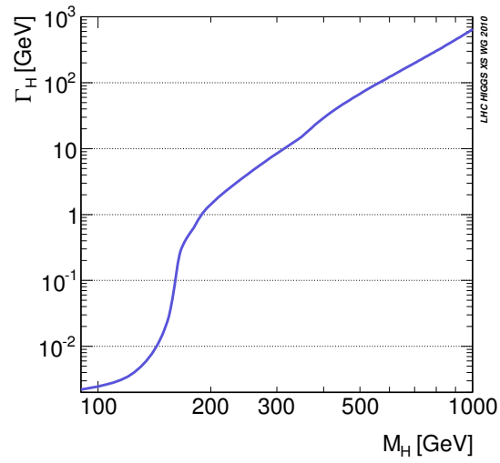
FIGURE 1.13 – Largeur intrinsèque du boson de Higgs (tiré de [28])
