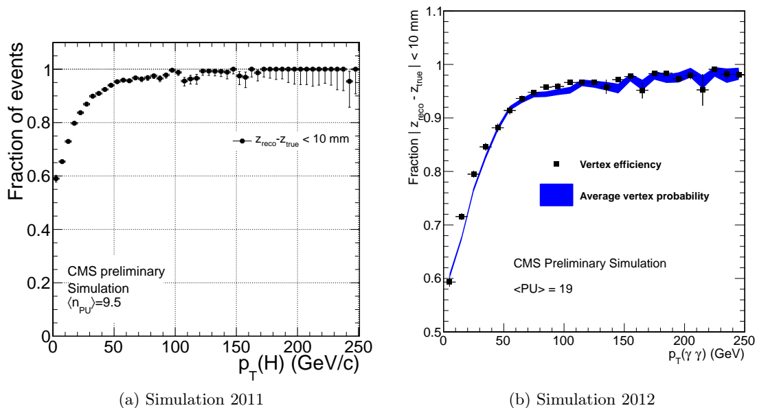
FIGURE 5.3 – Efficacité de l'arbre de décision boosté de sélection du bon vertex pour des événements simulant la désintégration d'un boson de Higgs en deux photons avec m_H = 120 \text{ GeV} , dans les conditions de prises de données 2011 (gauche, [91]) et 2012 (droite, [92]).
