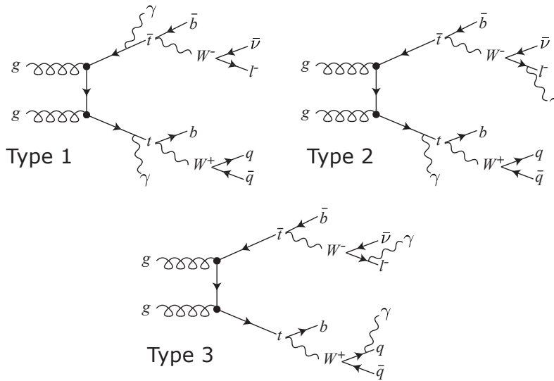
FIGURE 6.2 – Diagrammes de Feynman illustrant les trois types de radiations dans l'état final dans les événements t\bar{t} + \text{jets} dans l'analyse t\bar{t}H, H \rightarrow \gamma\gamma du Technical Design Report de l'expérience CMS [104]. Les photons à l'état final peuvent soit provenir des radiations des quarks top dans l'état final (Type 1), soit des radiations des produits de désintégrations des quarks top (Type 3), soit d'une combinaison de ces deux types (Type 2). Par défaut dans Alpgen, seul le type 1 est inclus, tandis que pour l'analyse de ce Technical Design Report, une version privée, développée par les auteurs d'Alpgen, a été utilisée. Le développement d'Alpgen a continué par la suite, et cette version privée n'est plus compatible avec la dernière version d'Alpgen (notamment à cause de changements dans la syntaxe des cartes de génération). Il n'a pas été possible techniquement d'inclure cette ancienne version privée d'Alpgen dans la dernière version. On sait cependant grâce à cette analyse t\bar{t}H, H \rightarrow \gamma\gamma que l'on peut sous-estimer la section efficace totale du processus \gamma\gamma + t\bar{t} + N jets de près de 90 %, lorsque les diagrammes de type 2 et 3 ne sont pas considérés. L'étude de l'interférence entre ces différents diagrammes, et l'étude d'un possible double comptage des photons avec ceux générés par le programme d'hadronisation (ici Pythia), devraient également être réalisées pour une modélisation correcte de ce processus.
