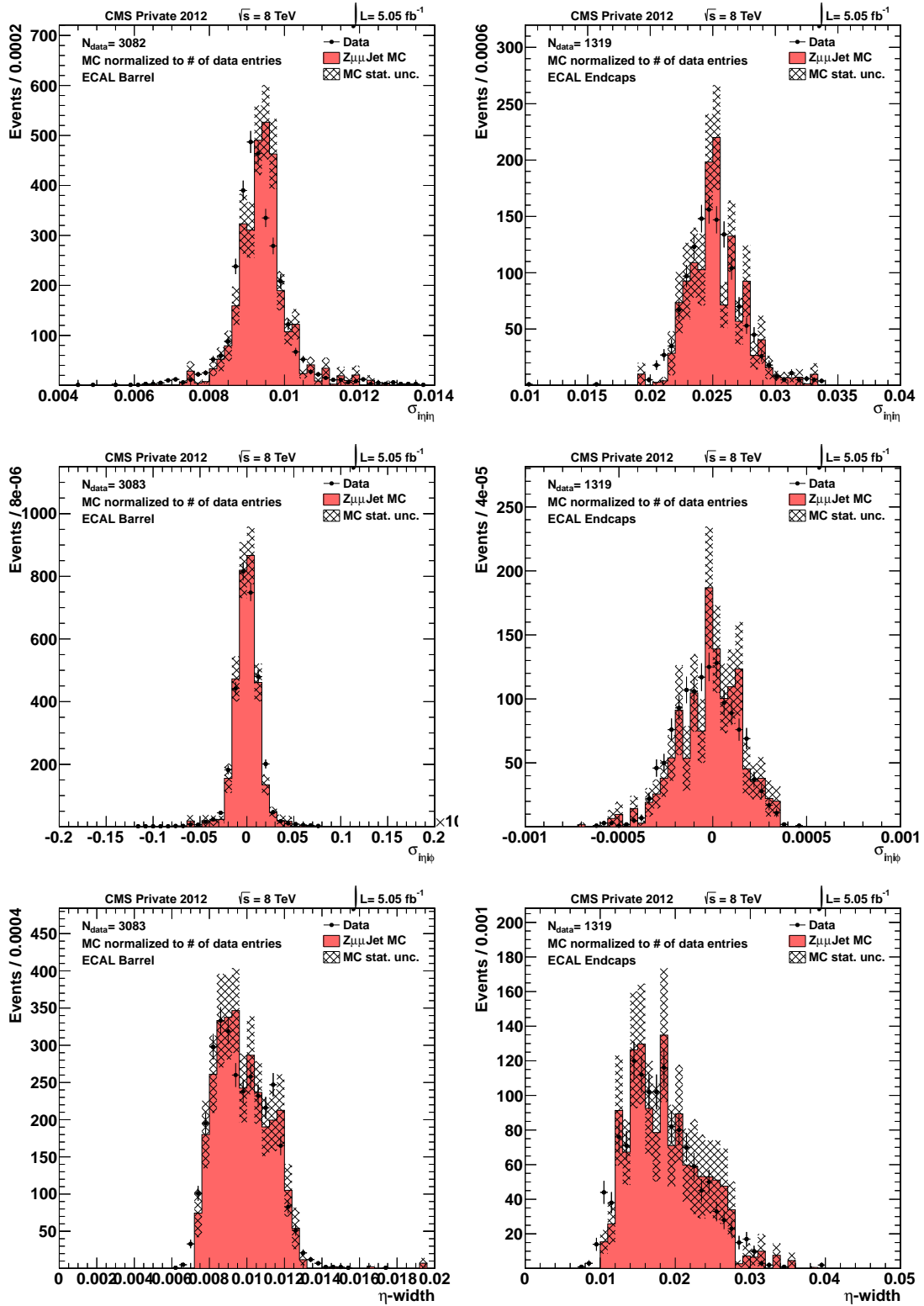
FIGURE 5.6 – Distributions des variables de forme du cluster \sigma_{inh} (haut), \sigma_{in\phi} (milieu) et \sigma_{\eta} (bas) pour le tonneau (gauche) et les bouchons (droite) dans les événements Z^0 \rightarrow \mu\mu\gamma .
