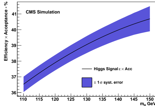
FIGURE 5.14 – Produit acceptation fois efficacité pour l’analyse présentée dans ce chapitre, en fonction de l’hypothèse de masse, pour toutes les classes d’événements combinées, dans la simulation à 8 TeV. Figure tirée de [92].
