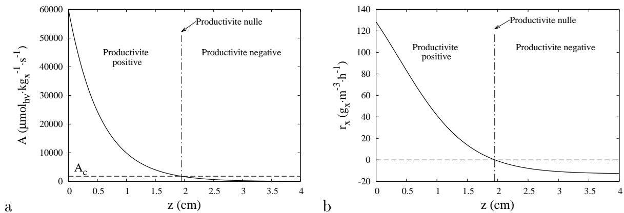
FIGURE 1.8: Champs dans la configuration simplifiée du photobioréacteur torique Fig. 1.5 pour un milieu gris purement absorbant. E = 4 \text{ cm} ; C_x = 0.9 \text{ kg}_x \cdot \text{m}^{-3} ; q_\Gamma = 300 \mu\text{mol}_{h\nu} \cdot \text{m}^{-2} \cdot \text{s}^{-1} ; \sigma_a = 200 \text{ m}^2 \cdot \text{kg}_x^{-1} . a : Champ de la vitesse spécifique locale d'absorption des photons \mathcal{A} . b : Champ de la productivité volumique locale r_x pour la loi de couplage de Chlamydomonas reinhardtii (voir l'annexe B et fig. 1.4).
