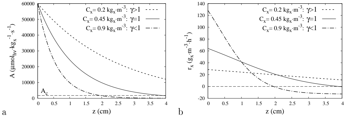
FIGURE 1.9: Règle du \gamma = 1 dans la configuration simplifiée du photobioréacteur torique Fig. 1.5 pour un milieu gris purement absorbant : E = 4 \text{ cm} ; q_{\cap} = 300 \mu\text{mol}_{h\nu} \cdot \text{m}^{-2} \cdot \text{s}^{-1} ; \sigma_a = 200 \text{ m}^2 \cdot \text{kg}_x^{-1} . a : Champ de la vitesse spécifique locale d'absorption des photons \mathcal{A} . b : Champ de la productivité volumique locale r_x pour la loi de couplage de Chlamydomonas reinhardtii (voir l'annexe B et fig. 1.4). Les figures a et b sont obtenues pour trois concentrations C_x représentatives des situations \gamma < 1 , \gamma = 1 , \gamma > 1 .
