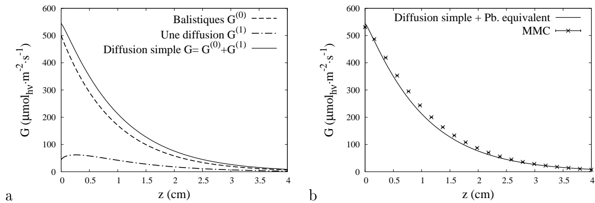
FIGURE 4.12: Champ d'irradiance \hat{G} dans le photobioréacteur Fig. 4.1; \rho^{\mathcal{R}} = 0 ; incidence collimatée normale. Résultats du problème de transport équivalent \alpha_s^* = 0.25 , k_{ext}^* = 110 \text{ m}^{-1} pour l'approximation de la diffusion simple. a : Proportion de photons balistiques et diffus. b : Comparaison avec la solution de référence (Méthode de Monte Carlo, MMC).
