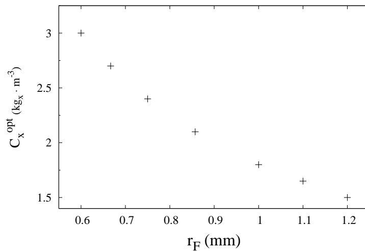
FIGURE 6.4: Concentration C_x optimale assurant une productivité \langle r_x \rangle maximale pour chacune des géométries définies par le rayon r_F des fibres (voir Fig. 6.3). Résultats obtenus par un balayage de l'espace des C_x qui a été guidé par la valeur de la sensibilité \partial_{C_x} \langle r_x \rangle . La valeur C_x^{\text{opt}} est définie telle que \partial_{C_x} \langle r_x \rangle (C_x^{\text{opt}}) = 0 .
