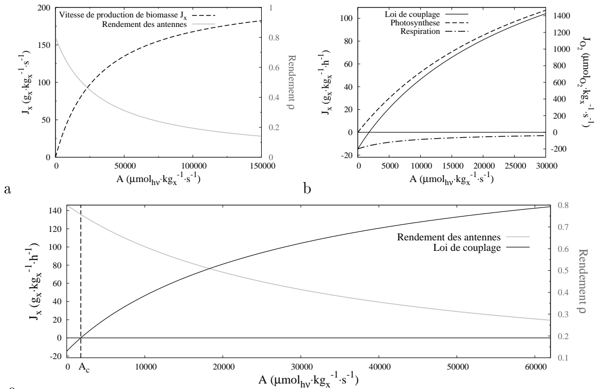
FIGURE 1.4: Loi de couplage cinétique d'un eucaryote (voir encart 1 pour une discussion sur les unités choisies). Les valeurs des paramètres utilisées sont celles obtenues pour Chlamydomonas reinhardtii dans l'annexe B en se basant sur les résultats de [16] : \rho_M = 0.8 , \bar{\phi}' = 1.183 \times 10^{-7} \text{ mol}_{O_2} \cdot \mu\text{mol}_{h\nu}^{-1} , K = 32000 \mu\text{mol}_{h\nu} \cdot \text{kg}_x^{-1} \cdot \text{s}^{-1} , K_r = 7500 \mu\text{mol}_{h\nu} \cdot \text{kg}_x^{-1} \cdot \text{s}^{-1} , \beta = 2 \times 10^{-4} \text{ mol}_{O_2} \cdot \text{kg}_x^{-1} \cdot \text{s}^{-1} . a : Production de biomasse par photosynthèse et rendement des antennes photosynthétiques. b : Bilan entre production de biomasse par photosynthèse et consommation par respiration. c : Loi de couplage et définition du point de compensation A_c ; dans le cas présent A_c = 1800 \mu\text{mol}_{h\nu} \cdot \text{kg}_x^{-1} \cdot \text{s}^{-1}
