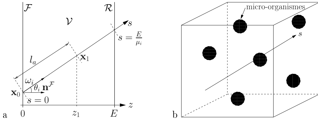
FIGURE 4.6: Chemin optique des photons en l'absence de diffusion. a : Demi-droite \mathbf{x}_0 + s \boldsymbol{\omega}_i d'abscisse curviligne s \in [0, \infty] . b. Propagation des photons sur leur chemin optique dans la suspension de micro-organismes.
