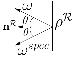
FIGURE 7.7: Définition de la direction spéculaire \omega^{spec} associée à la direction \omega .
