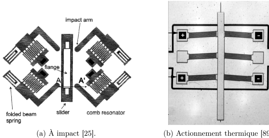
FIGURE 1.8 – Convoyeurs micrométriques.
