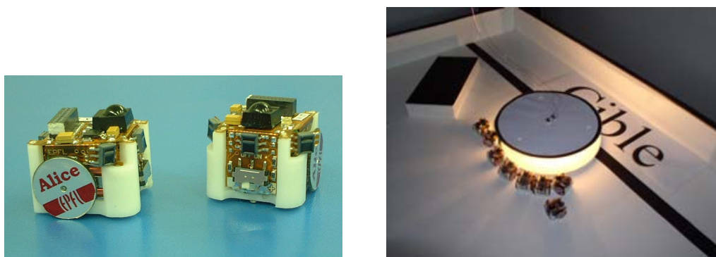
FIGURE 1.2 – Minirobots à roues Alice [13] travaillant en coopération pour pousser un objet vers une cible [4].
