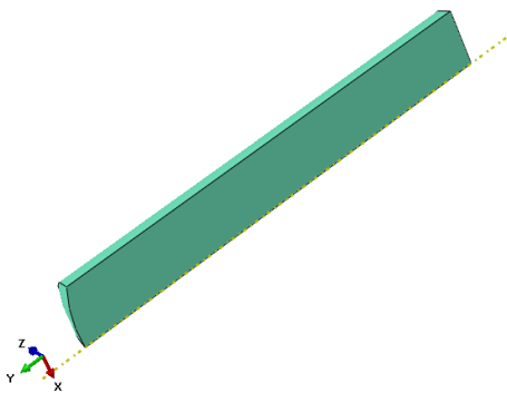
Figure 4-47. Modèle d'un quart du projectile
