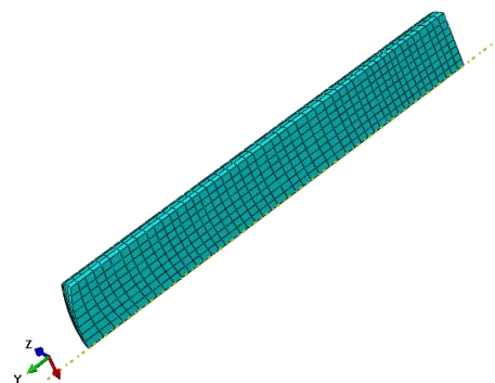
Figure 4-48. Maillage d'un quart du projectile
