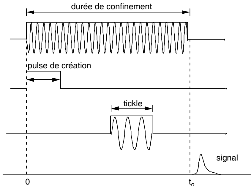
Figure 3.7. Principe de la méthode d'éjection résonnante.
