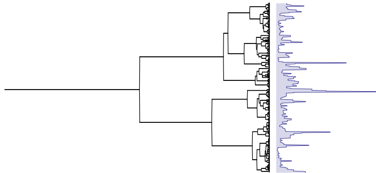
Figure 1.6 – Une simulation de \Delta et de sa mesure harmonique au niveau 1. Clairement cette dernière n’est pas uniforme et a un comportement fractal.
