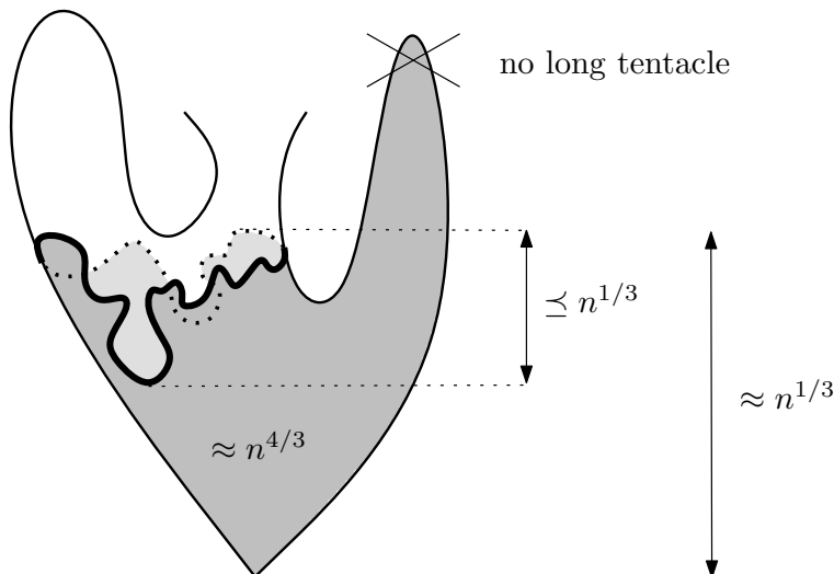
Figure 2.16 – Illustration de la preuve de la sous-diffusivité.
