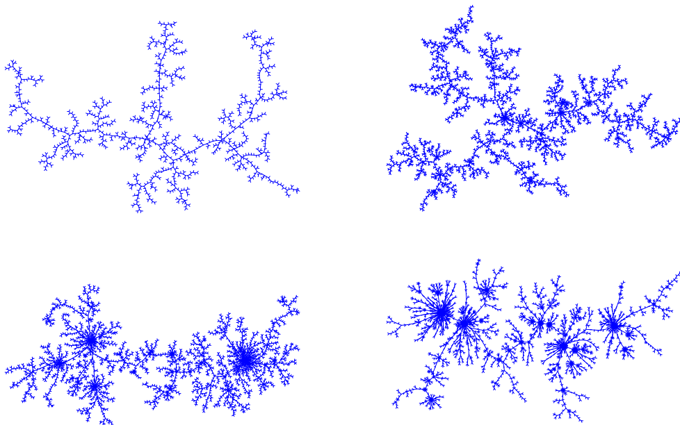
Figure 1.2 – Photo de famille. De haut en bas et de gauche à droite des simulations (approchées) de \mathcal{T}_2, \mathcal{T}_{1.9}, \mathcal{T}_{1.5} et \mathcal{T}_{1.2}
