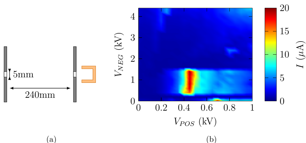
FIGURE 2.21 – Réglage des électrodes d'extraction : (a) schéma de la coupelle de faraday munie d'un système de définition d'émittance. (b) Intensité d'un faisceau de \text{He}^+ à 5 keV lors du balayage des potentiels d'extraction.
