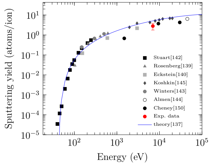
FIGURE 4.17 – Rendement de pulvérisation du tungstène irradié avec des ions Xe + en fonction de l'énergie du projectile.
