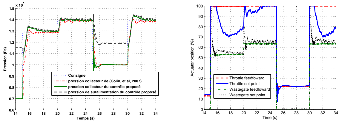
(a) Pressions (Pa) en fonction du temps (s) : consigne p_{man}^{sp} (pointillés bleus), p_{man} avec le contrôle proposé dans [Colin et al. , 2007b] (points-tirets rouges), p_{man} avec le contrôle proposé (trait plein vert), p_{boost} pression de suralimentation du contrôle proposé
