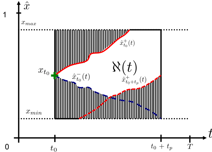
FIGURE 2.12 – Réduction de la grille de recherche de la programmation dynamique prenant en compte les contraintes : \hat{x}_{t_0+t_p}^+(t) est la recharge maximale respectant les contraintes d'état de charge, \hat{x}_{t_0}^-(t) (resp. \hat{x}_{t_0}^+(t) ) est la trajectoire maximale de décharge (resp. recharge) en partant de l'état de charge x_{t_0}
