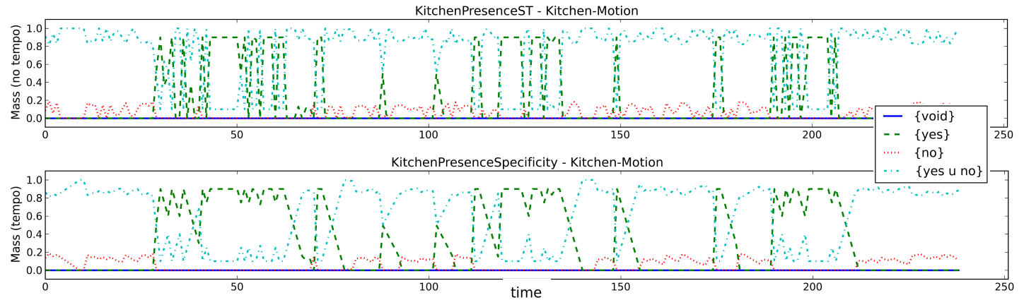
FIGURE 4.5 – Croyances induites par un capteur de mouvement pour la détection de la présence dans une pièce. La personne se déplace dans les intervalles [30-62], [120-140] et [190-215]. Une temporisation avec T_{max} = 6s est appliquée.
