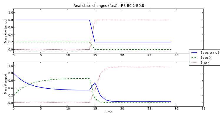
FIGURE 4.12 – Effet de la temporisation avec fusion sur la transition d'un état à croyance faible vers un état à croyance forte ( R = 8 ).
