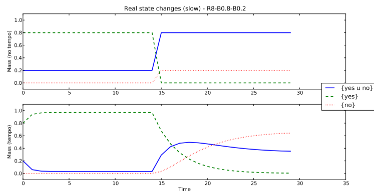
FIGURE 4.11 – Effet de la temporisation avec fusion sur la transition d'un état à croyance forte vers un état à croyance faible ( R = 8 ).
