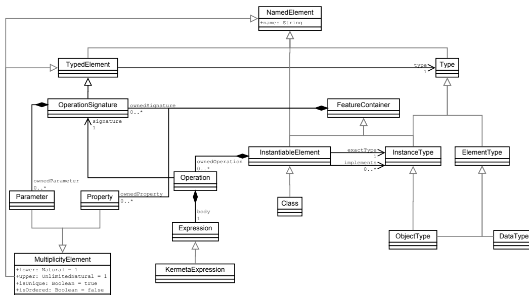
FIGURE 6.2 – Sous ensemble de la syntaxe abstraite du métalangage METAL exposant les concepts communs avec le MOF et Ecore.
