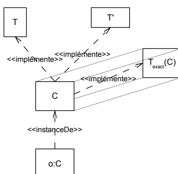
FIGURE 6.5 – Exemple de type exact .
