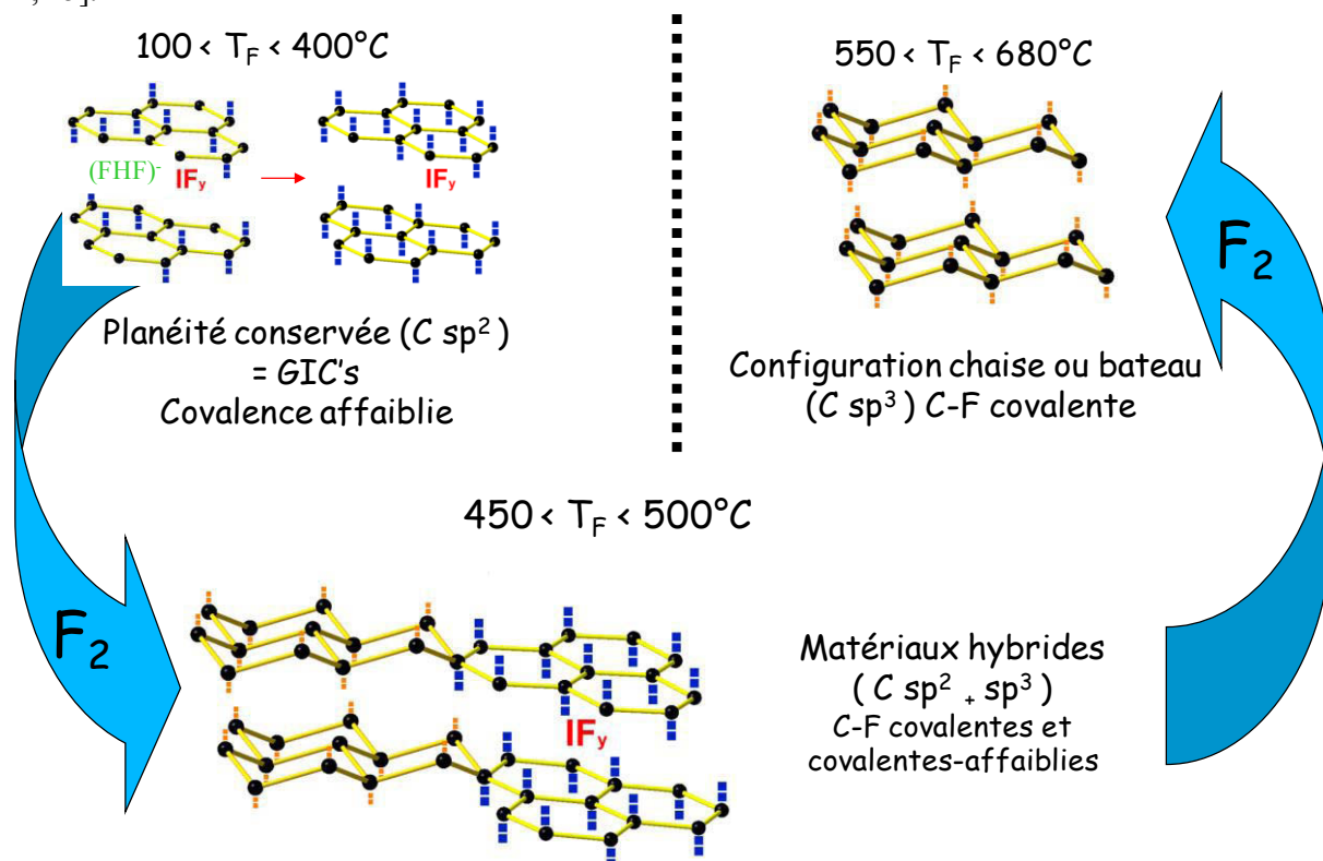
Figure 59. Les étapes de la post-fluoruration de graphite fluoré basse température (cas du mélange catalytique \text{F}_2(\text{g})/\text{HF}(\text{g})/\text{IF}_3(\text{g}) )
