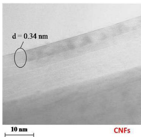
Figure 77. Image MET des NFC MER. La distance interfeuillets mesurée est de 0,34 nm
