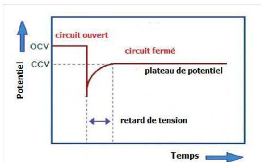
Figure 177. Représentation schématique du fonctionnement d'une pile \text{Li/SOCl}_2
