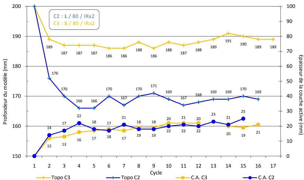
Figure 77 : Évolution de la topographie et de la couche active pour deux modèles contenant chacun 80 % de glace mais l'un composé d'un mélange de sédiment à dominance limoneuse (C2) et l'autre à dominance sableuse (C3). Le dégel est assuré par deux émetteurs IR dont la température à la source est asservie à 300 °C (environ 20 °C en surface des modèles).
