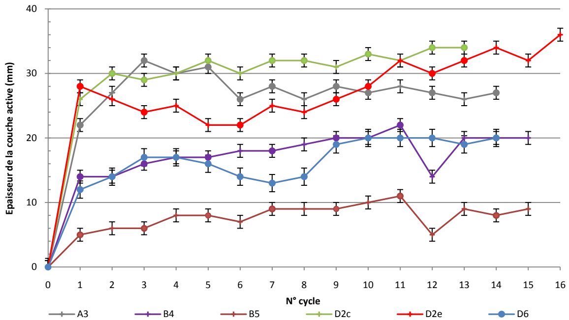
Figure 59 : Exemples d'évolution de l'épaisseur de la couche active en lien avec des ajouts d'eau en surface des blocs de pergélisol. Les marqueurs ronds figurent les cycles où il y a un ajout d'eau.
