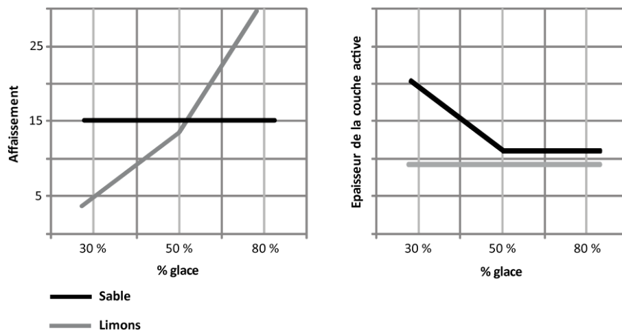
Figure 78 : Récapitulatif de l'évolution de l'affaissement et de l'épaisseur de la couche active en fonction de la lithologie et de la teneur en glace d'un bloc de pergélisol expérimental.
