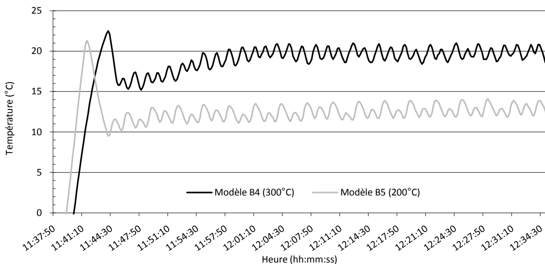
Figure 92 : Température de surface des modèles B4 et B5 durant la phase de réchauffement avec deux émetteurs IR asservis respectivement à la source à 300 et 200 °C.
