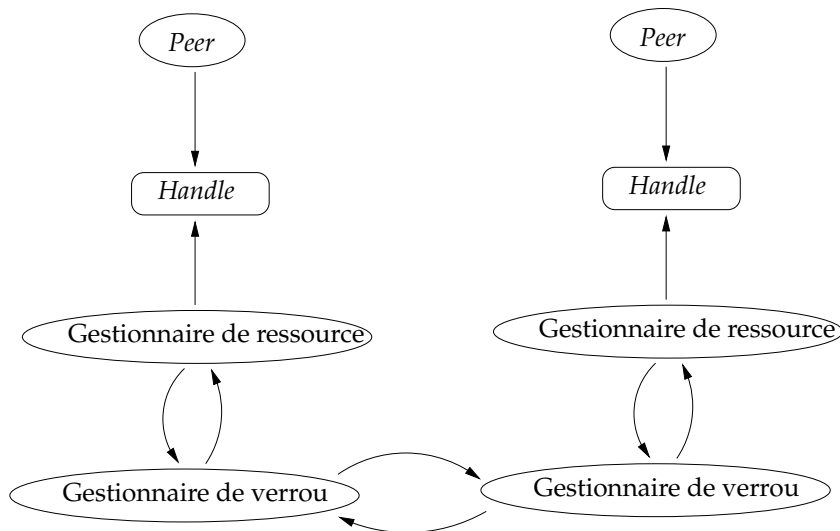
FIGURE 6.2 – Interactions entre processus de chaque peer
