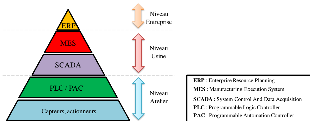
Figure A.7– Exemple de pyramide CIM
