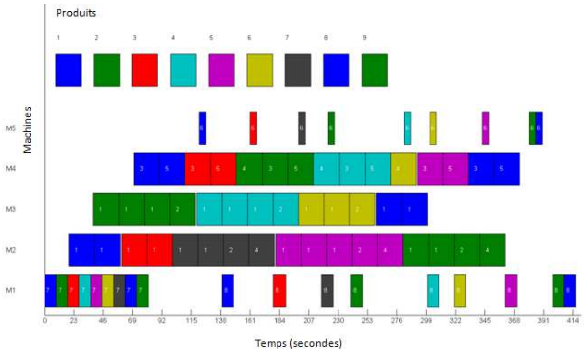
Figure 5.17– Diagramme de GANTT avec les champs de potentiel pour I-A-I-A-A-P-P-I-P
