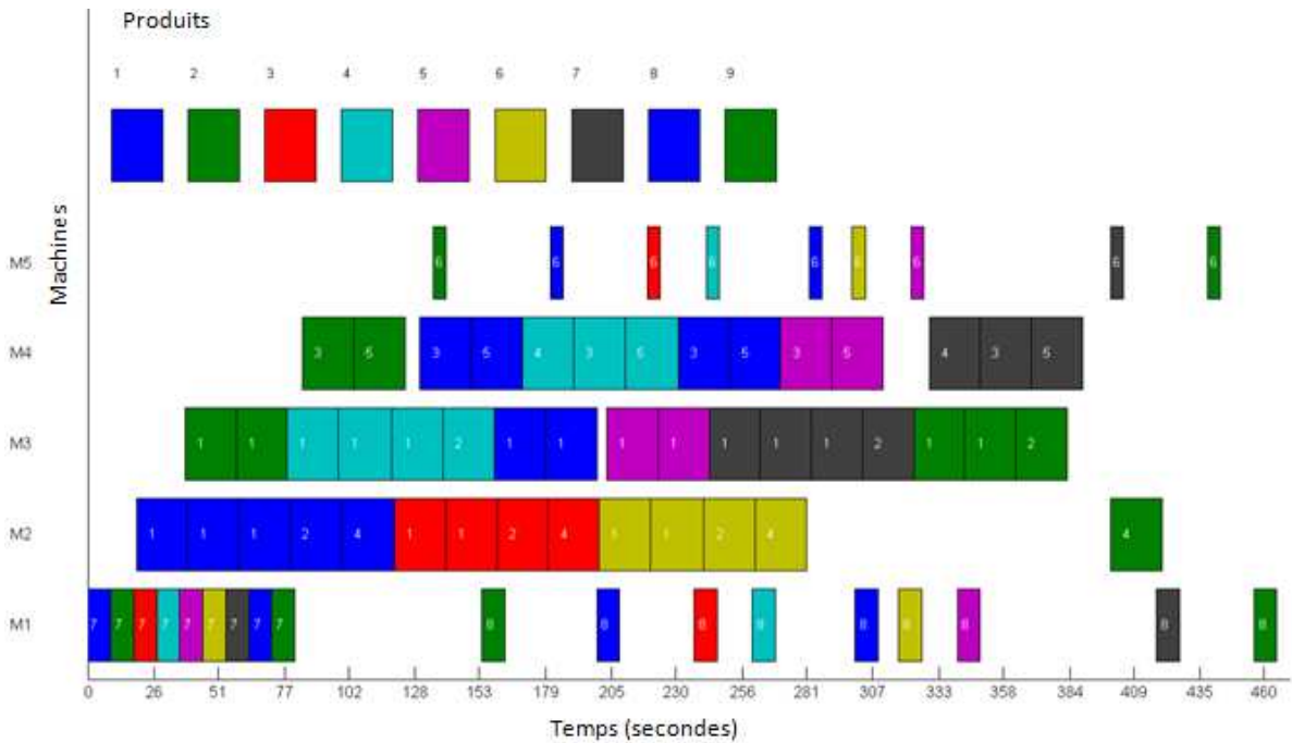
Figure 5.16– Diagramme de GANTT avec les champs de potentiel pour A-I-P-A-I-P-A-I-P
