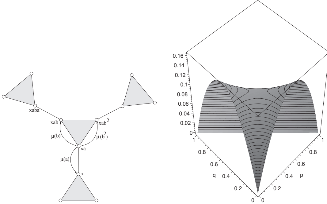
FIGURE 1. A gauche, une marche aléatoire au plus proche voisin sur \mathbb{Z}/2\mathbb{Z} * \mathbb{Z}/3\mathbb{Z} . A droite, la vitesse de fuite de (\mathbb{Z}/2\mathbb{Z} * \mathbb{Z}/3\mathbb{Z}, \mu) en fonction de p = \mu(b) et q = \mu(b^2) .
