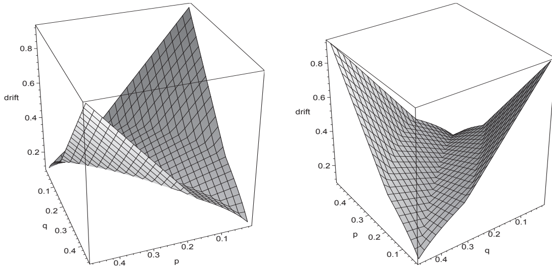
FIGURE 2. La vitesse \gamma en fonction de p = \mu(a) = 1/2 - \mu(b^{-1}) et q = \mu(b) = 1/2 - \mu(a^{-1}) .
