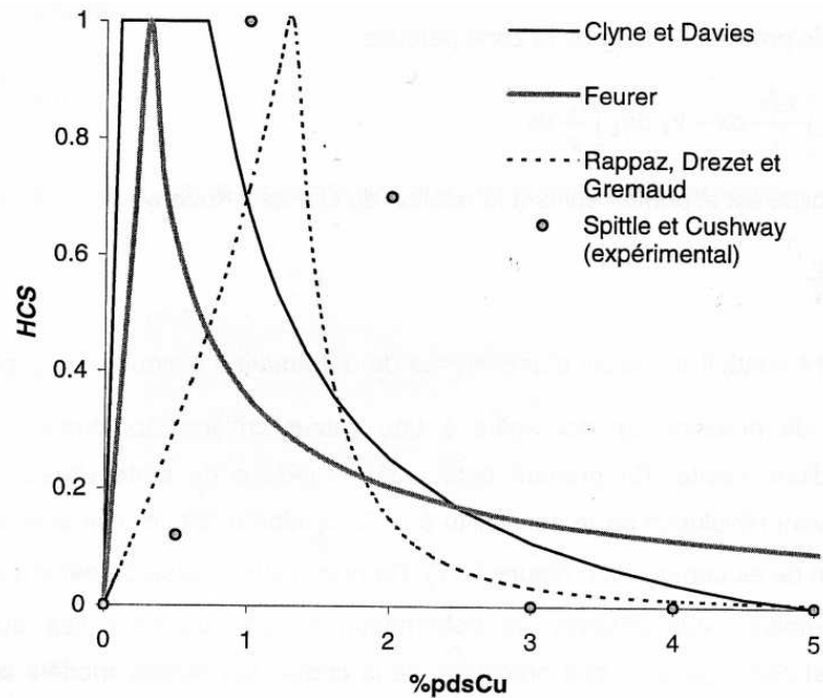
Figure 1.17 – Comparaison de plusieurs critères de fissuration à chaud et les points expérimentaux de Spittle et al. [Spittle & Cushway, 1983] en fonction de la composition d'un alliage Al-Cu [Braccini, 2000]
