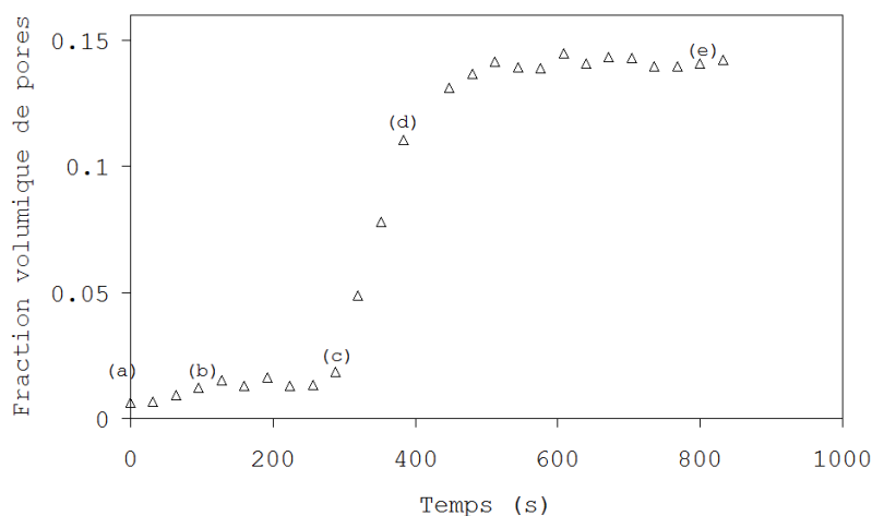
Figure 3.36 – Evolution de la fraction volumique de pores au cours de l'essai. Les lettres réfèrent aux images correspondantes de la figure 3.39
