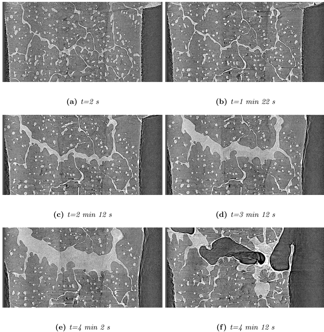
Figure 4.7 – Suivi d'une coupe 2D au cours d'un essai en tomographie rapide d'Octobre 2011 en conditions isothermes. Alliage Al-6pds.%Cu, champ de vue 1320 \times 660\ \mu\text{m} , optiques 1.1\ \mu\text{m} , temps de scan = 2\text{ s} , temps entre deux scans = 10\text{ s} , vitesse de déformation de 6.10^{-4}\ \text{s}^{-1}
