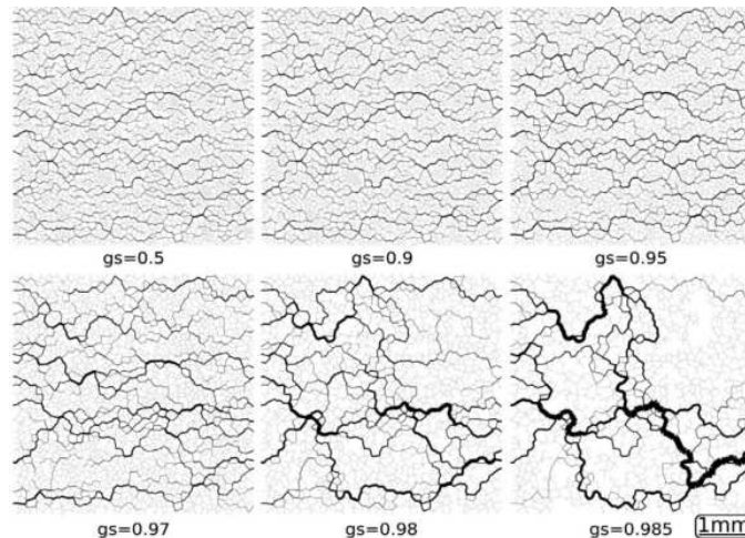
Figure 1.44 – Flux de liquide au sein d'un volume élémentaire ( 5 \times 5 \text{ mm}^2 ) à l'état pâteux en conditions isothermes. L'épaisseur de chaque canal est proportionnelle au flux local normalisé par le flux total
