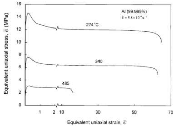
Figure 2.11 – Courbes contrainte-déformation pour de l'aluminium pur en torsion à différentes températures et pour \dot{\epsilon} = 5.8.10^{-4} s^{-1} [Kassner & Pérez-Prado, 2000]
