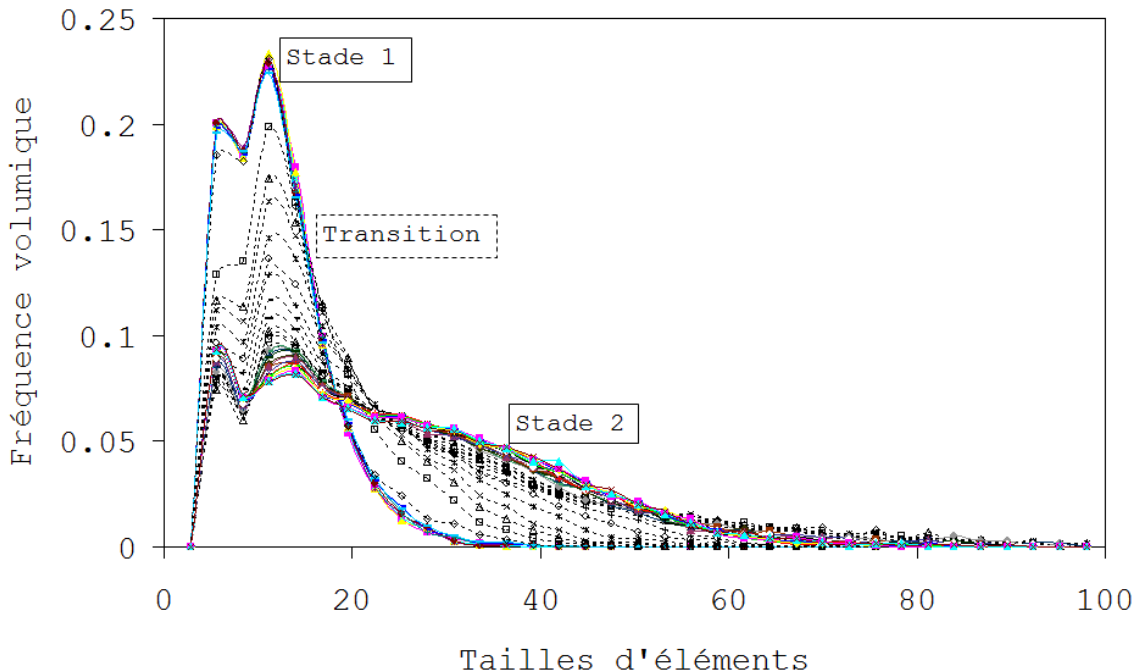
Figure 3.15 – Evolution de la taille des canaux de liquide au cours du temps lors de l'essai en conditions isothermes
