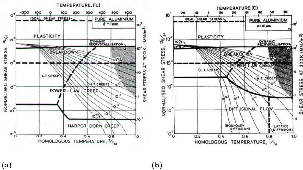
Figure 1.45 – Cartes de mécanismes de déformation (contrainte de cisaillement normalisée-température homologue) pour de l'aluminium pur avec taille de grains de (a) 1 μ m et (b) 1 mm [Frost & Ashby, 1982]
