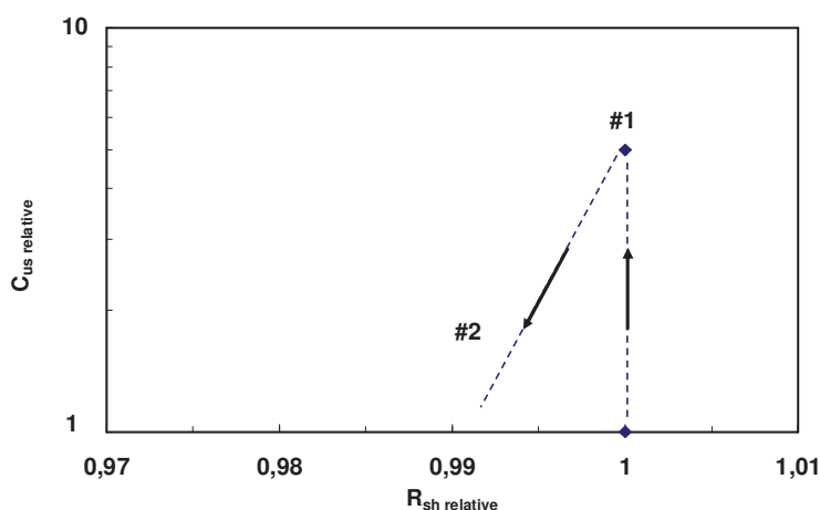
Figure III-34 Simulation issue de notre modèle : C_{us\ relative} en fonction de R_{sh\ relative} en présence d'éclairage.
