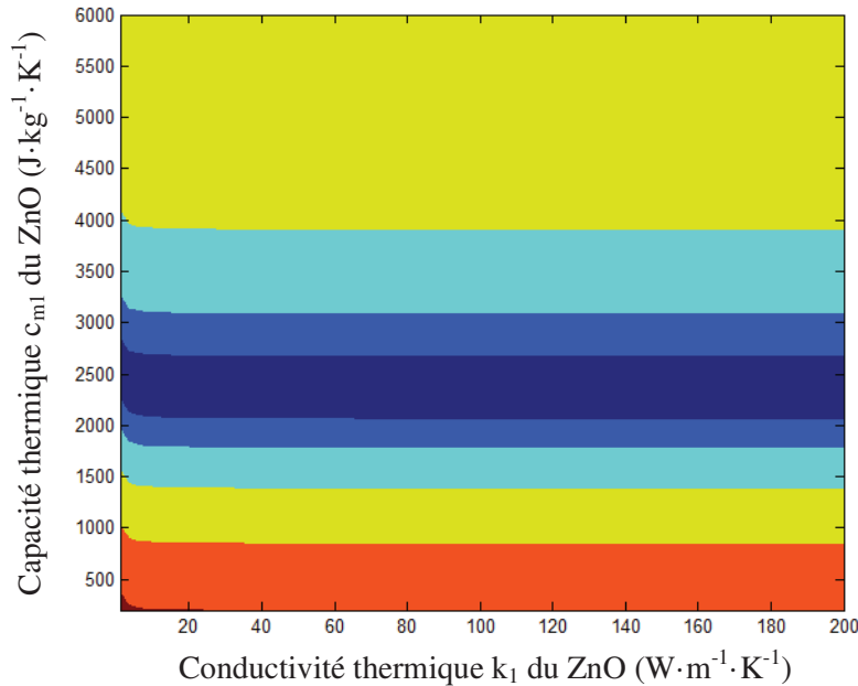
Figure IV-16 Courbe de niveau pour la capacité thermique massique c_{m1} en fonction de la conductivité thermique k_1 de couche de ZnO et paramétrée par \chi^2 .
