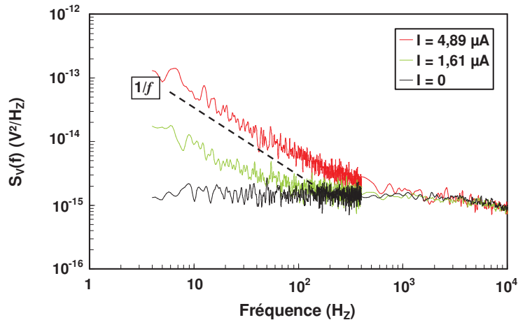
Figure III-15 Exemple de spectres de bruit en 1/f obtenus en fonction de différents courants continus appliqués. La courbe du bas en noir indique le bruit de fond (obtenu avec I = 0 ) (cf. Annexe No.2).
