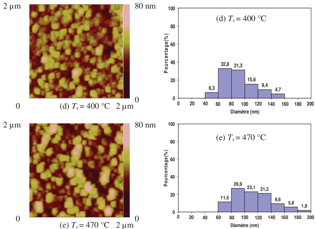
Figure II-12 Images AFM et distributions du diamètre des particules analysées par AFM pour le dépôt de ZnO sur verre à : (a) T_s = 28 \text{ }^\circ\text{C} ; (b) T_s = 100 \text{ }^\circ\text{C} ; (c) T_s = 250 \text{ }^\circ\text{C} ; (d) T_s = 400 \text{ }^\circ\text{C} et (e) T_s = 470 \text{ }^\circ\text{C} (cf. Annexe No.6 et No.18-21).
