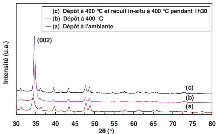
Figure II-23 ZnO sur verre : diffractogrammes des films déposés à (a) T_s = 28 °C ; (b) T_s = 400 °C ; (c) T_s = 400 °C et recuits in-situ à 400 °C pendant 1h30 (cf. Annexe No.6 No.20 No.22).
