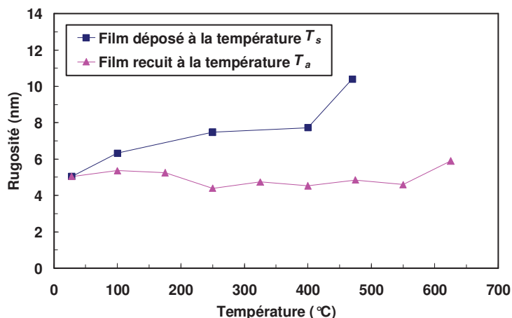
Figure II-24 ZnO sur verre : évolution de la rugosité de la surface des films en fonction de la température de dépôt T_s ou de la température de recuit T_a à l'air (cf. Annexe No.6-14 et No.18-20).
