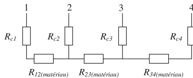
Figure III-3 Schéma équivalent de l'échelle de résistance.
