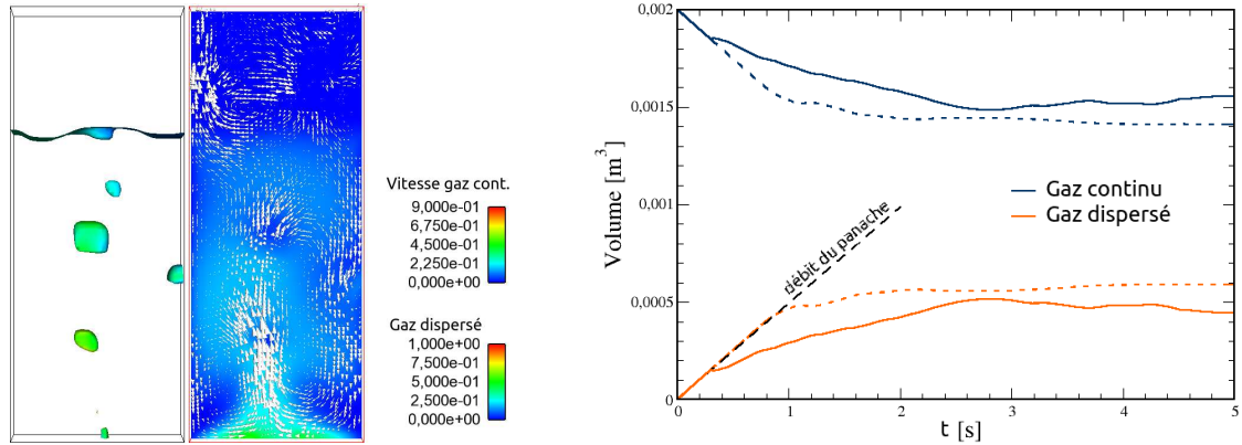
FIGURE 4.5 – Sur la figure de gauche, on juxtapose l'isosurface \alpha_{cg} = 0.5 , indiquant la position de la surface libre et des larges bulles, et la fraction volumique de gaz dispersé à laquelle on a superposé le champs de vitesse moyen de la phase gaz ((\alpha_{dg} \mathbf{U}_{dg} + \alpha_{cg} \mathbf{U}_{cg}) / (\alpha_{dg} + \alpha_{cg})) . Les courbes en pointillés et en traits pleins représentent respectivement les volumes des deux champs gaz calculés sans et avec terme de création de large bulle.
