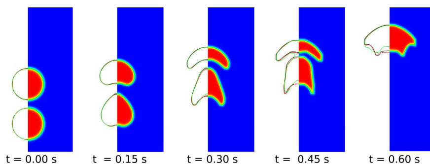
FIGURE 3.23 – Simulation numérique de l’expérience de Chen et al. avec NEPTUNE_CFD. Sur la partie droite de chaque image, on a représenté les interfaces obtenues avec les trois maillages 100 \times 300 (vert), 120 \times 360 (rouge) et 140 \times 420 (noir). La partie de droite montre le taux de vide pour la phase gaz pour le maillage 120 \times 360 .
