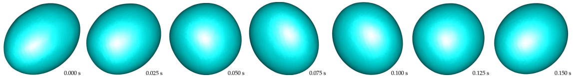
FIGURE 2.24 – Oscillation d'une bulle sphérique ayant subi une déformation d'ordre 2 (ellipsoïdale). L'intervalle de temps entre deux images est de 25 ms. La surface représentée est l'isosurface \alpha_{cg} = 0.5 .
