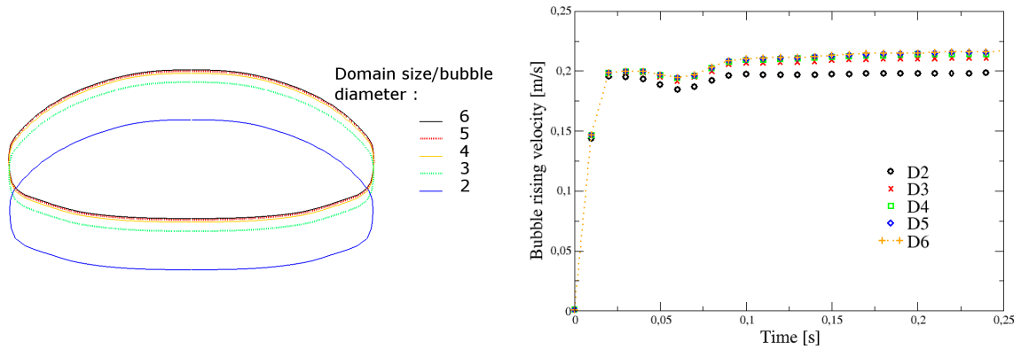
FIGURE 3.15 – Études de la forme de la bulle en fonction de la taille du domaine physique, rayon du domaine de 2 à 6 fois le diamètre de bulle (à gauche).
