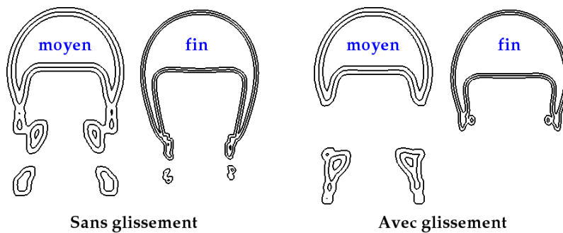
FIGURE 4.7 – Isosurfaces \alpha = 0.1, 0.5 et 0.9 pour les maillages moyen et fin. A gauche sont présentés les résultats avec le modèle d'interface localisé présenté au chapitre précédent, à droite les résultats avec l'ajout d'un glissement pour les interfaces mal résolues.
