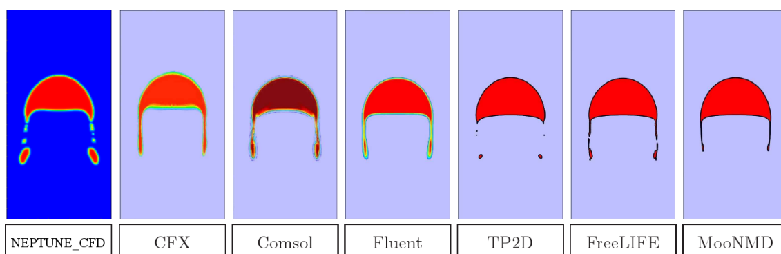
FIGURE 3.12 – Simulation numérique d'une bulle ascendante 2D pour six codes différents (source Hysing [54]) comparée aux résultats obtenus sous NEPTUNE_CFD avec étape de compression artificielle.
