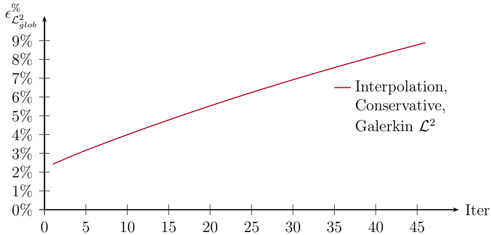
FIGURE 2.9 – Éléments finis de volumes – Évolution de l'erreur \epsilon_{L^2_{glob}}^{\%} . Transfert et mesure de l'erreur effectués en norme \mathcal{L}^2 .
