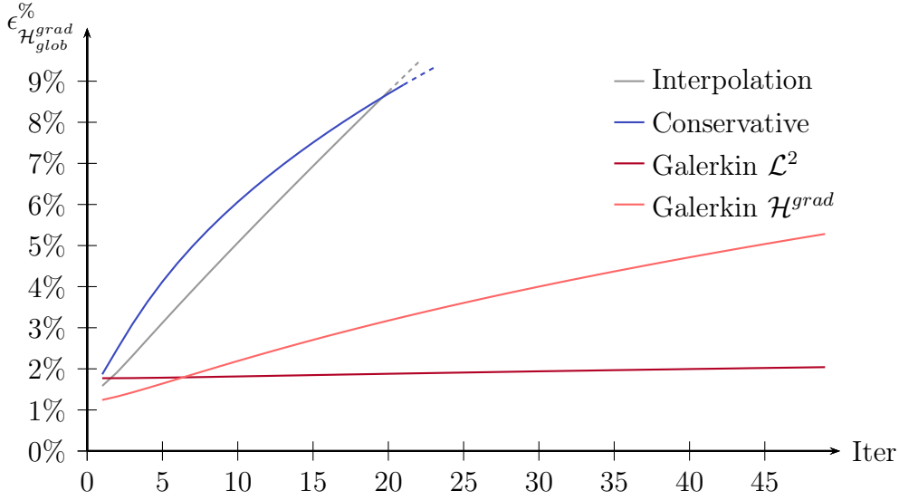
FIGURE 2.4 – Éléments finis nodaux – Évolution de l'erreur \epsilon_{\mathcal{H}^{grad}}^{%} pour la projection orthogonale et des éléments cibles linéaires. Transfert et mesure de l'erreur effectués en norme \mathcal{H}^{grad} .
