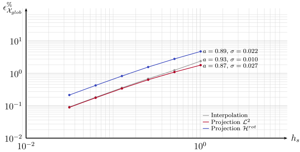
FIGURE 2.11 – Évolution de l'erreur pour des subdivisions successives des maillages source et cible. Cas des transferts des éléments d'arêtes.
