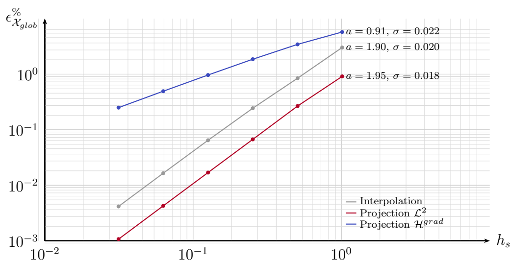
FIGURE 2.10 – Évolution de l'erreur pour des subdivisions successives des maillages source et cible. Cas des transferts nodaux.
