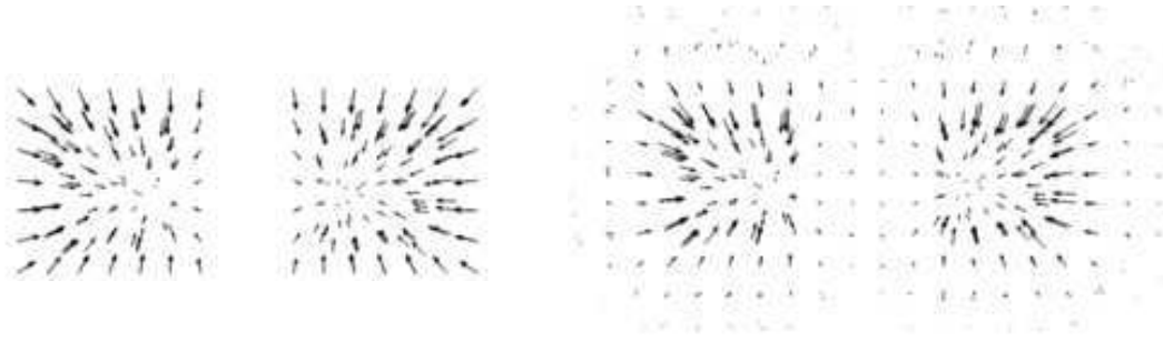
FIGURE 1.4 – Gauche : densité de forme déterminée sur les seules parties mécaniques. Droite : exemple de diffusion de la solution dans l'espace environnant.
