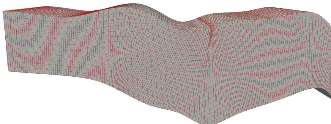
FIGURE 1.11 – Détail des diverses intersections sélectionnées. Les valeurs de directions et de surfaces servent à déterminer la direction et la norme de champ de vecteurs en tous points.
