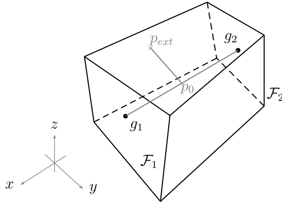
FIGURE 1.3 – Détail de la géométrie du changement de section.
