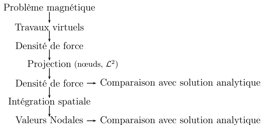
FIGURE 1.8 – Principales étapes utilisées pour le test du couplage à l'aide de la densité de force. Une étape de détermination de la densité de force est nécessaire, une intégration spatiale est ajoutée afin de comparer les valeurs nodales.
