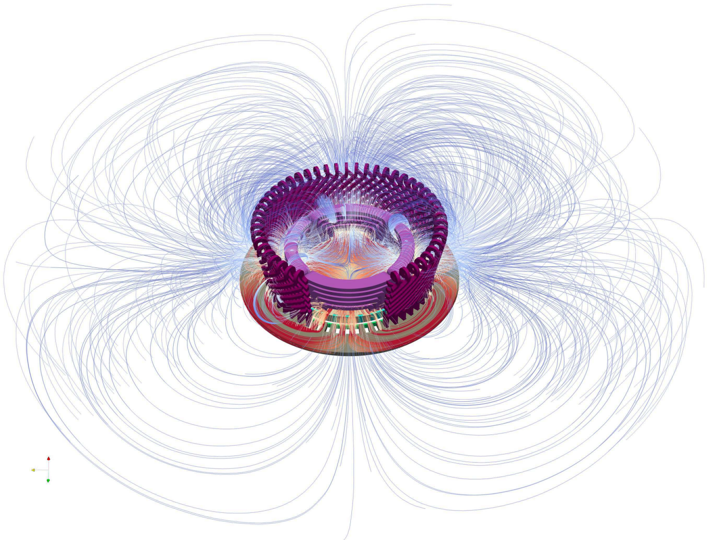
FIGURE 1.30 – Résultat de calcul pour une extrémité d’alternateur à angle interne nul. Le rotor est pris en compte et alimenté.
