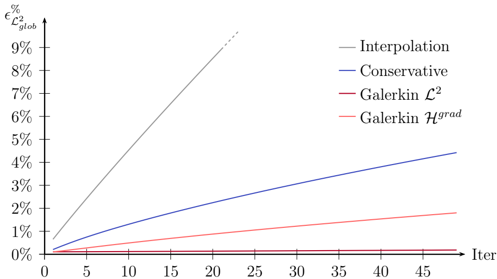
FIGURE 2.3 – Éléments finis nodaux – Évolution de l'erreur \epsilon_{\mathcal{L}^2}^{\%} pour des éléments cibles linéaires. Transfert et mesure de l'erreur effectués en norme \mathcal{L}^2 .
