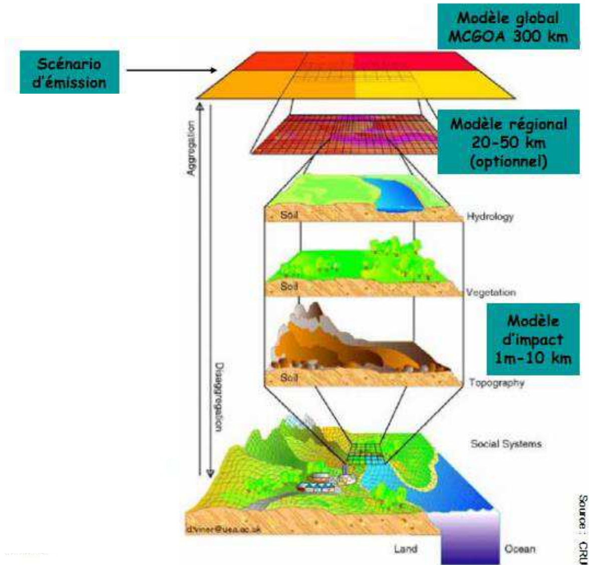
Figure 2.6. Réduction d'échelle de la maille d'un MCG-OA vers une maille à haute résolution spatiale. Sources : Climate Research Unit (D. Viner) et projet Rexhyss.
