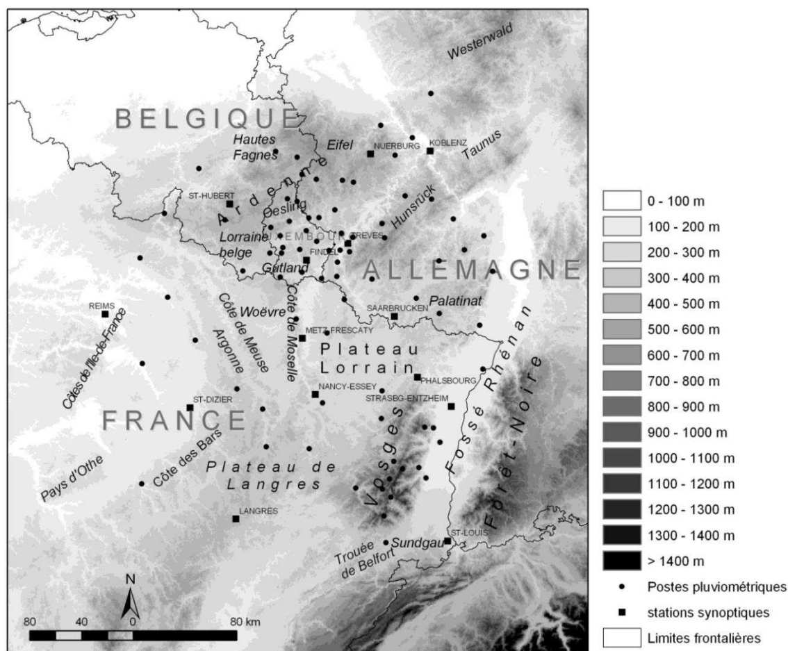
Figure 1.21. Stations pluviométriques, régions naturelles et principales unités topographiques dans l'espace transfrontalier rhéno-mosan (de Bâle à Coblenz). Période postérieure à la SGM.
