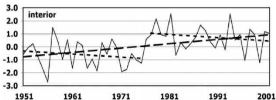
Figure 2.2. Anomalies de température (°C) déduites des températures annuelles enregistrées dans la partie intérieure de l'Alaska entre 1951 et 2001. In Hartmann et Wendler (2005).
