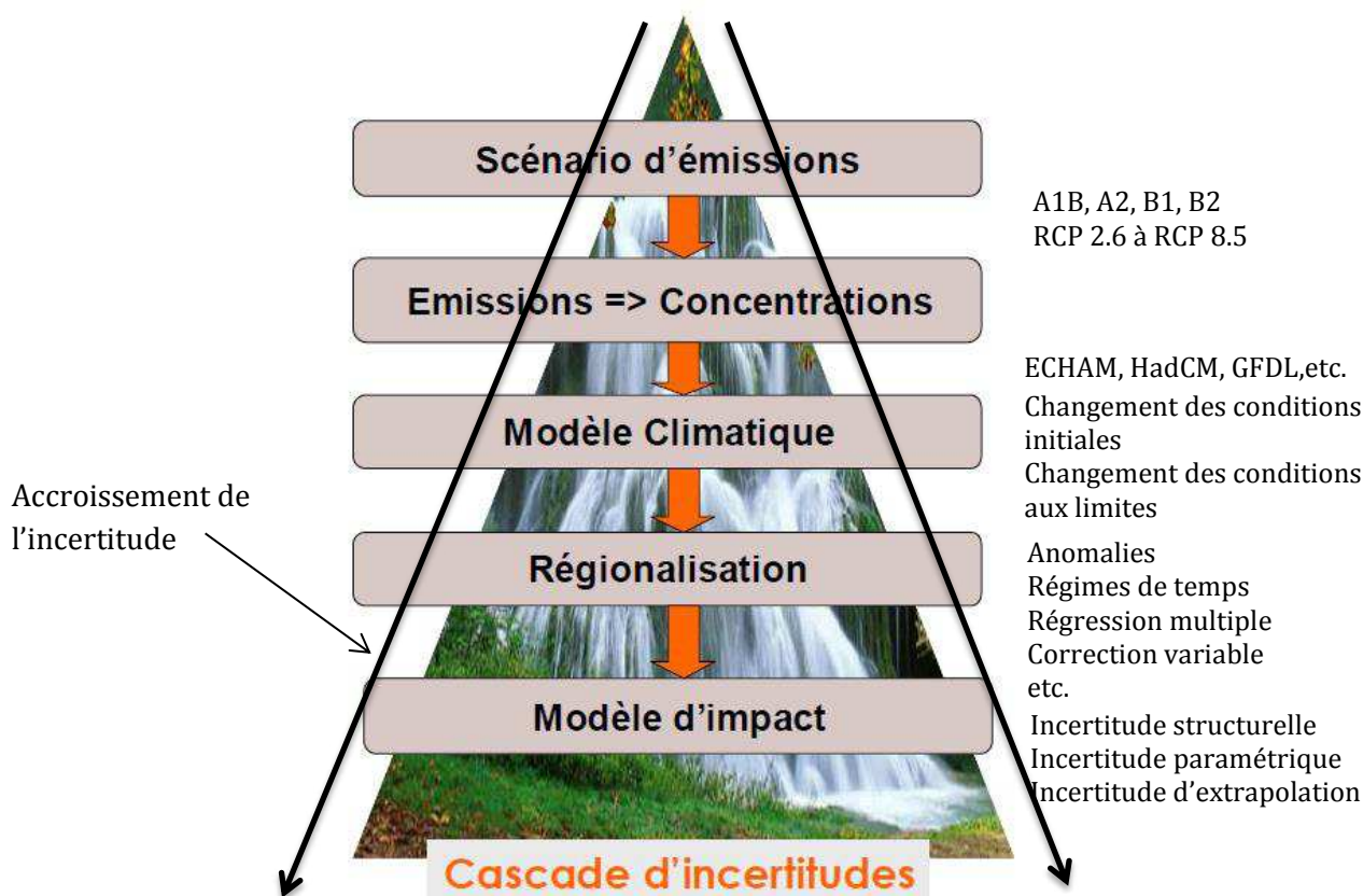
Figure 2.8. Cascade et cône d'incertitudes en modélisation prospective du climat.
