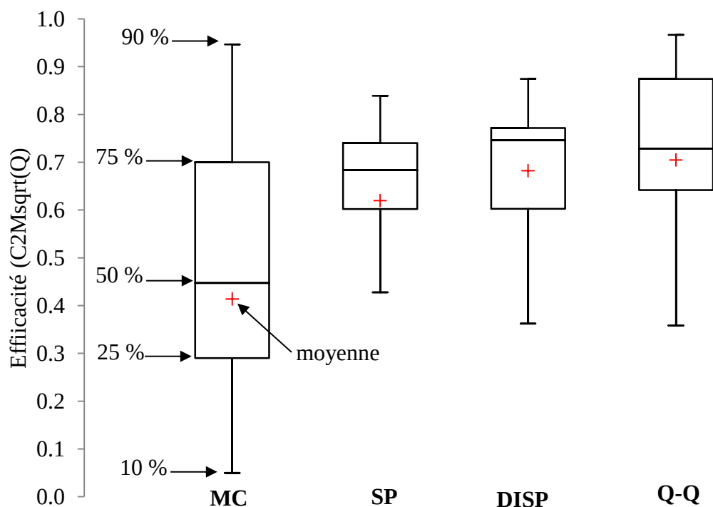
Figure 4.23. Distribution des valeurs du critère d'efficacité pour les quatre méthodes de régionalisation testées sur l'échantillon de 21 stations des RCS. MC : Carte de corrélation ; SP : proximité spatiale ; DISP : paramétrisation discrète ; QQ : méthode débit-débit. In 3-Drogue et Plasse (à paraître).
