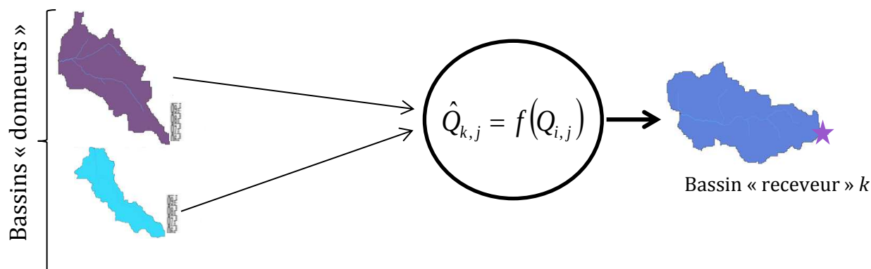
Figure 2.16. Principes de la régionalisation hydrologique par modélisation débit-débit (pas de temps journalier, deux donneurs). \hat{Q}_{k,j} représente le débit journalier ( j ) simulé à l'aide des i débits fournis par les bassins-receveurs.
