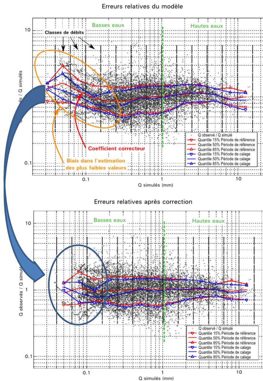
Figure 2.18. Correction et incertitudes des débits simulés (en mm/j) par le modèle pluie-débit GR4J. Exemple de la Meuse à Chalaines (1717 km 2 ), période 1973-2000. In 14-François et al. (2011).
