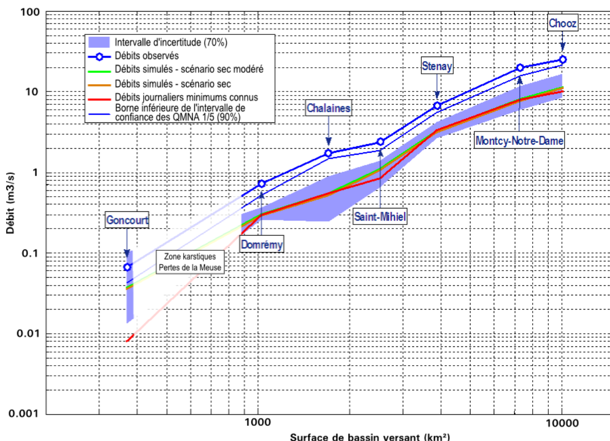
Figure 4.16. Profil hydrologique de la Meuse française. Débits mensuels d'étéage quinquennal sec (QMNA 5 ). Période de projection 2071-2100 vs. 1971-2000. In 14-François et al. (2011).
