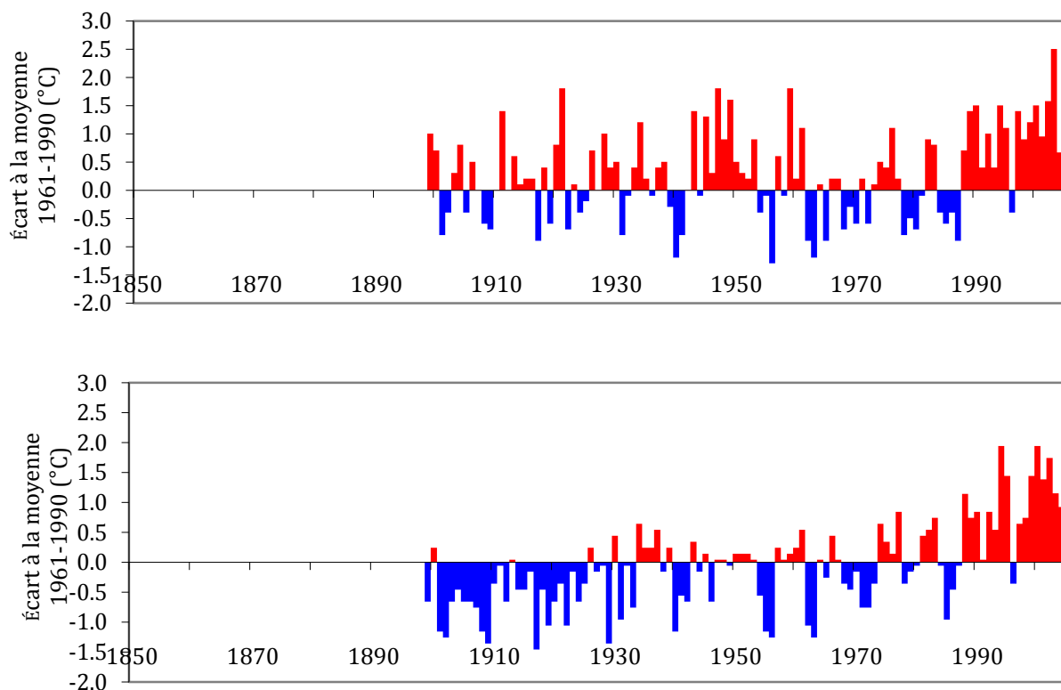
Figure 4.3. Ecarts annuels de la température maximale de l'air sous abri Tx (en haut) et de la température minimale de l'air sous abri Tn (en bas) par rapport à la moyenne 1961-1990 sur la période 1899-2007 à la station météorologique de Metz-Frescaty. Source des données : Météo-France.
