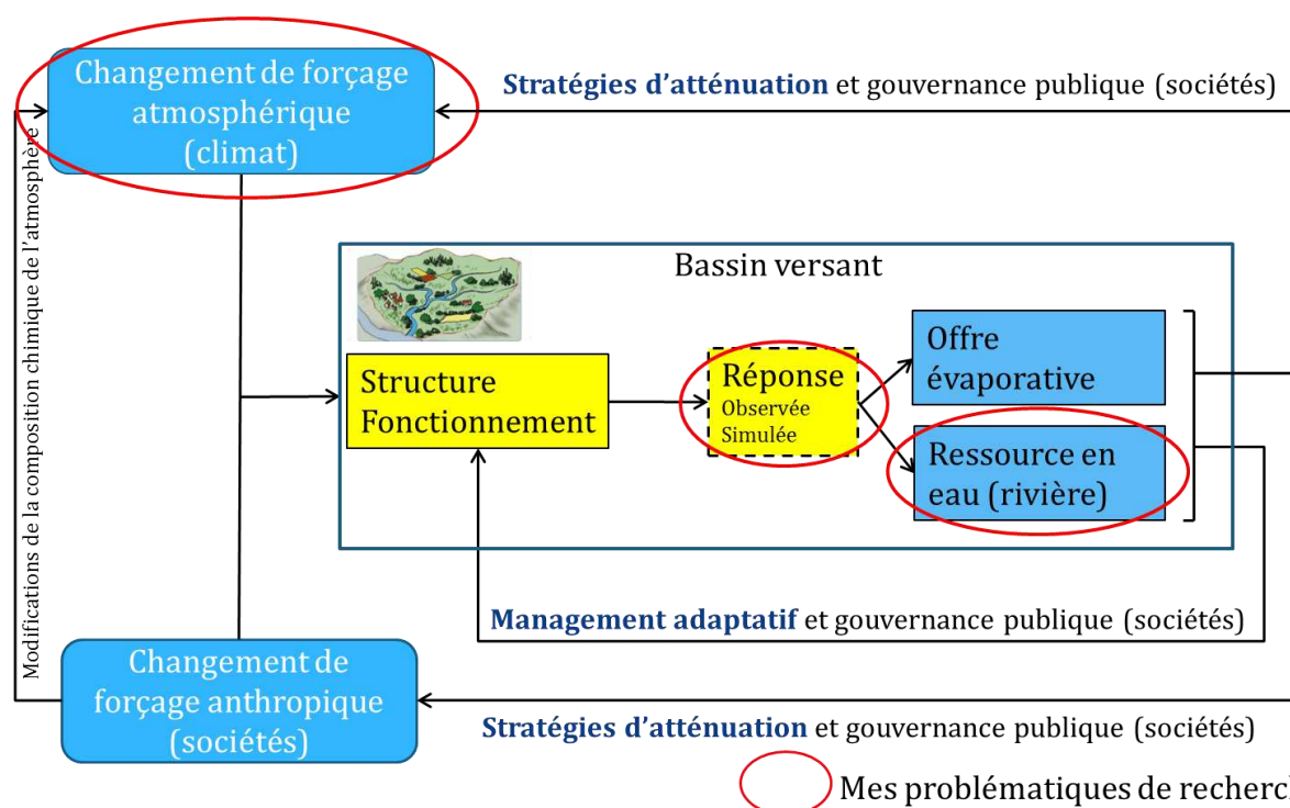
Figure 1.14 a. Contributions au champ de recherche portant sur l'hydrosystème appréhendé dans un contexte de changement global.
