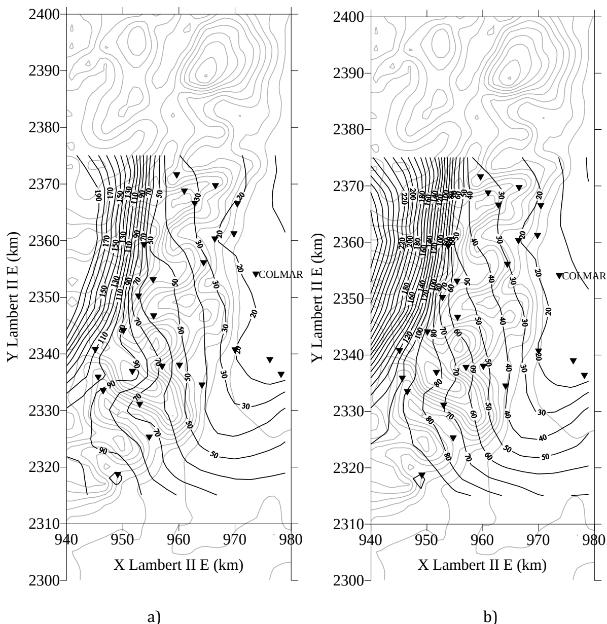
Figure 4.18. Isohyètes (en mm) afférentes à l'épisode pluvieux du 3 au 7 octobre 1988, secteur des Hautes-Vosges et leur piémont. Méthode du Krigeage à deux Dérives Externes (a) sans variance d'erreur de mesure (b) avec variance d'erreur de mesure. Voisinage d'interpolation unique, résidus structurés. Les isohypses sont représentées en gris. Résolution de la grille : 3 x 3 km. In 21-Drogue et al. (2010).
