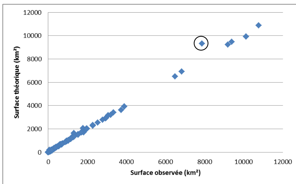
Figure 1.31. Comparaison entre surfaces observées et théoriques ( i.e. dérivées du plan de drainage HydroDem) dans la partie française du bassin Rhin-Meuse (350 bassins).
