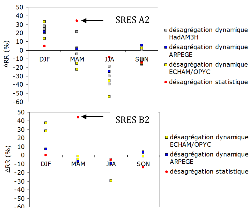
Figure 4.13. Taux de variation saisonniers de la pluie de bassin à l'échelle du bassin de la Sûre au Luxembourg. Scénarios PRUDENCE, période de projection 2071-2100. In 39-Droge et al. (2005).
