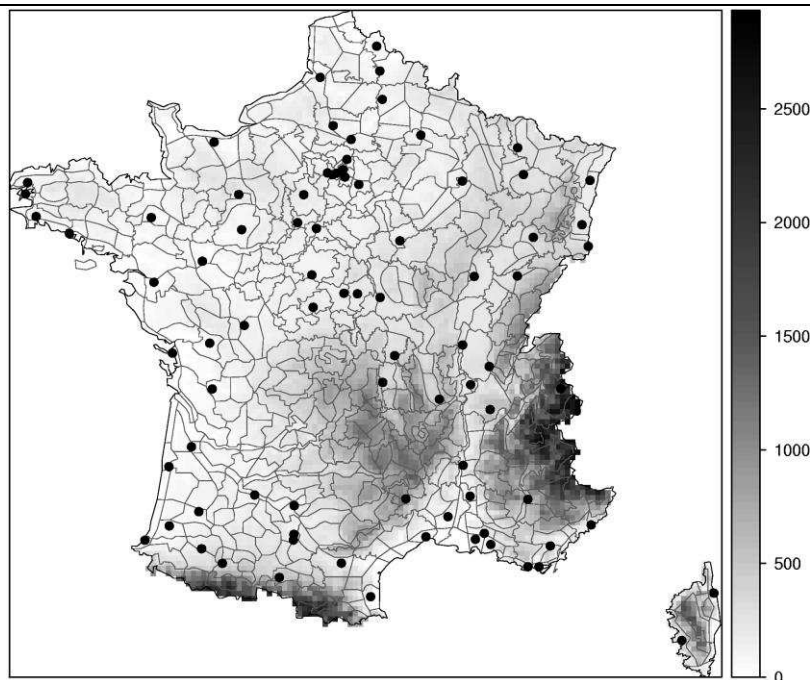
Figure 1.25. Zones climatiquement homogènes (615 zones sur France + Corse) et altitude des mailles. In Vidal (2011).
