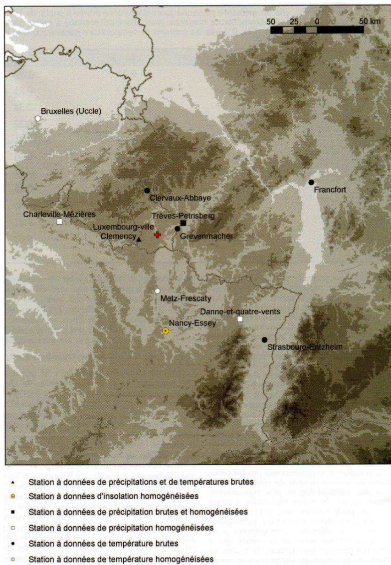
Figure 1.20. Réseau de stations de mesure historiques disponibles dans l'espace rhéno-mosan français de Bâle à Coblenze. In 16-Drogue et al. (2005).
