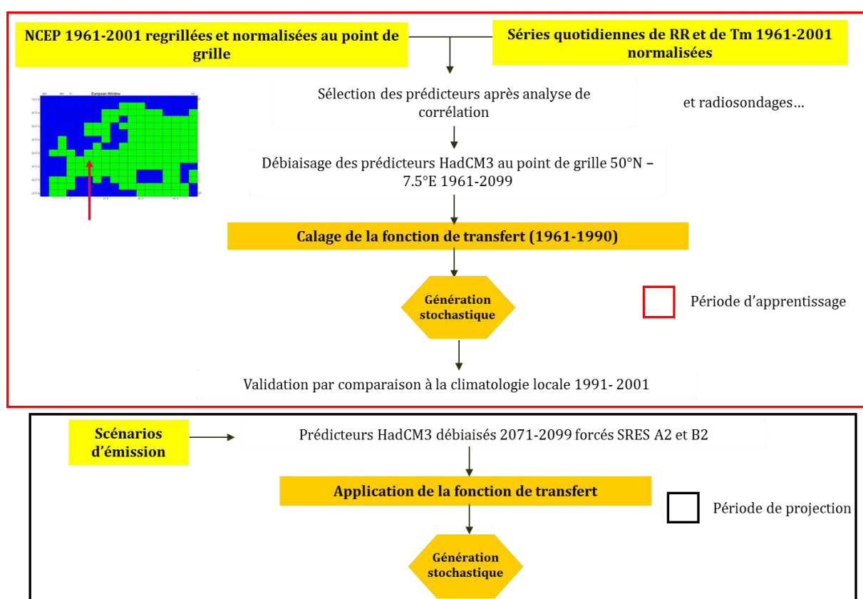
Figure 3.5.   tapes de la d  marche de descente d'  chelle statistique des sorties du MCG-OA HadCM3. RR : pr  cipitations, Tm : temp  rature moyenne de l'air. Adapt   de 39-Drogue et al. (2005).
