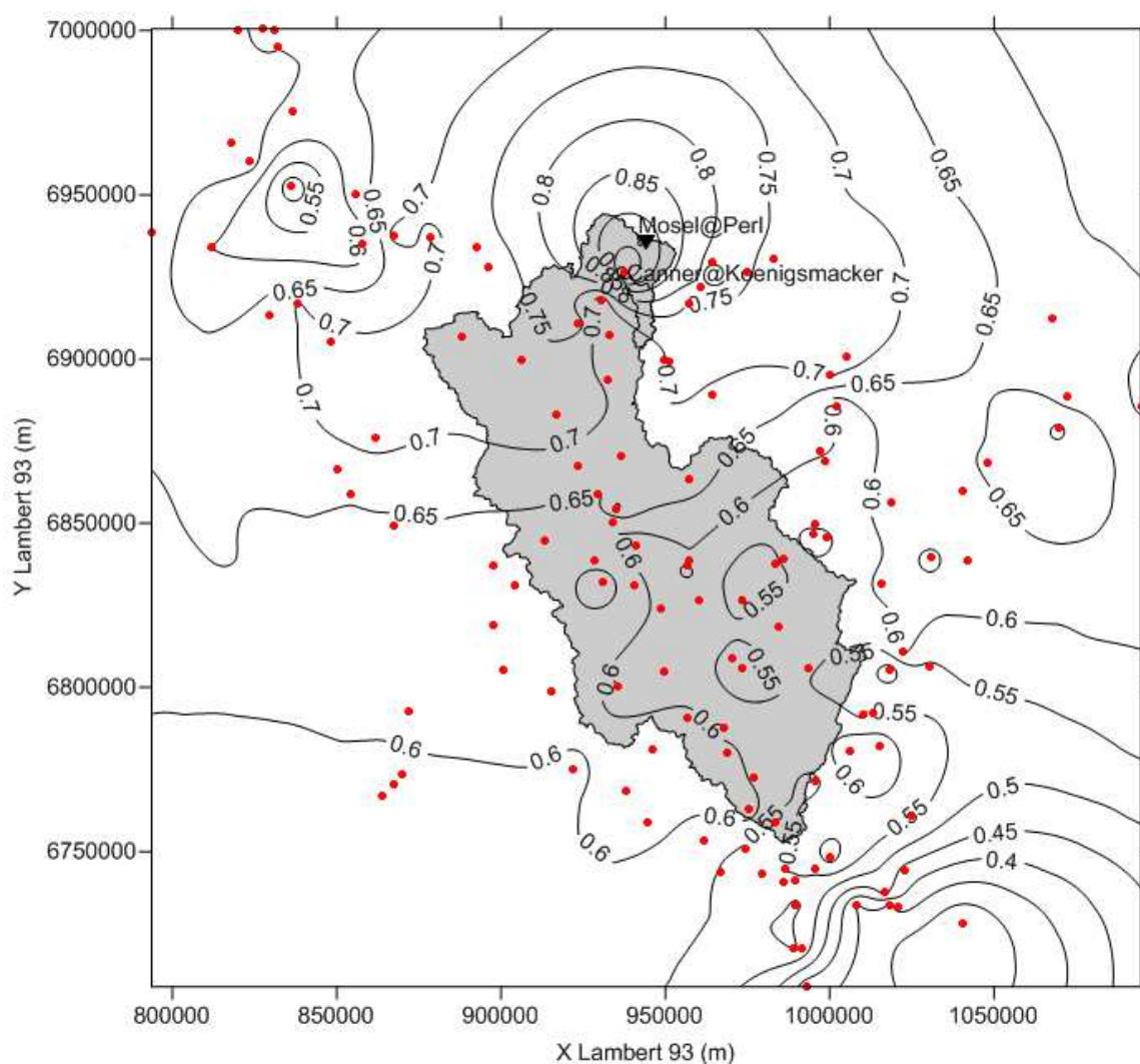
Figure 3.11. « Carte de corrélation » de la station hydrométrique de Koenigsmacker sur la Canner (affluent de rive droite de la Moselle). Distribution spatiale (krigeage ordinaire) du coefficient de corrélation de Bravais-Pearson entre les débits journaliers mesurés à cette station et les autres stations hydrométriques du réseau de mesure (149 au total) sur la période 1990-2009. Les contours des bassins de la Moselle à Perl et de la Canner à Koenigsmacker sont également représentés (voir commentaire). In 3-Drogue et Plasse (à paraître).
